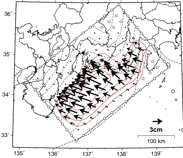
最近1年間のすべり欠損 ( 2009年7月 ~ 2010年7月 )
