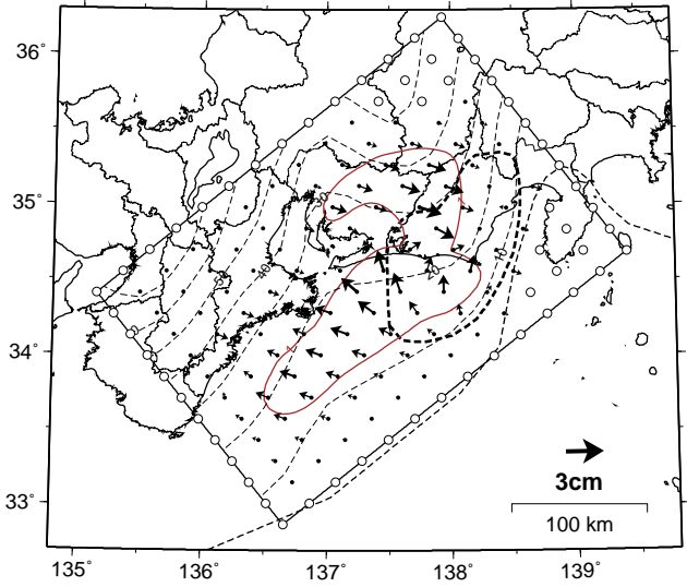
スロースリップ発生前との差 ( 2009年7月 ~ 2010年7月 )
