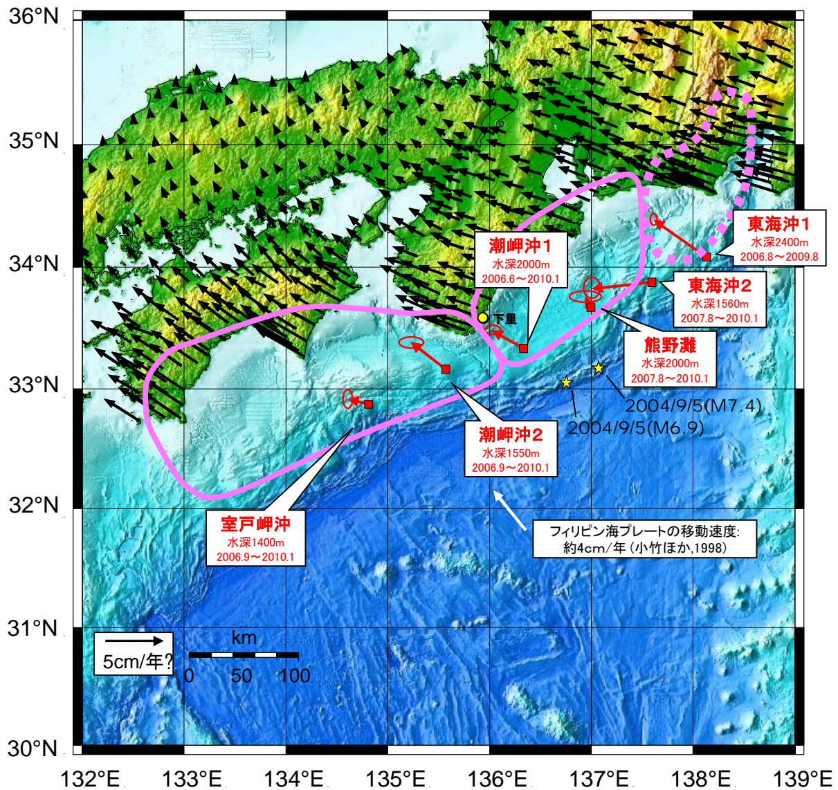
図1 ユーラシアプレート安定域に対する速度ベクトル
