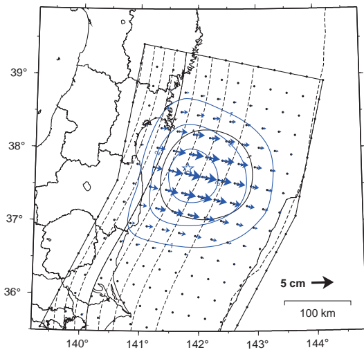
【2010 年 3 月 14 日福島県沖の地震時と地震後の比較】
