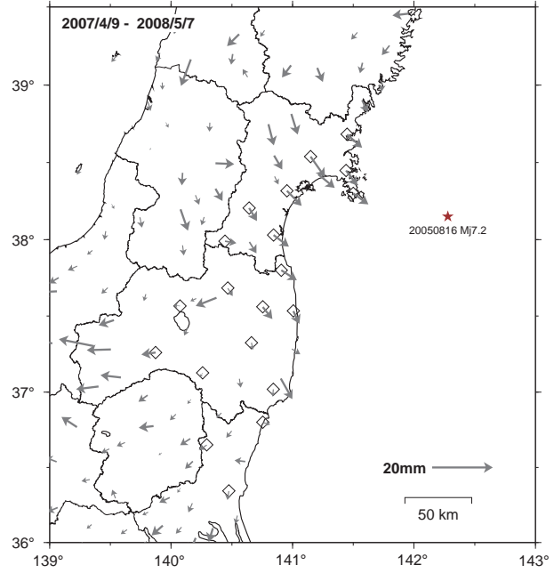
【2005年宮城県沖の地震発生以後2】
