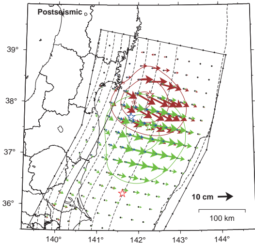
【地震後のすべりの比較】
