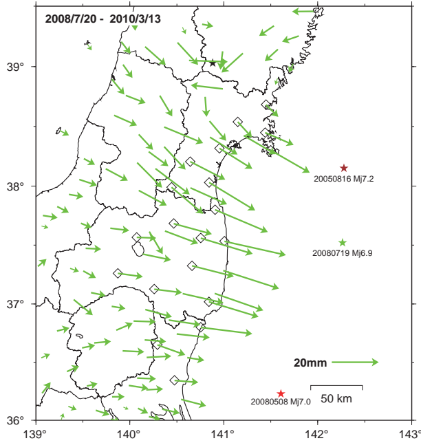
【2008年福島県沖の地震発生以後】
