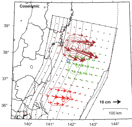
【地震時のすべりの比較】
