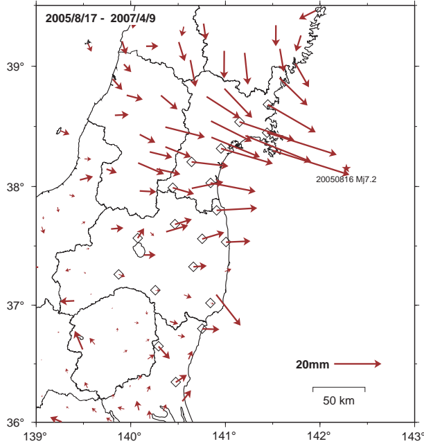
【2005年宮城県沖の地震発生以後】
