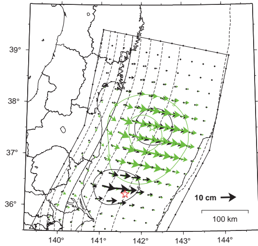
【2008 年 7 月 19 日福島県沖の地震時と地震後の比較】
