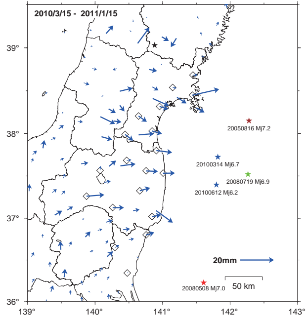
【2010年福島県沖の地震発生以後】
