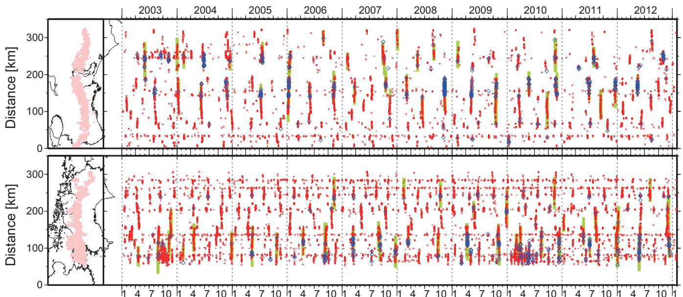
図3. 2003年1月～2013年1月までの深部低周波微動 (赤) および、深部超低周波地震 (青菱形) の時空間分布。緑太線は、傾斜変動から検出された短期的SSE。
