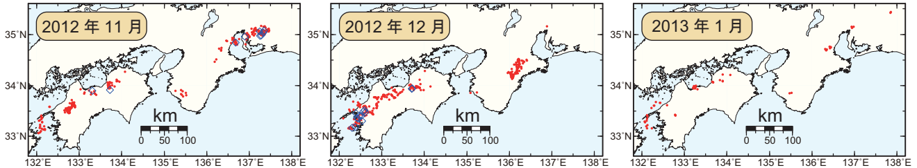
図1. 西南日本における2012年11月～2013年1月の月毎の深部低周波微動活動。赤丸はエンベロープ相関・振幅ハイブリッド法 (Maeda and Obara, 2009) およびクラスタ処理 (Obara et al., 2010) において、1時間毎に自動処理された微動分布の重心である。青菱形は周期20秒に卓越する深部超低周波地震 (Ito et al., 2007) である。
