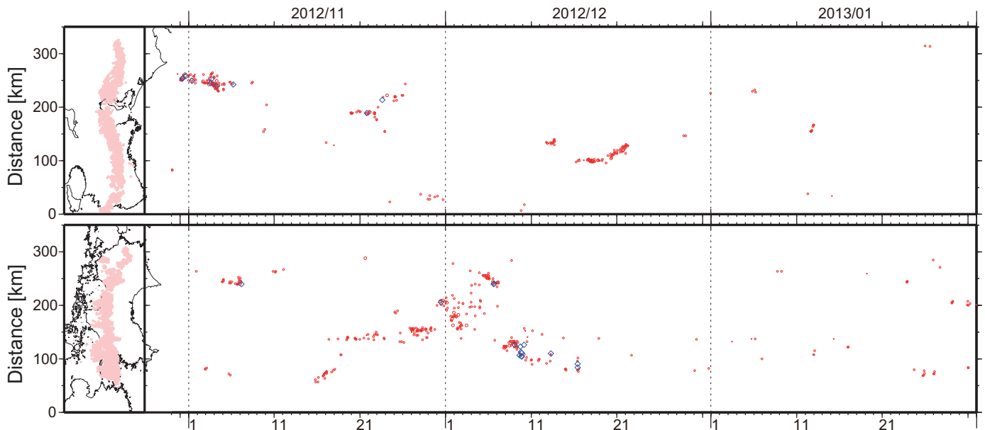
図2. 2012年10月30日～2013年1月の深部低周波微動 (赤) および、深部超低周波地震 (青菱形) の時空間分布。
