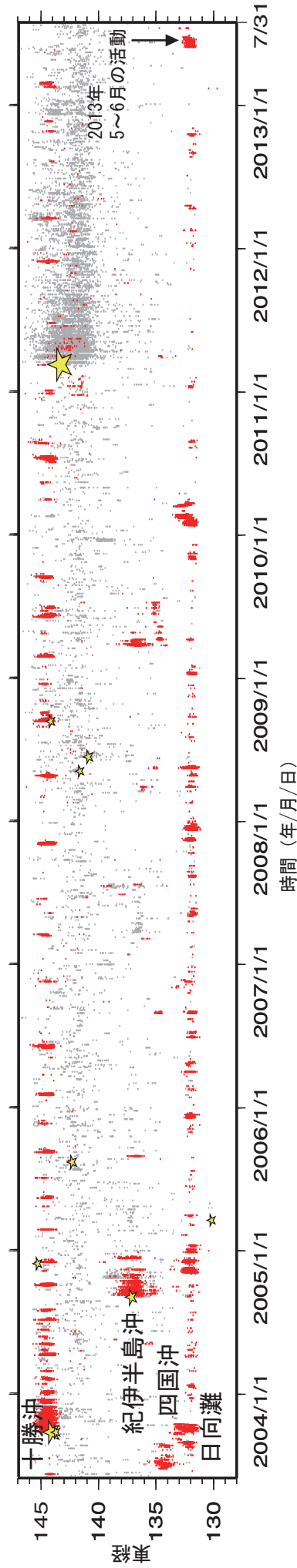
第3図. 2003年6月1日から2013年7月31日までの期間に検出されたイベントの時空間分布. 検出されたイベントを防災科研 Hi-net 手動, または自動検測震源と照合し, 対応する地震が見出されたイベントを灰色で, それ以外を赤色の点でそれぞれ示す. その他は第1図に同じ.
