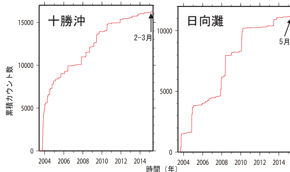
第2図. 十勝沖および日向灘周辺における検出イベントの累積カウント数の時間変化. 幅60秒間の解析時間窓を15秒毎に設定し，それぞれの解析時間窓内にイベントが検出される度に1カウントと数えるよう定義した.
