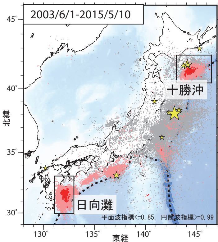
第1図. 2003年6月1日から2015年5月10日までの期間にアレイ解析によって検出されたイベントの震央分布. 検出イベントを防災科研 Hi-net の手動または自動検測震源と照合し，対応する地震が見出されたイベントを灰色で，それ以外を桃色（2014年10月31日以前），および赤色（11月1日以降）の点でそれぞれ示す. これらは主として周期10秒以上に卓越する超低周波地震を表すが，東北地方太平洋沖地震の発生以降は，除去しきれない通常の地震を多数含む. 期間内に発生したM7以上の地震の震央を黄色星印で併せて示す（ただし，2011年3月11日以降は東北地方太平洋沖地震の本震のみ）.
