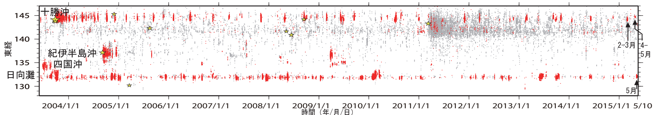
第3図. 2003年6月1日から2015年5月10日までの期間に検出されたイベントの時空間分布. 検出されたイベントを防災科研 Hi-net 手動または自動検測震源と照合し，対応する地震が見出されたイベントを灰色で，それ以外を赤色の点でそれぞれ示す. その他は第1図に同じ.
