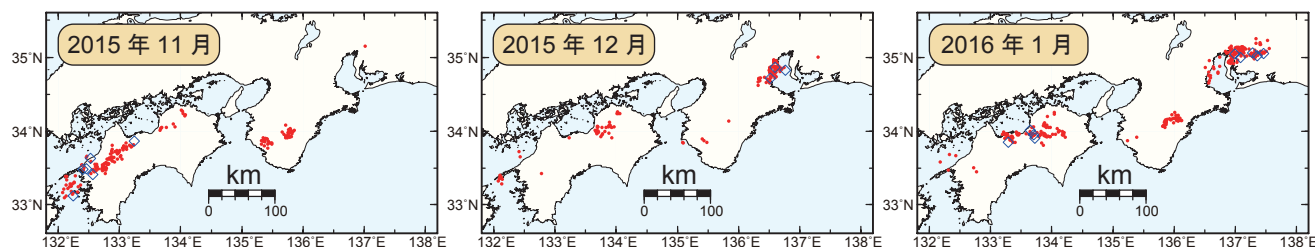
図 1. 西南日本における 2015 年 11 月～2016 年 1 月の月毎の深部低周波微動活動．赤丸はエンベロープ相関・振幅ハイブリッド法 (Maeda and Obara, 2009) およびクラスタ処理 (Obara et al., 2010) において，1 時間毎に自動処理された微動分布の重心である．青菱形は周期 20 秒に卓越する深部超低周波地震 (Ito et al., 2007) である．
