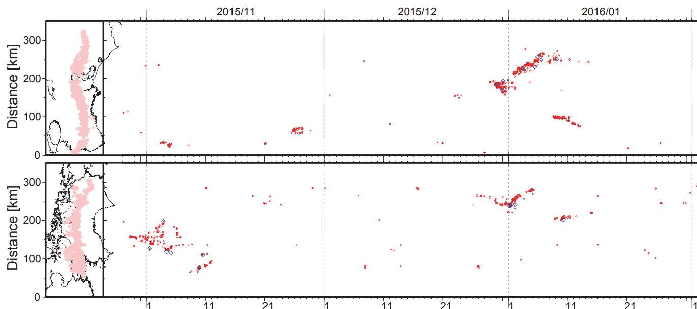
図 2. 2015 年 10 月 28 日～2016 年 2 月 1 日の深部低周波微動（赤）および，深部超低周波地震（青菱形）の時空間分布．
