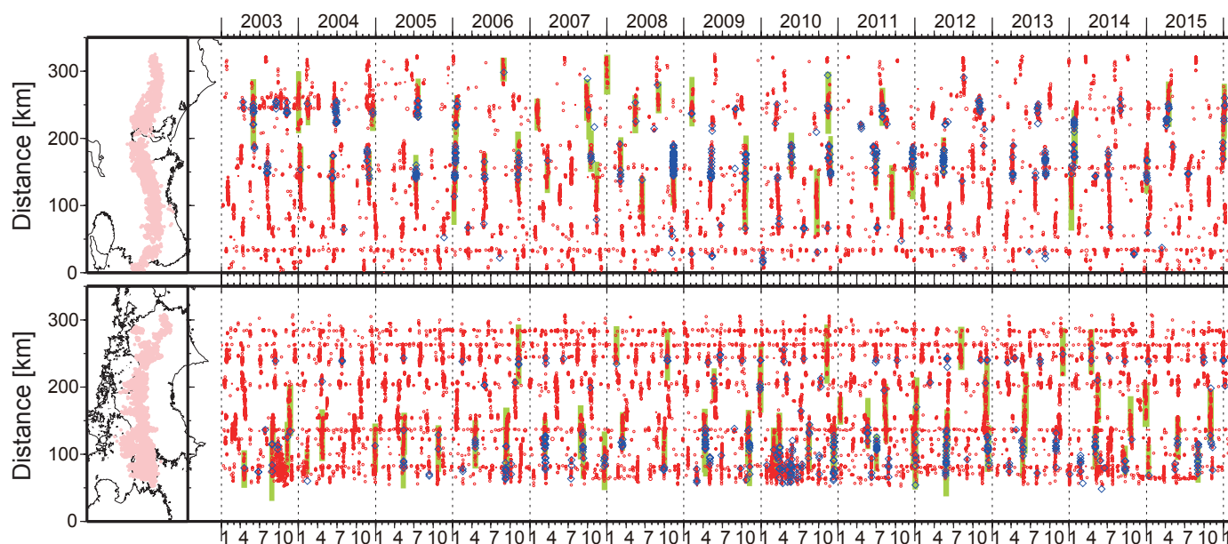
図 3. 2003 年 1 月～2016 年 2 月 1 日までの深部低周波微動（赤）および，深部超低周波地震（青菱形）の時空間分布．緑太線は，傾斜変動から検出された短期的スロースリップイベント．
