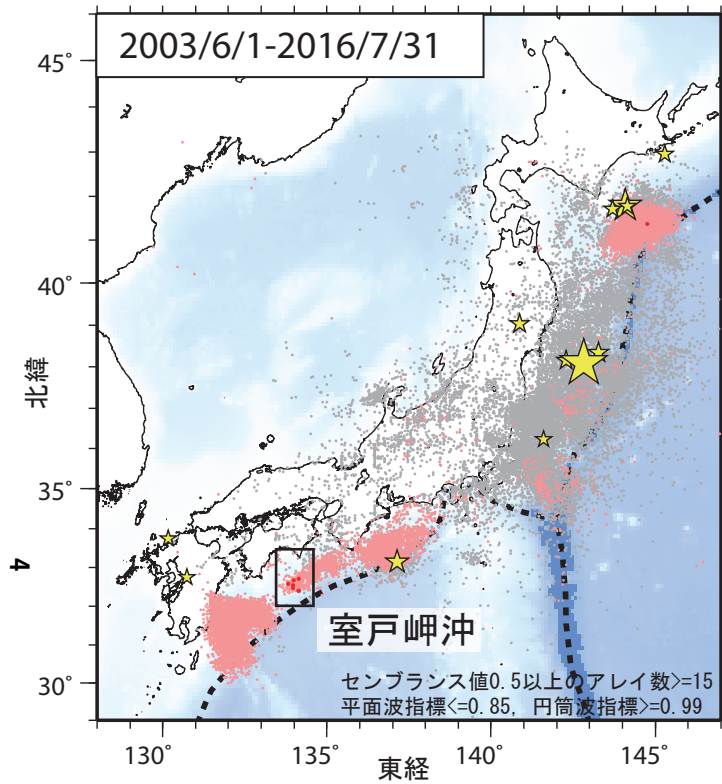
第1図. 2003年6月1日から2016年7月31日までの期間にアレイ解析によって検出されたイベントの震央分布. 検出イベントを防災科研 Hi-net の手動または自動検測震源と照合し, 対応する地震が見出されたイベントを灰色で, それ以外を桃色 (2016年4月30日以前), および赤色 (5月1日以降) の点でそれぞれ示す. これらは主として周期10秒以上に卓越する超低周波地震を表すが, 東北地方太平洋沖地震の発生以降は, 除去しきれない通常の地震を含む. 期間内に発生した M7 以上の地震 (ただし, 2011年～2015年の期間は東北地方太平洋沖地震の本震のみ) の震央を黄色星印で示す.
