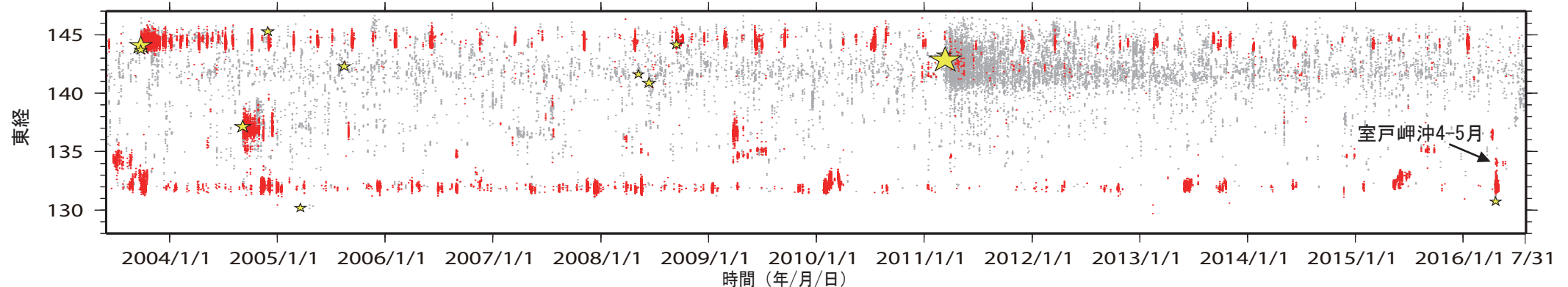
第3図. 2003年6月1日から2016年7月31日までの期間に検出されたイベントの時空間分布. 検出されたイベントを防災科研 Hi-net 手動または自動検測震源と照合し, 対応する地震が見出されたイベントを灰色で, それ以外を赤色の点でそれぞれ示す. その他は第1図に同じ.
