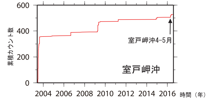
第2図. 室戸岬沖における検出イベントの累積カウンタ数の時間変化. 幅60秒間の解析時間窓を15秒毎に設定し, それぞれの解析時間窓内にイベントが検出される度に1カウントと数えるよう定義した.
