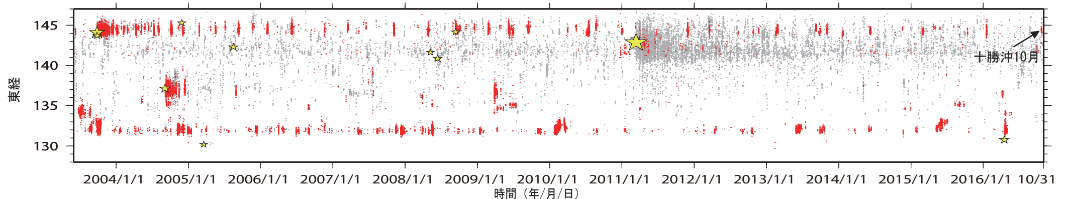
第3図. 2003年6月1日から2016年10月31日までの期間に検出されたイベントの時空間分布. 検出されたイベントを防災科研 Hi-net 手動または自動検測震源と照合し, 対応する地震が見出されたイベントを灰色で, それ以外を赤色の点でそれぞれ示す. その他は第1図に同じ.
