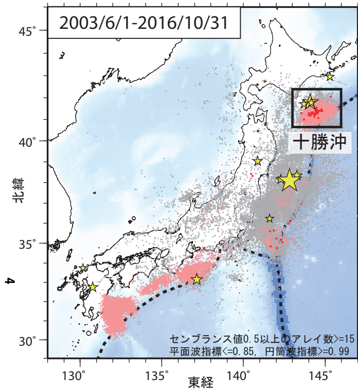
第1図. 2003年6月1日から2016年10月31日までの期間にアレイ解析によって検出されたイベントの震央分布. 検出イベントを防災科研 Hi-net の手動または自動検測震源と照合し, 対応する地震が見出されたイベントを灰色で, それ以外を桃色 (2016年4月30日以前), および赤色 (8月1日以降) の点でそれぞれ示す. これらは主として周期10秒以上に卓越する超低周波地震を表すが, 東北地方太平洋沖地震の発生以降は, 除去しきれない通常の地震を含む. 期間内に発生した M7 以上の地震 (ただし, 2011年～2015年の期間は東北地方太平洋沖地震の本震のみ) の震央を黄色星印で示す.
