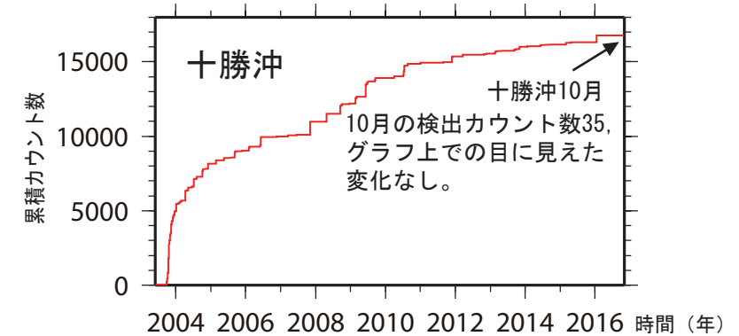
第2図. 十勝沖における検出イベントの累積カウンタ数の時間変化. 幅60秒間の解析時間窓を15秒毎に設定し, それぞれの解析時間窓内にイベントが検出される度に1カウントと数えるよう定義した.
