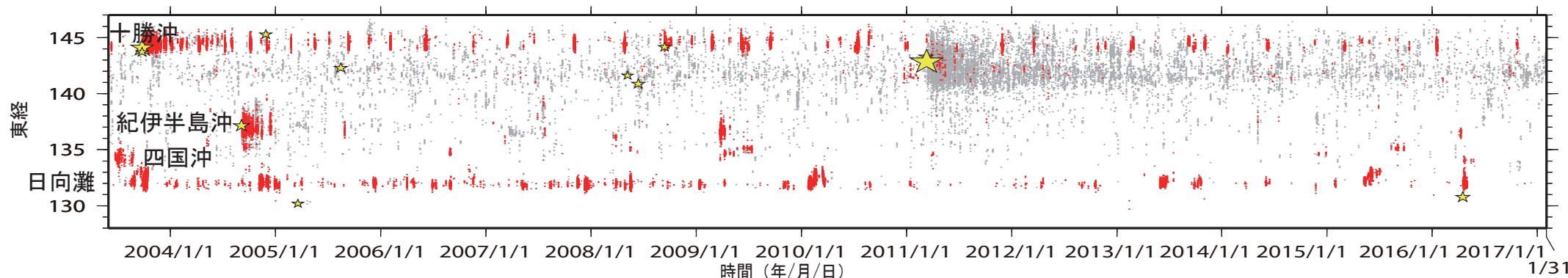
第2図. 2003年6月1日から2017年1月31日までの期間に検出されたイベントの時空間分布. 検出されたイベントを防災科研 Hi-net 手動, または自動検測震源と照合し, 対応する地震が見出されたイベントを灰色で, それ以外を赤色の点でそれぞれ示す. その他は第1図に同じ.
