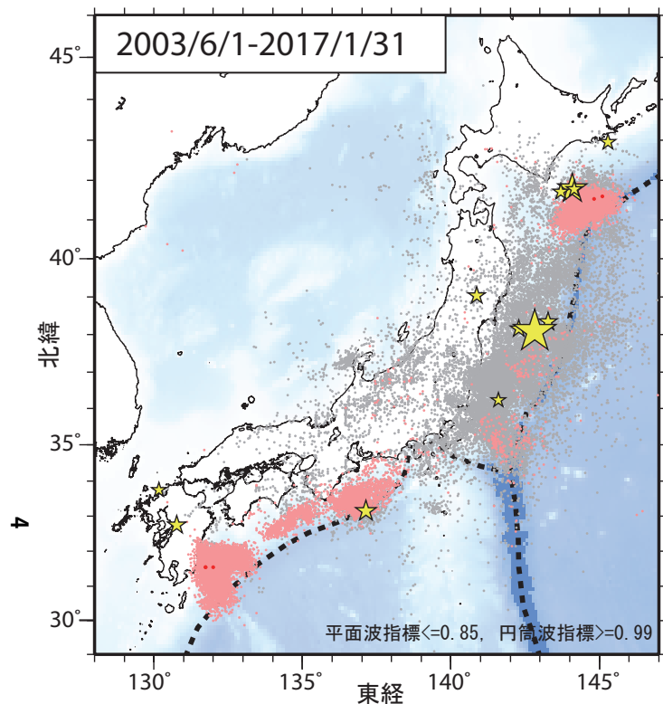
第1図. 2003年6月1日から2017年1月31日までの期間にアレイ解析によって検出されたイベントの震央分布. 検出イベントを防災科研 Hi-net の手動, または自動検測震源と照合し, 対応する地震が見出されたイベントを灰色で, それ以外を桃色 (2016年10月31日以前), および赤色 (11月1日以降) の点でそれぞれ示す. これらは主として周期10秒以上に卓越する超低周波地震を表すが, 東北地方太平洋沖地震の発生以降は, 除去しきれない通常の地震を多数含む. 期間内に発生したM7以上の地震の震央を黄色星印で併せて示す (ただし, 2011年3月11日～2015年は東北地方太平洋沖地震の本震のみ).
