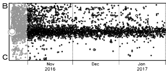
領域 a 内の時空間分布図 (B - C 投影)
