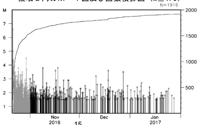
領域 a 内の M - T 図及び回数積算図 (M \geq 1.5)
