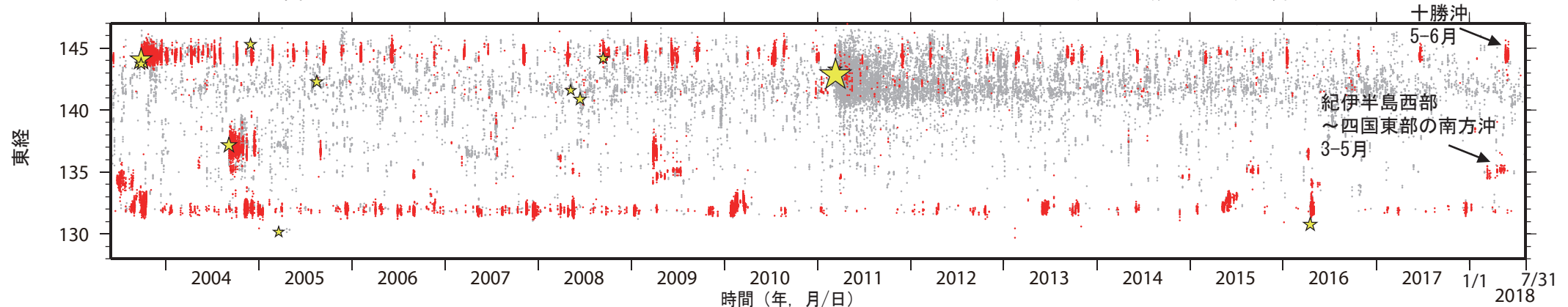
第3図. 2003年6月1日から2018年7月31日までの期間に検出されたイベントの時空間分布. 検出されたイベントを防災科研 Hi-net 手動または自動検測震源と照合し, 対応する地震が見出されたイベントを灰色で, それ以外を赤色の点でそれぞれ示す. その他は第1図に同じ.
