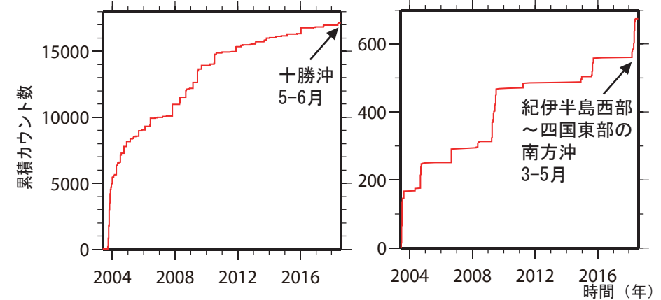
第2図. (左) 十勝沖, (右) 紀伊半島西部～四国東部の南方沖における検出イベントの累積カウンタ数の時間変化. 幅60秒間の解析時間窓を15秒毎に設定し, それぞれの解析時間窓内にイベントが検出される度に1カウントと数えるよう定義した.
