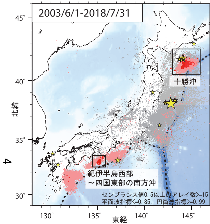
第1図. 2003年6月1日から2018年7月31日までの期間にアレイ解析によって検出されたイベントの震央分布. 検出イベントを防災科研 Hi-net の手動または自動検測震源と照合し, 対応する地震が見出されたイベントを灰色で, それ以外を桃色 (2018年4月30日以前), および赤色 (5月1日以降) の点でそれぞれ示す. これらは主として周期10秒以上に卓越する超低周波地震を表すが, 東北地方太平洋沖地震の発生以降は, 除去しきれない通常の地震を含む. 期間内に発生した M7 以上の地震 (ただし, 2011年～2015年の期間は東北地方太平洋沖地震の本震のみ) の震央を黄色星印で示す.
