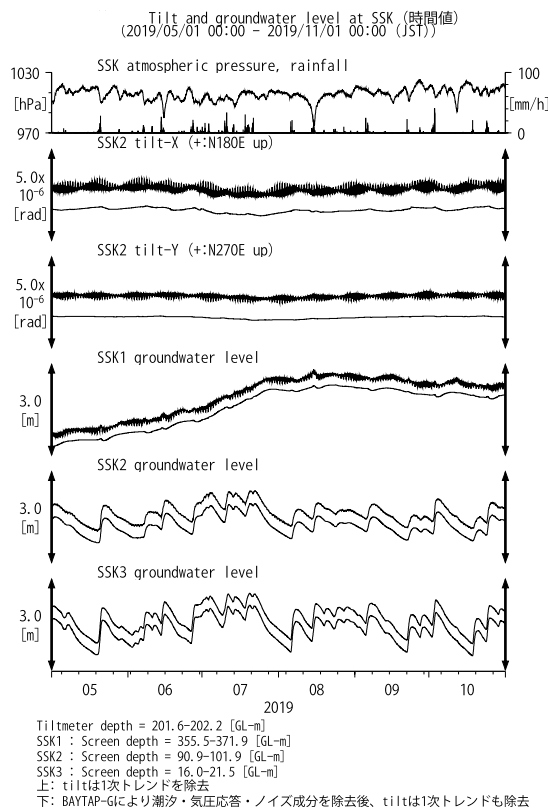
第28図 SSKにおける傾斜・地下水位観測結果(2019年5月～2019年10月)
