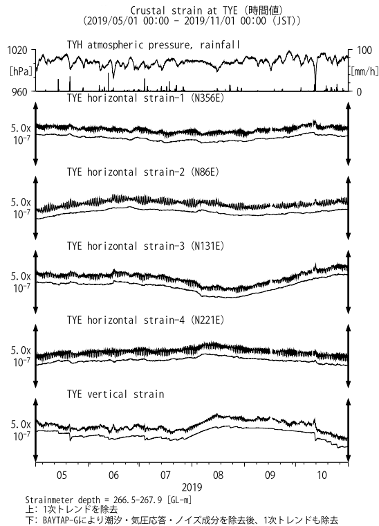
第6図 TYEにおける歪観測結果(2019年5月～2019年10月) Fig. 6 Observed strains at the TYE observation site from May 2019 to October 2019.
