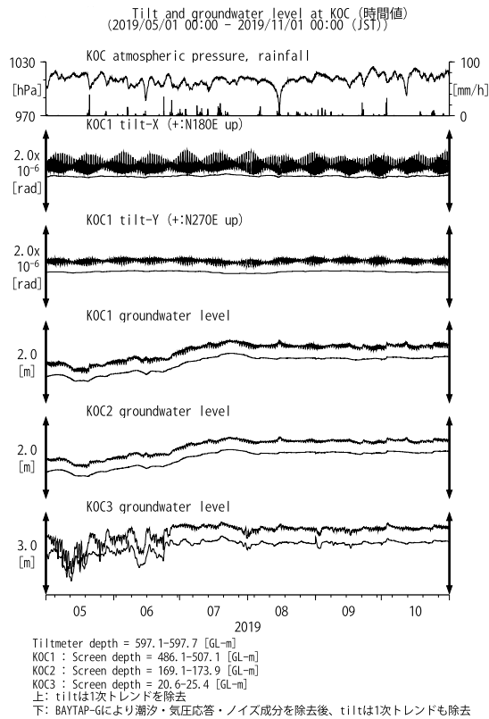
第26図 KOCにおける傾斜・地下水位観測結果(2019年5月～2019年10月)
