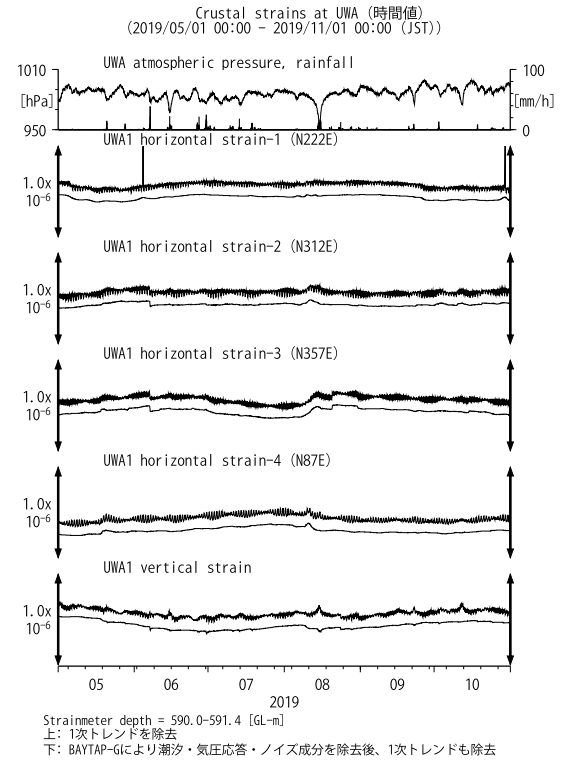
第31図 UWAにおける歪観測結果(2019年5月～2019年10月)
