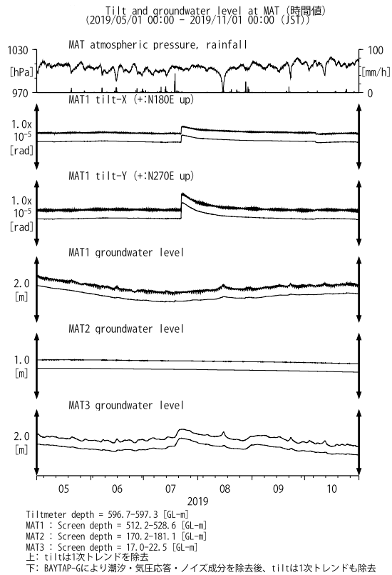
第 34 図 MAT における傾斜・地下水位観測結果 (2019 年 5 月～2019 年 10 月)
