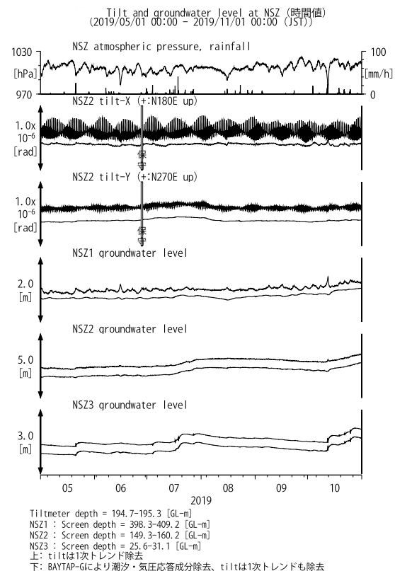
第5図 NSZにおける傾斜・地下水位観測結果(2019年5月～2019年10月) Fig. 5 Observed tilts and groundwater levels at the NSZ observation site from May 2019 to October 2019.
