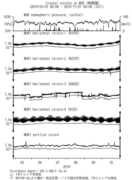
第23図 MURにおける歪観測結果(2019年5月～2019年10月)
