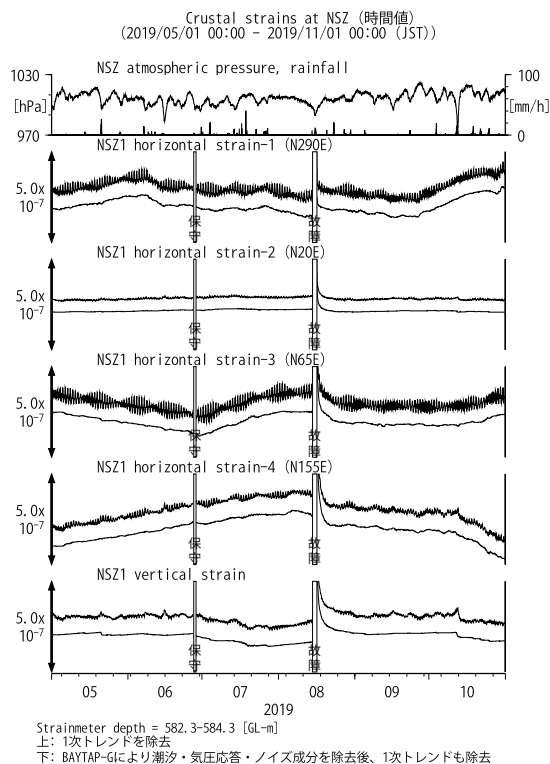
第4図 NSZにおける歪観測結果(2019年5月～2019年10月) Fig. 4 Observed strains at the NSZ observation site from May 2019 to October 2019.
