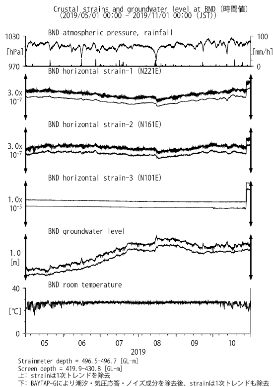
第 20 図 BND における歪・地下水位観測結果 (2019 年 5 月～2019 年 10 月) Fig. 20 Observed strains and groundwater level at the BND observation site from May 2019 to October 2019.
