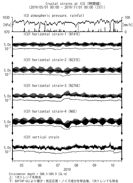
第 14 図 ICU における歪観測結果 (2019 年 5 月～2019 年 10 月) Fig. 14 Observed strains at the ICU observation site from May 2019 to October 2019.
