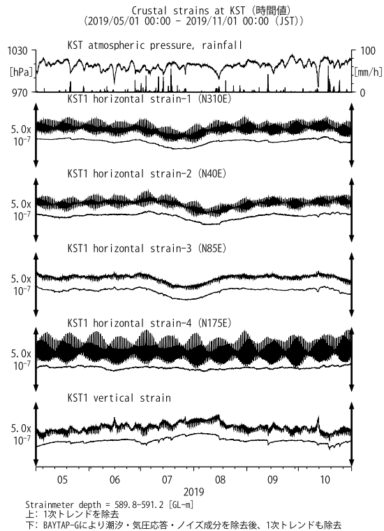
第 18 図 KST における歪観測結果 (2019 年 5 月～2019 年 10 月) Fig. 18 Observed strains at the KST observation site from May 2019 to October 2019.
