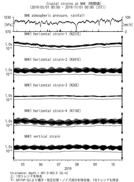
第 35 図 NHK における歪観測結果 (2019 年 5 月～2019 年 10 月)
