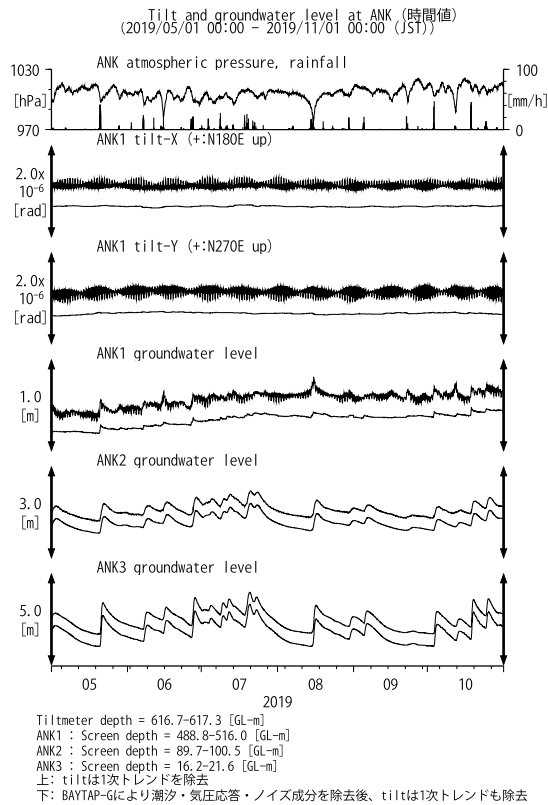
第22図 ANKにおける傾斜・地下水位観測結果(2019年5月～2019年10月)
