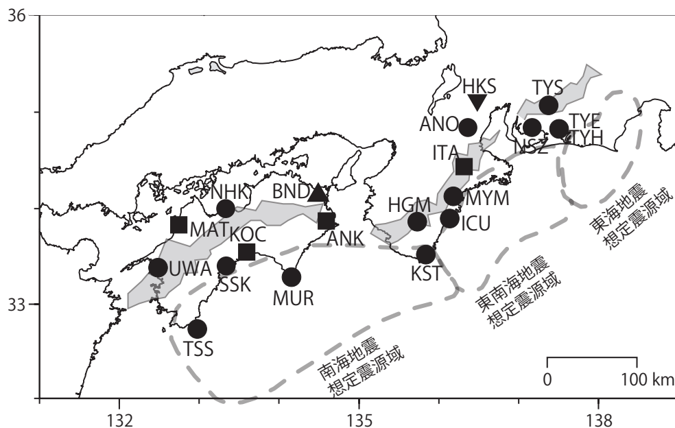
第1図 地下水等総合観測点の分布図 (●, ■, ▲, ▼). 観測点の一覧は第1表に示す. ●はデジタル方式の石井式歪計・傾斜計を併設している新規観測点, ■は Gladwin 式歪計・ミットヨ式傾斜計を併設している新規観測点, ▲はアナログ方式の石井式歪計を併設している既存の観測点, ▼は既存の地下水観測点. 灰色の領域は短期的 SSE 及び深部低周波微動が定常的に発生していると考えられる地域.
