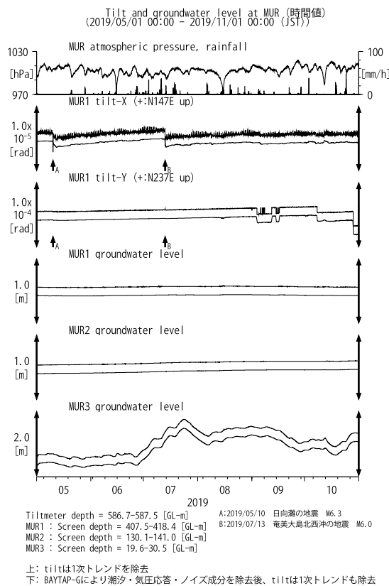
第24図 MURにおける傾斜・地下水位観測結果(2019年5月～2019年10月)
