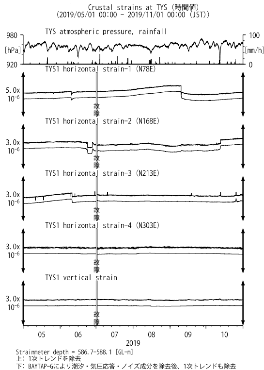
第2図 TYSにおける歪観測結果(2019年5月～2019年10月) Fig. 2 Observed strains at the TYS observation site from May 2019 to October 2019.
