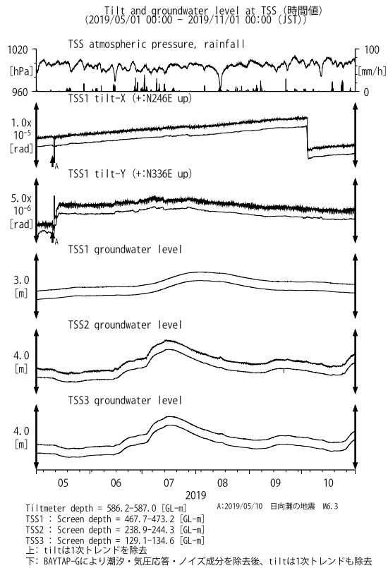
第30図 TSSにおける傾斜・地下水位観測結果(2019年5月～2019年10月)
