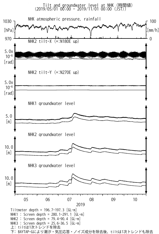
第 36 図 NHK における傾斜・地下水位観測結果 (2019 年 5 月～2019 年 10 月)
