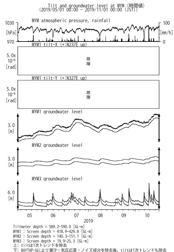
第13図 MYMにおける傾斜・地下水位観測結果(2019年5月～2019年10月) Fig. 13 Observed tilts and groundwater levels at the MYM observation site from May 2019 to October 2019.
