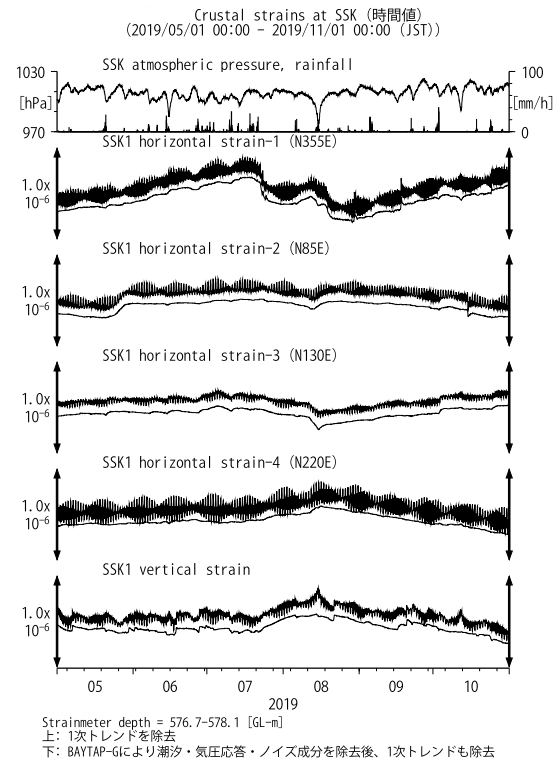
第27図 SSKにおける歪観測結果(2019年5月～2019年10月)
