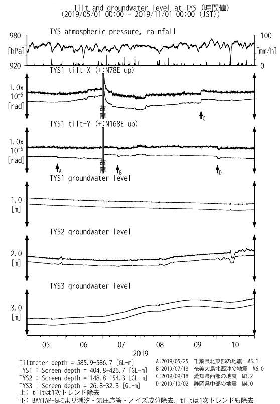
第3図 TYSにおける傾斜・地下水位観測結果(2019年5月～2019年10月) Fig. 3 Observed tilts and groundwater levels at the TYS observation site from May 2019 to October 2019.
