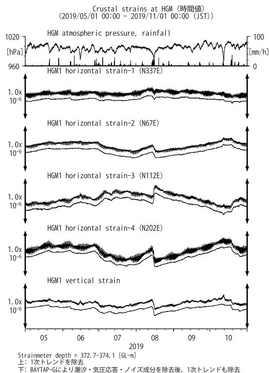
第 16 図 HGM における歪観測結果 (2019 年 5 月～2019 年 10 月) Fig. 16 Observed strains at the HGM observation site from May 2019 to October 2019.
