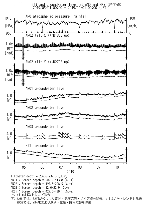
第9図 ANOおよびHKSにおける傾斜・地下水位観測結果(2019年5月～2019年10月) Fig. 9 Observed tilts and groundwater levels at the ANO and the HKS observation site from May 2019 to October 2019.
