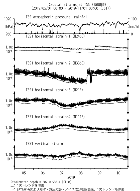
第29図 TSSにおける歪観測結果(2019年5月～2019年10月)
