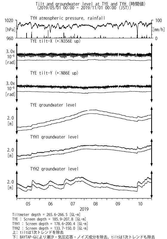
第7図 TYEおよびTYHにおける傾斜・地下水位観測結果(2019年5月～2019年10月) Fig. 7 Observed tilts and groundwater levels at the TYE and the TYH observation site from May 2019 to October 2019.
