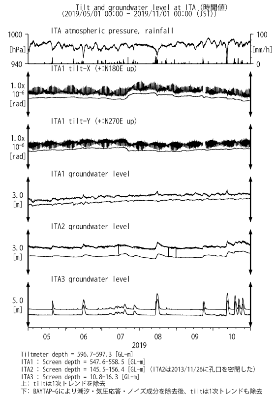
第11図 ITAにおける傾斜・地下水位観測結果(2019年5月～2019年10月) Fig. 11 Observed tilts and groundwater levels at the ITA observation site from May 2019 to October 2019.
