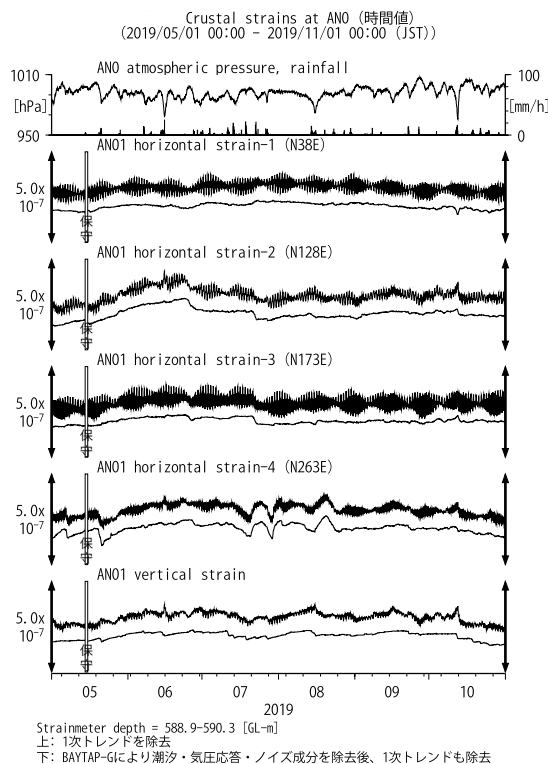
第8図 ANOにおける歪観測結果(2019年5月～2019年10月) Fig. 8 Observed strains at the ANO observation site from May 2019 to October 2019.
