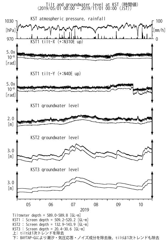
第 19 図 KST における傾斜・地下水位観測結果 (2019 年 5 月～2019 年 10 月) Fig. 19 Observed tilts and groundwater levels at the KST observation site from May 2019 to October 2019.
