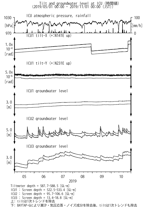
第 15 図 ICU における傾斜・地下水位観測結果 (2019 年 5 月～2019 年 10 月) Fig. 15 Observed tilts and groundwater levels at the ICU observation site from May 2019 to October 2019.
