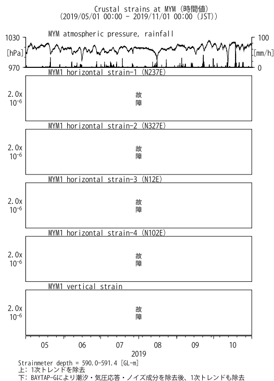
第12図 MYMにおける歪観測結果(2019年5月～2019年10月) Fig. 12 Observed strains at the MYM observation site from May 2019 to October 2019.
