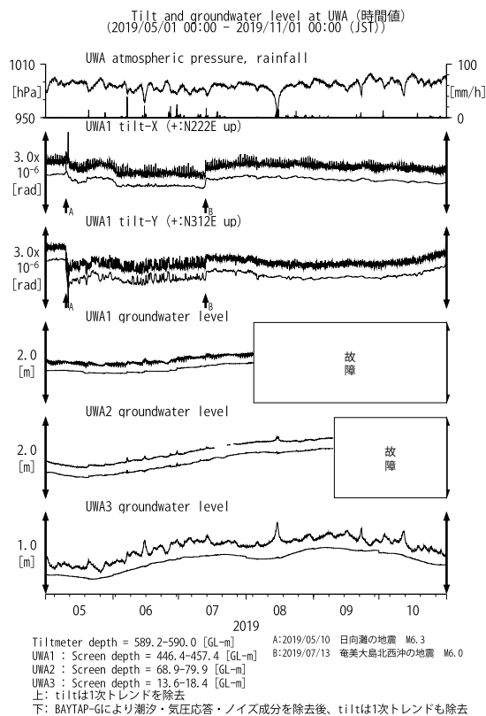
第32図 UWAにおける傾斜・地下水位観測結果(2019年5月～2019年10月)
