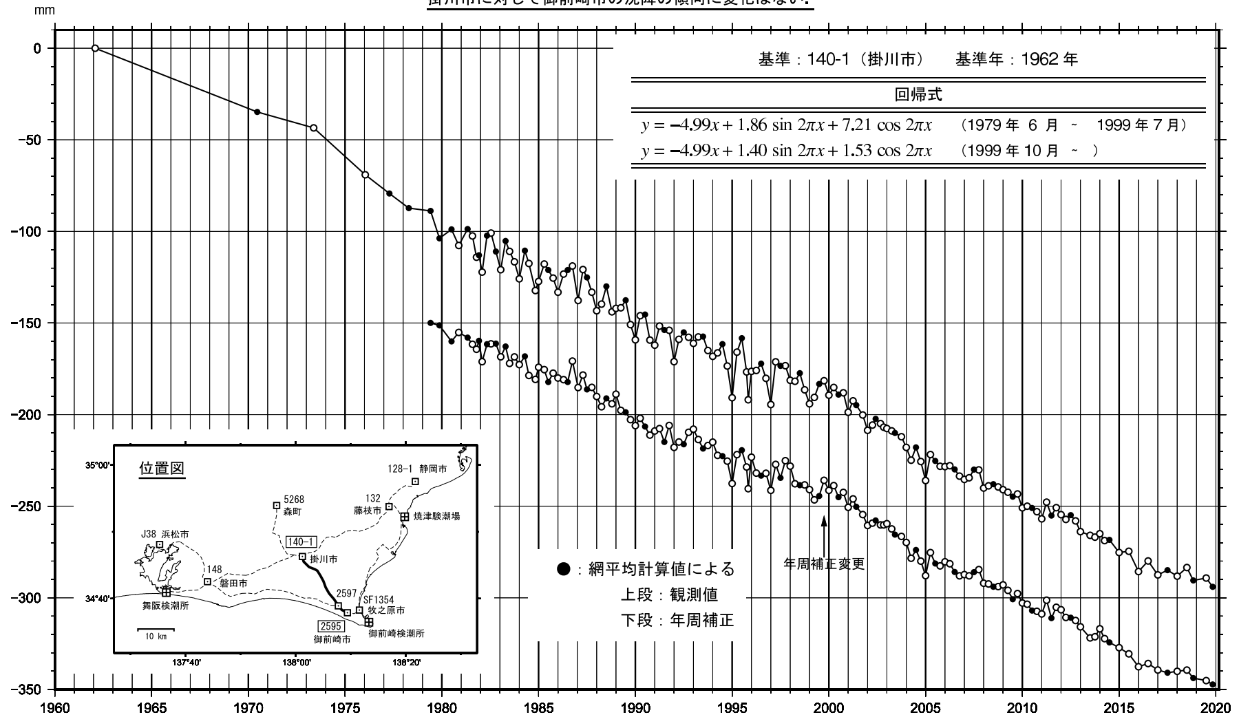
第 7 図 水準点 140-1（掛川市）を基準とした 2595（御前崎市浜岡）の高さの経年変化
