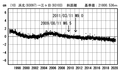
第 15 図 御前崎周辺 GNSS 連続観測点観測結果 (斜距離) (2)
