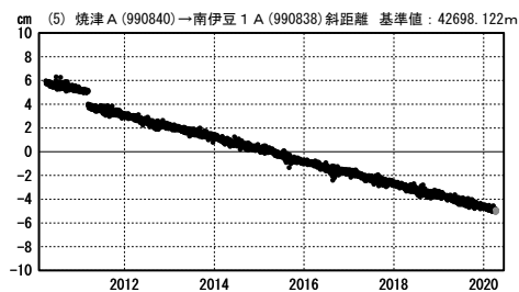
第 19 図 駿河湾周辺 GNSS 連続観測点観測結果 (斜距離) (1)
