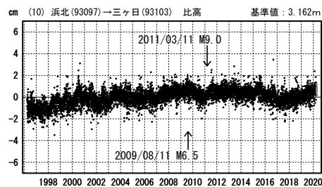
第 17 図 御前崎周辺 GNSS 連続観測点観測結果 (比高) (2)
