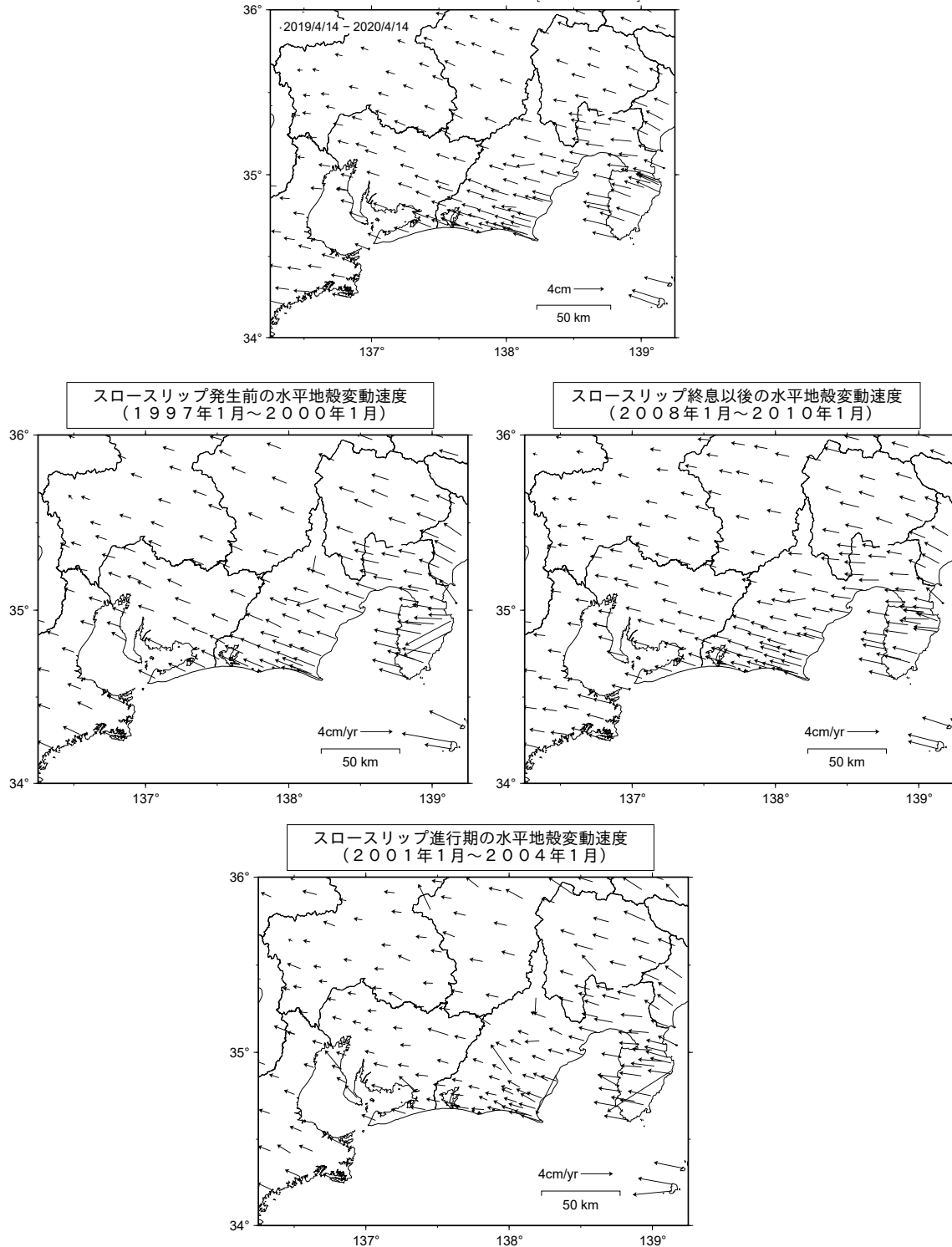
第 23 図 GNSS 観測による東海地方の最近 1 年間の水平変動及びスロースリップ開始前・進行期・終息後の水平変動速度（三隅固定）
