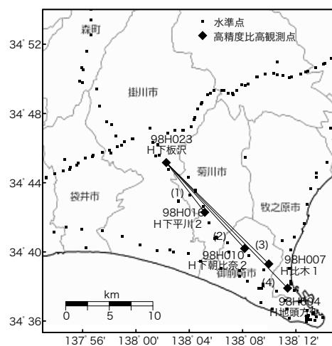
第 2 図 御前崎地域の高精度比高観測点の上下変動 (水準測量と GNSS)
