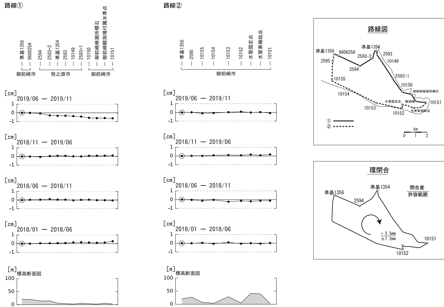
第 11 図 水準測量による御前崎先端部の上下変動 (1)
