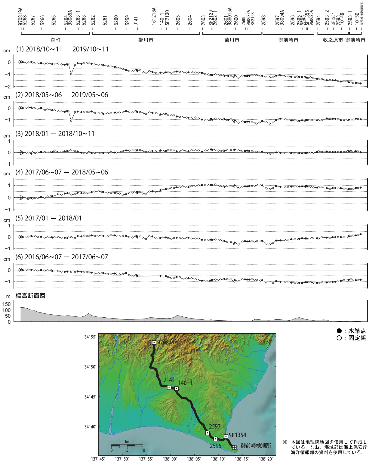
第 6 図 水準測量による森町～掛川市～御前崎市間における上下変動 Fig. 6 Vertical displacements from Mori town to Omaezaki city via Kakegawa city.
