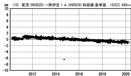
第 20 図 駿河湾周辺 GNSS 連続観測点観測結果 (斜距離) (2)
