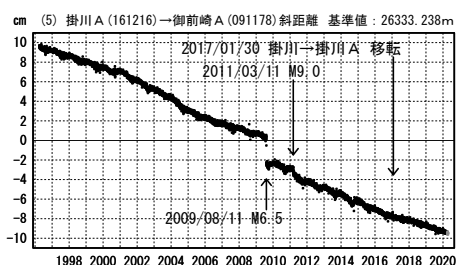
第 14 図 御前崎周辺 GNSS 連続観測点観測結果 (斜距離) (1)
