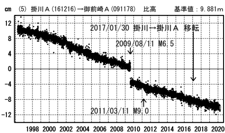
第 16 図 御前崎周辺 GNSS 連続観測点観測結果 (比高) (1)
