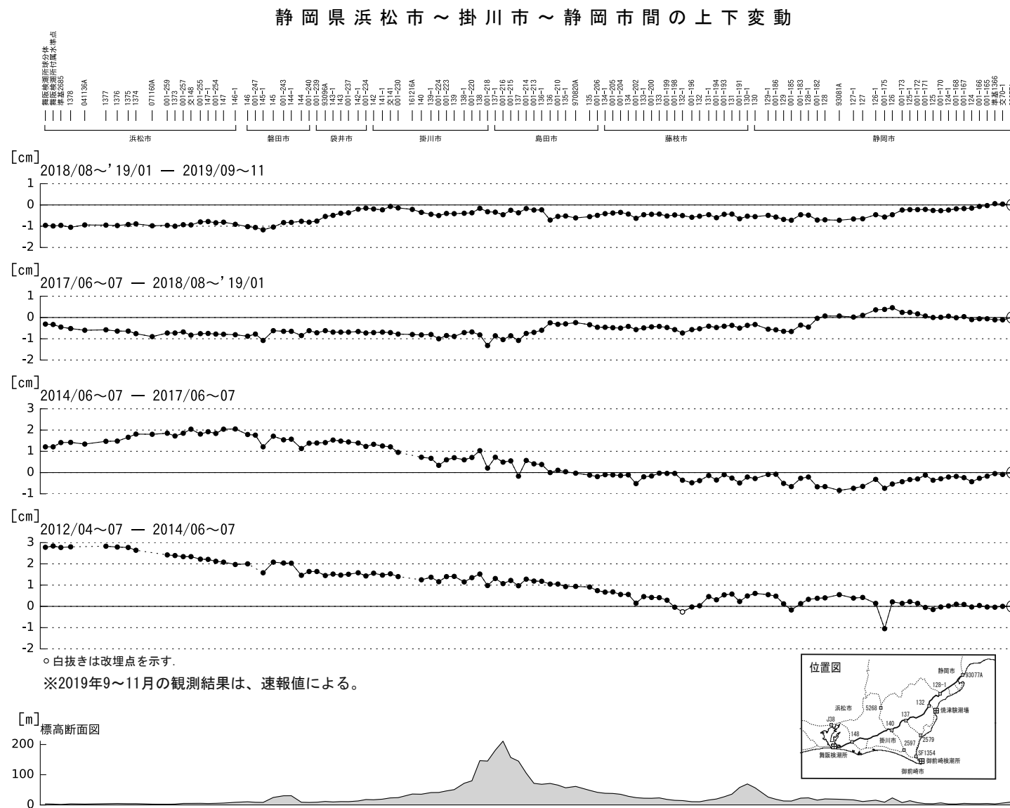
第 28 図 浜松～掛川～静岡間の上下変動
