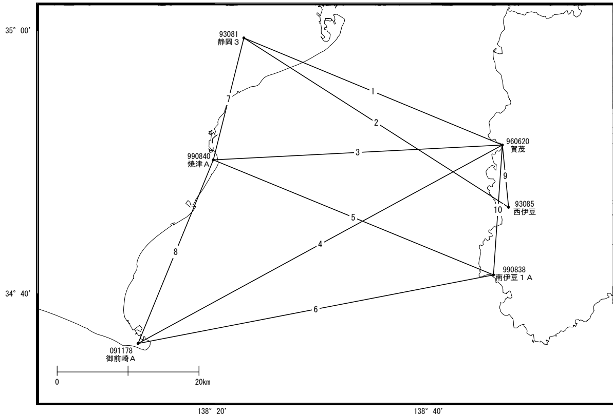
基線図
