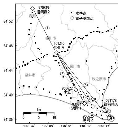
第 1 図 御前崎 電子基準点の上下変動 (水準測量と GNSS)
