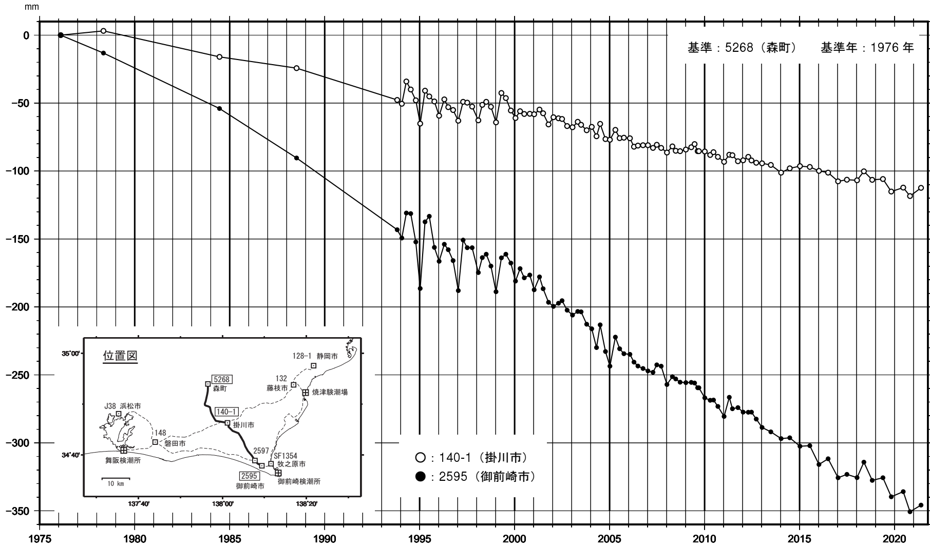
第9図 水準点 5268（森）を基準とした 140-1（掛川）と 2595（御前崎市）の上下変動時系列
