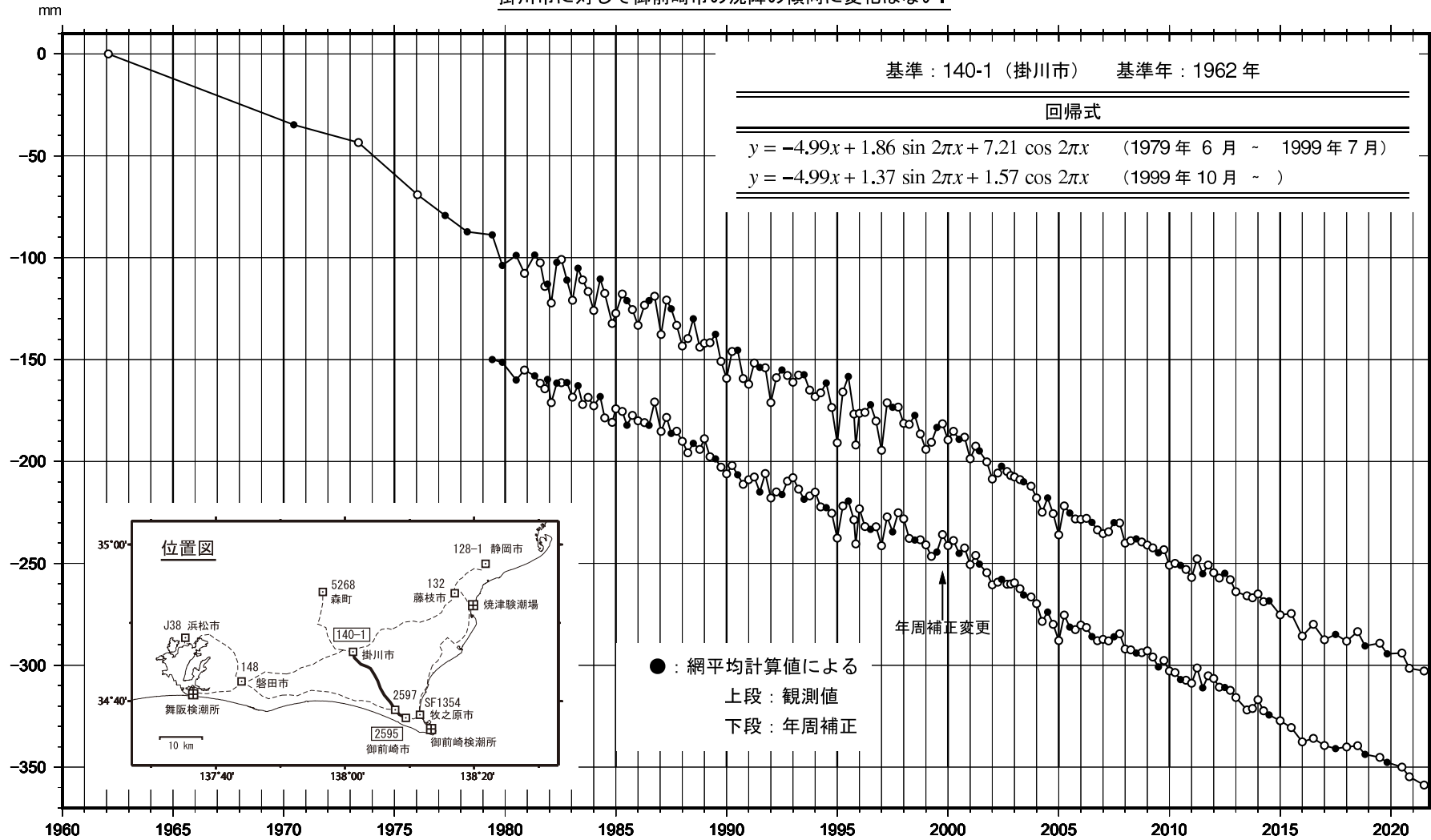
第 7 図 水準点 140-1（掛川市）を基準とした 2595（御前崎市）の高さの経年変化
