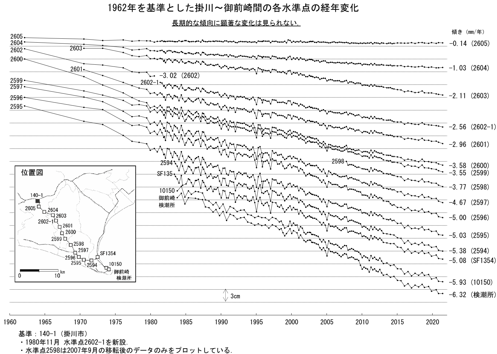
第 10 図 水準点 140-1 (掛川市) を基準とした掛川～御前崎間の各水準点の高さの経年変化
