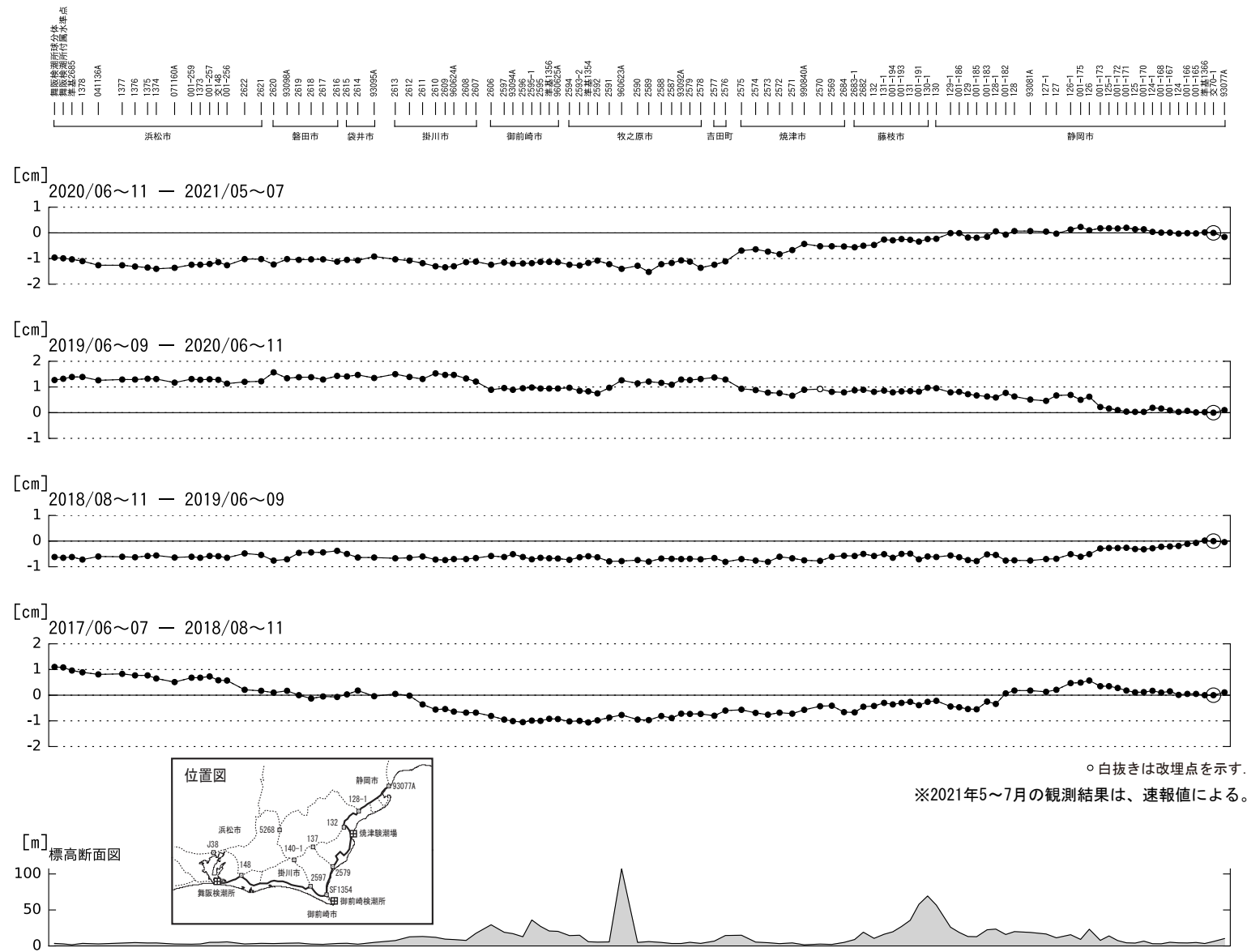
第 28 図 浜松市～御前崎市～静岡市間の上下変動
