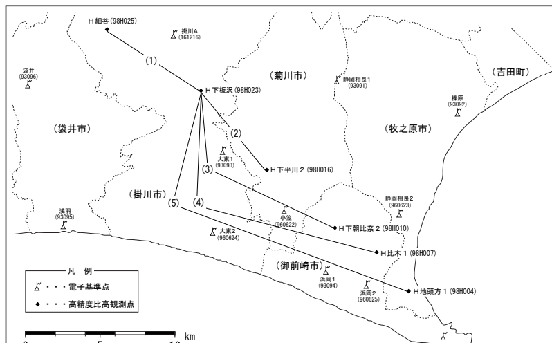
第 3 図 (a) 御前崎地域の高精度比高観測 GNSS 観測結果 (基線図)
