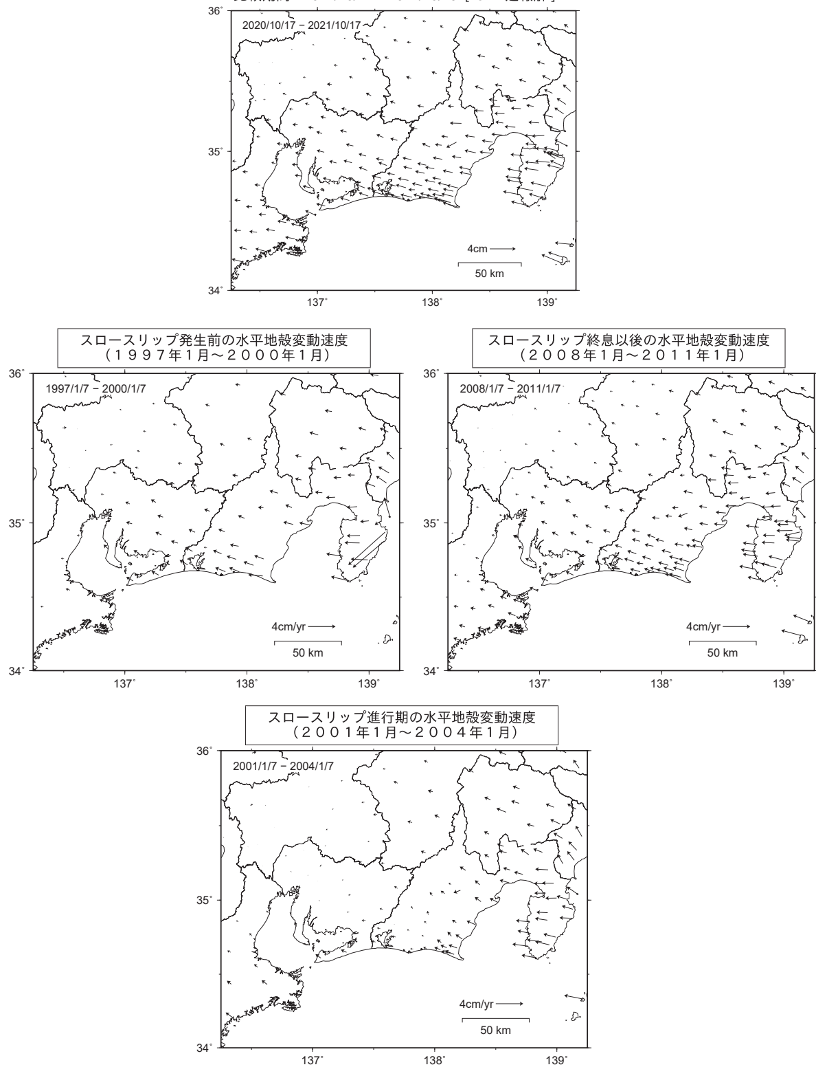
第 23 図 GNSS 観測による東海地方の最近 1 年間の水平変動及びスロースリップ開始前・進行期・終息後の水平変動速度（白鳥固定）
