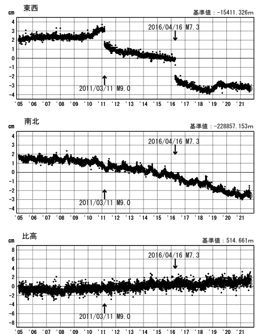
第 18 図 南海トラフ周辺における GNSS 連続観測結果: 1 次トレンド及び年周・半年周成分を除去した時系列 (固定局: 三隅)
