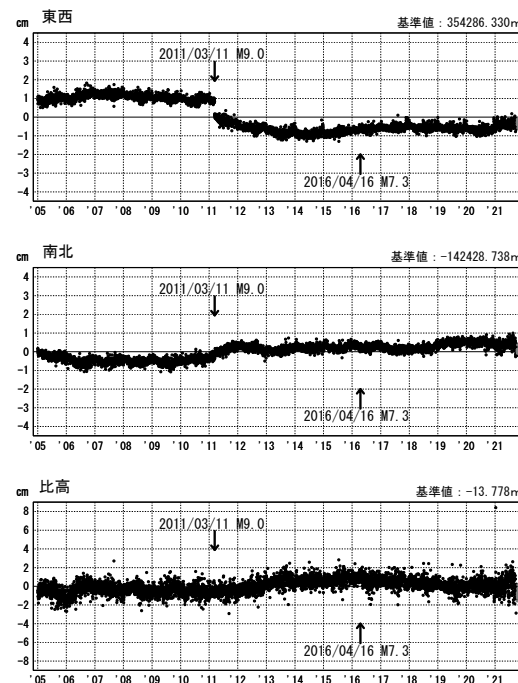
第 16 図 南海トラフ周辺における GNSS 連続観測結果: 1 次トレンド及び年周・半年周成分を除去した時系列 (固定局: 三隅)
