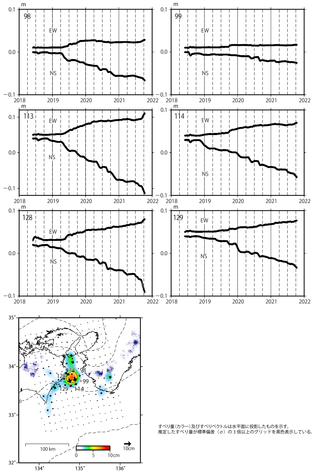
第 6 図 時間依存インバージョンで推定されたプレート間滑りの時間変化 Fig. 6 Time evolution of the estimated slip by the time dependent inversion method.
