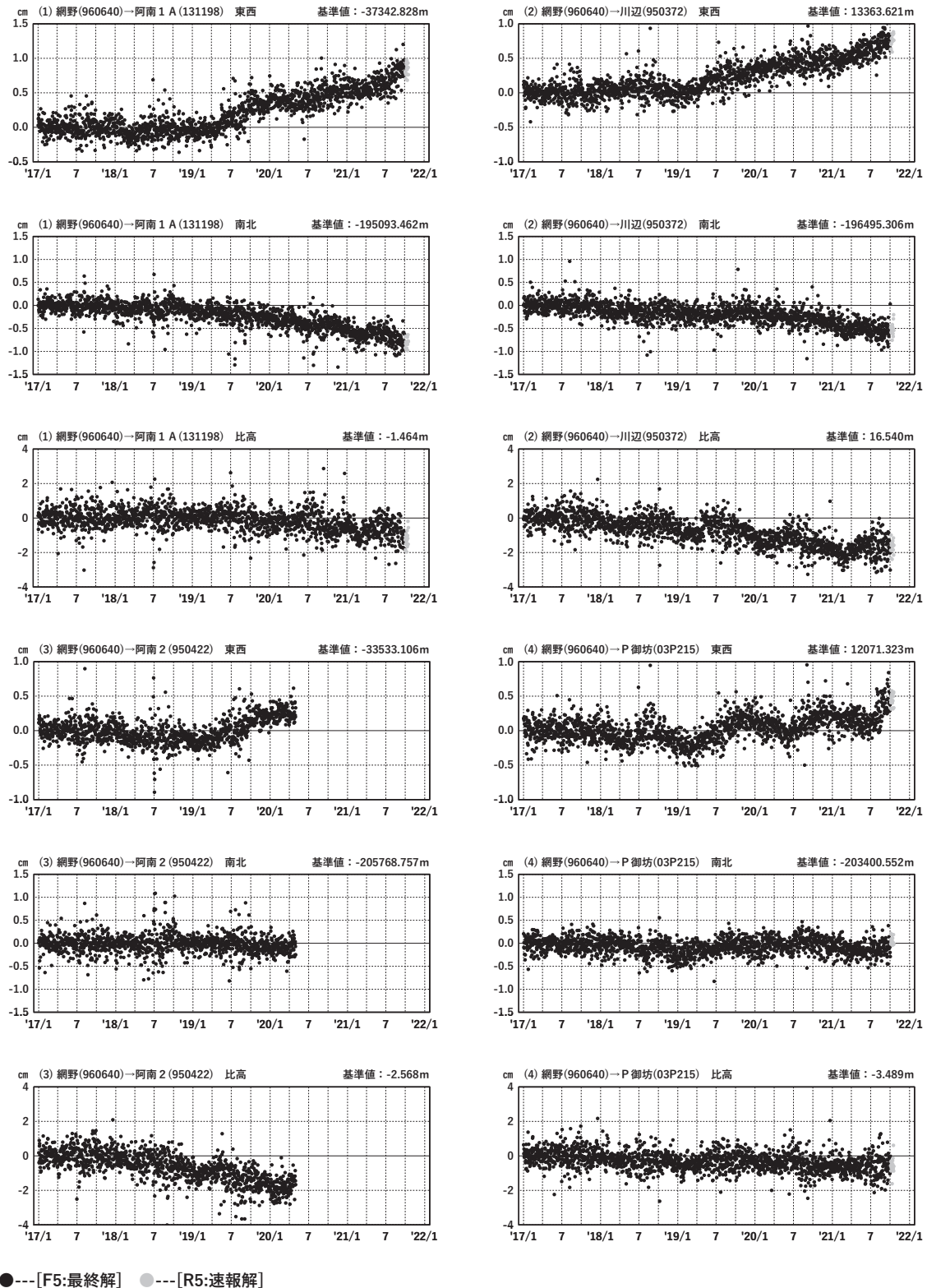
第 2 図 紀伊半島西部・四国東部 GNSS 連続観測時系列
