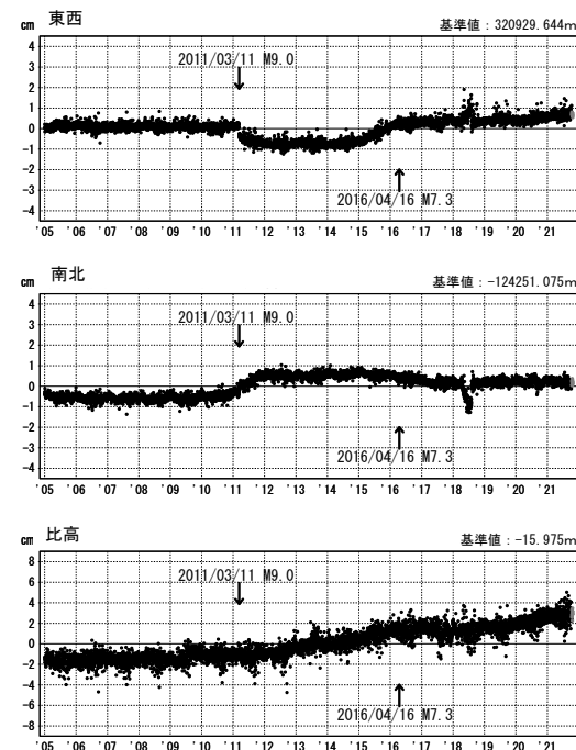
第 16 図 南海トラフ周辺における GNSS 連続観測結果: 1 次トレンド及び年周・半年周成分を除去した時系列 (固定局: 三隅)
