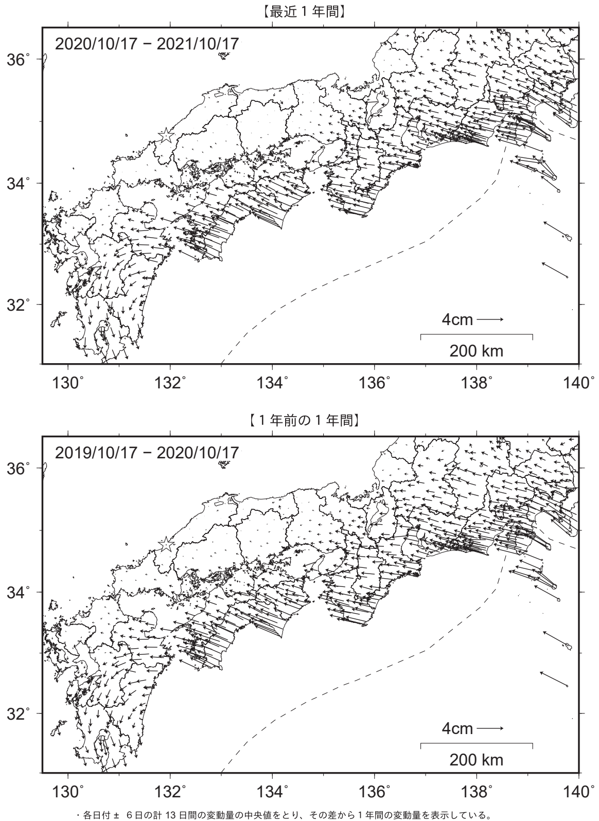
第 19 図 南海トラフ沿いの水平地殻変動（1 年間）：（上図）最近 1 年間（2020 年 10 月～2021 年 10 月），（下図）1 年前の 1 年間（2019 年 10 月～2020 年 10 月）。（固定局：三隅）
