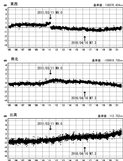
第 17 図 南海トラフ周辺における GNSS 連続観測結果: 1 次トレンド及び年周・半年周成分を除去した時系列 (固定局: 三隅)
