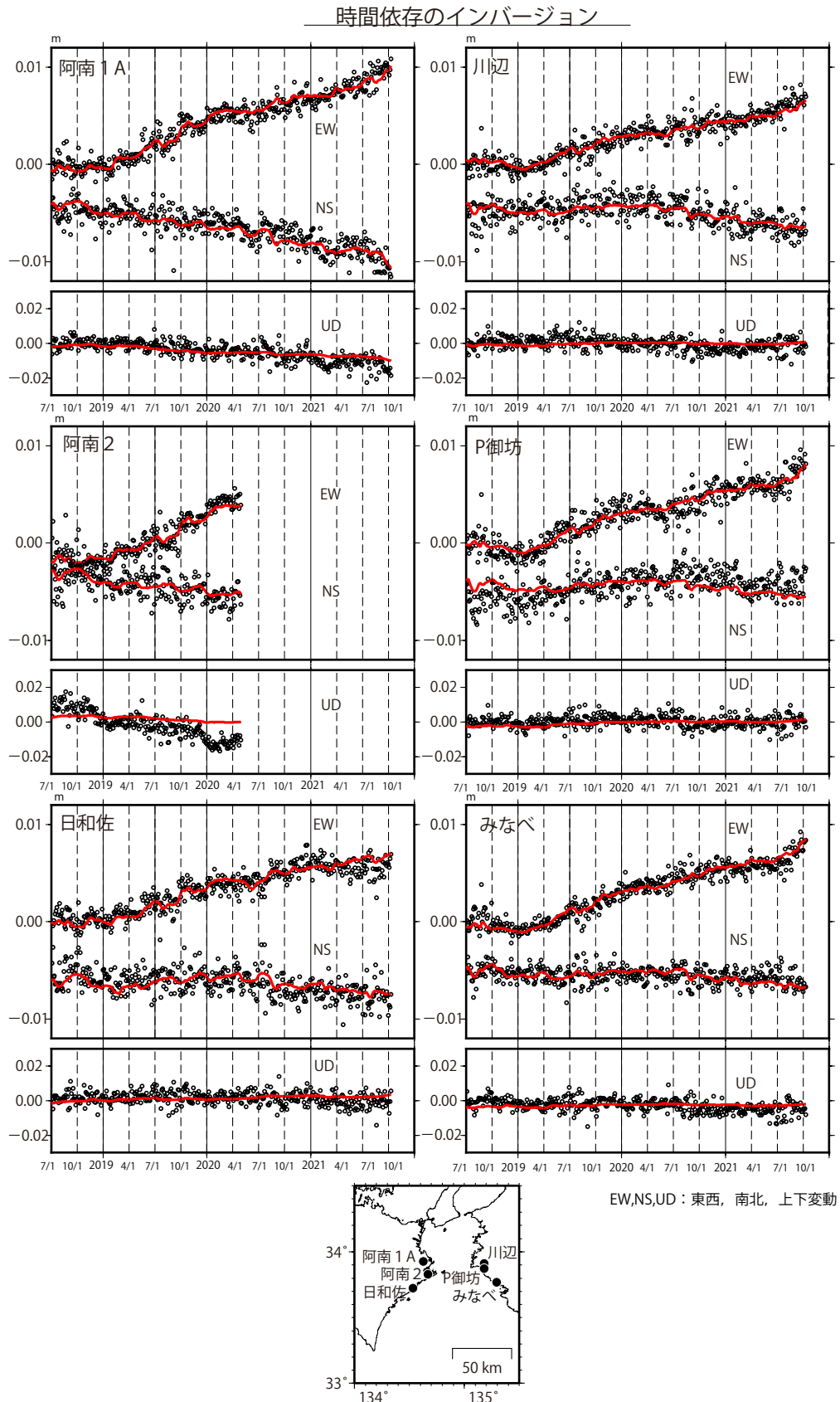
第 5 図 紀伊水道地域の座標時系列(黒丸)と計算値(赤線)
