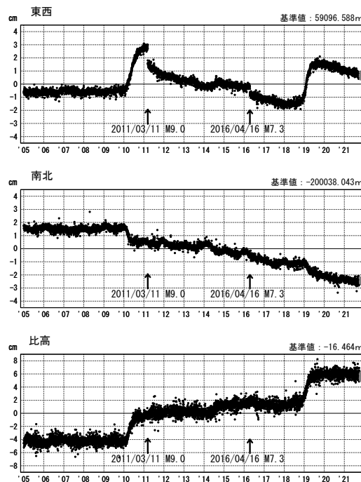
第 18 図 南海トラフ周辺における GNSS 連続観測結果: 1 次トレンド及び年周・半年周成分を除去した時系列 (固定局: 三隅)
