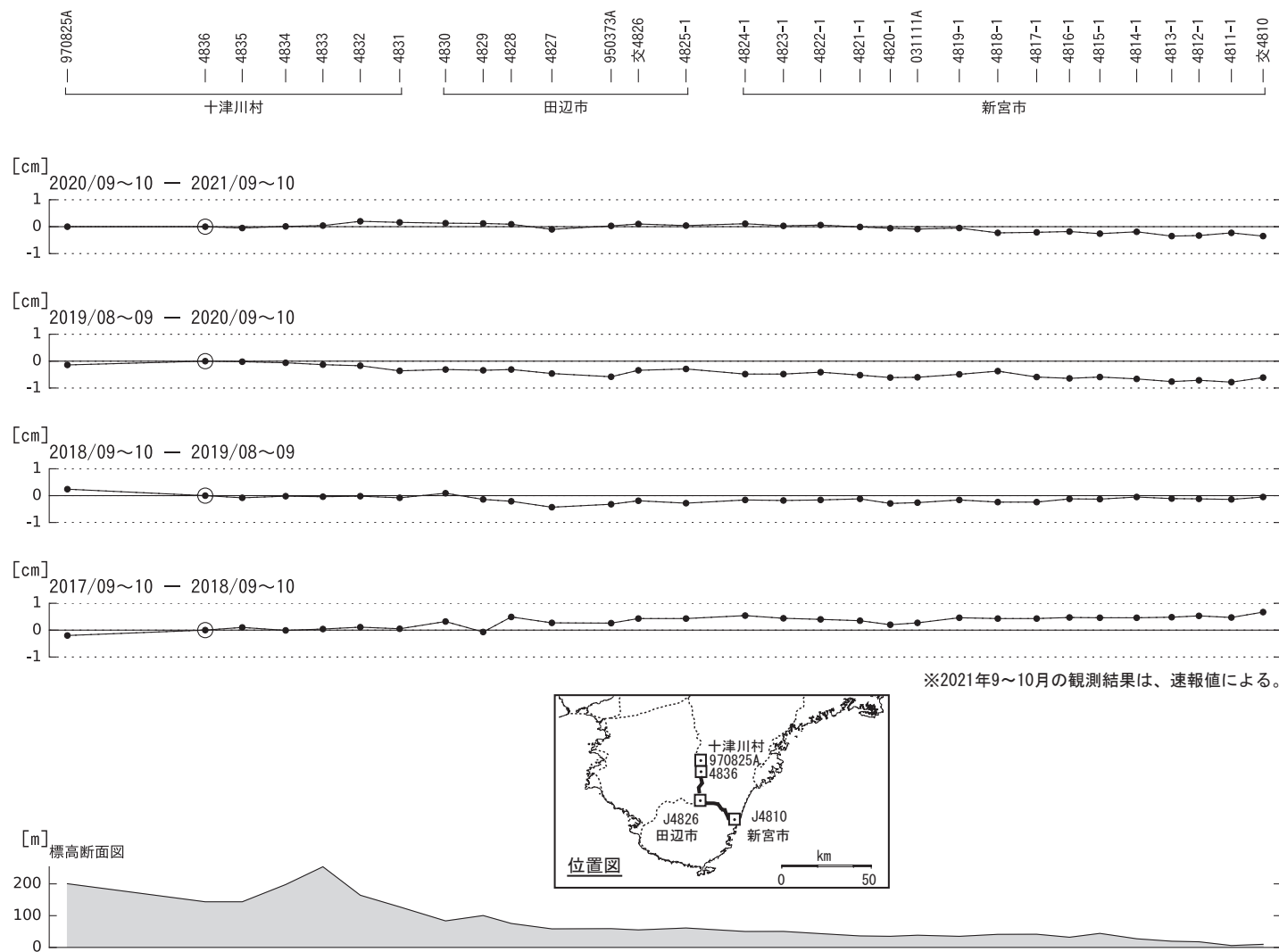
第 14 図 十津川村～新宮市間の上下変動
