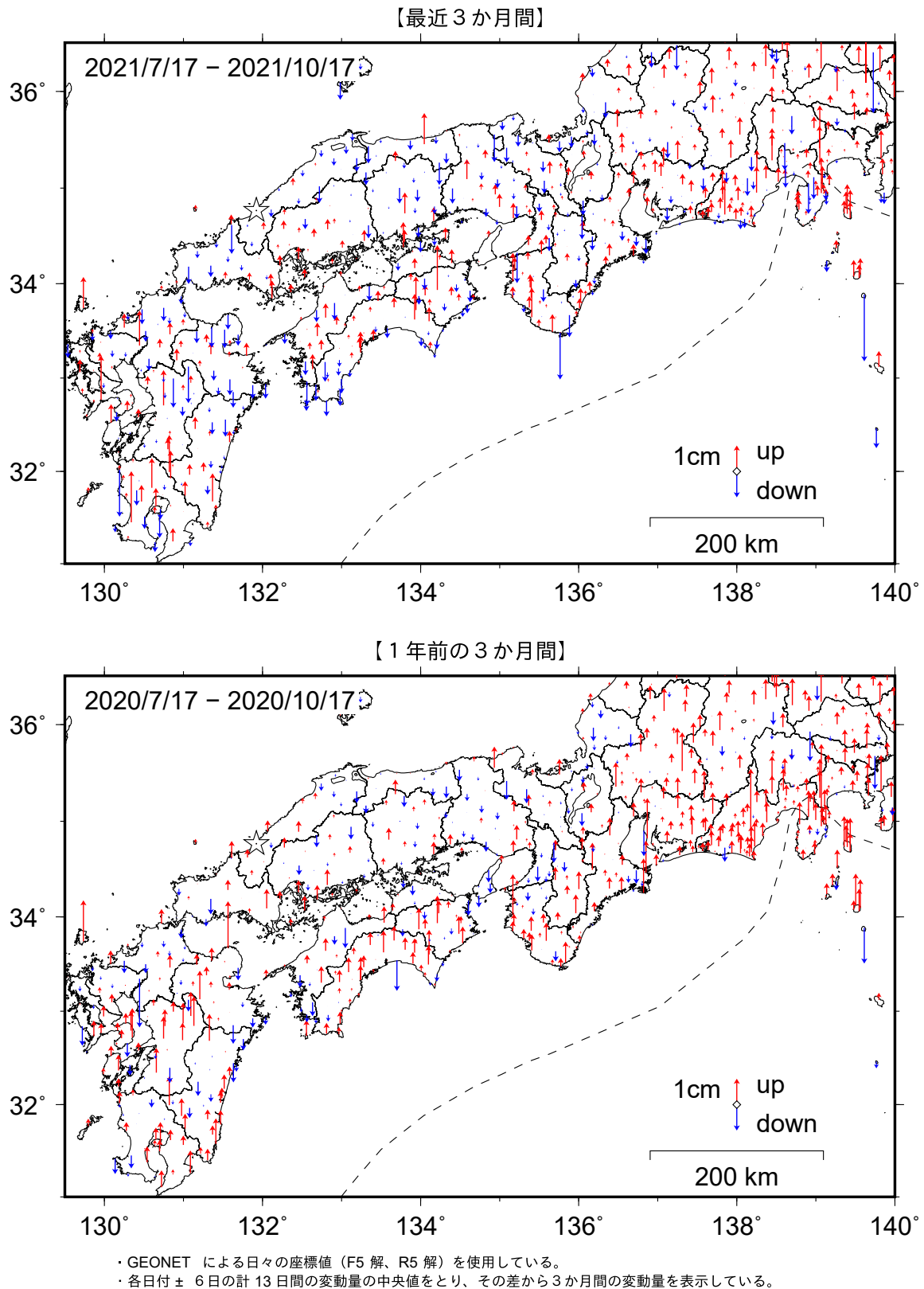
第 22 図 南海トラフ沿いの上下地殻変動 (3 か月間) : (上図) 最近 3 か月間 (2021 年 7 月 ~ 2021 年 10 月), (下図) 1 年前の 3 か月間 (2020 年 7 月 ~ 2020 年 10 月) (固定局 : 三隅)
