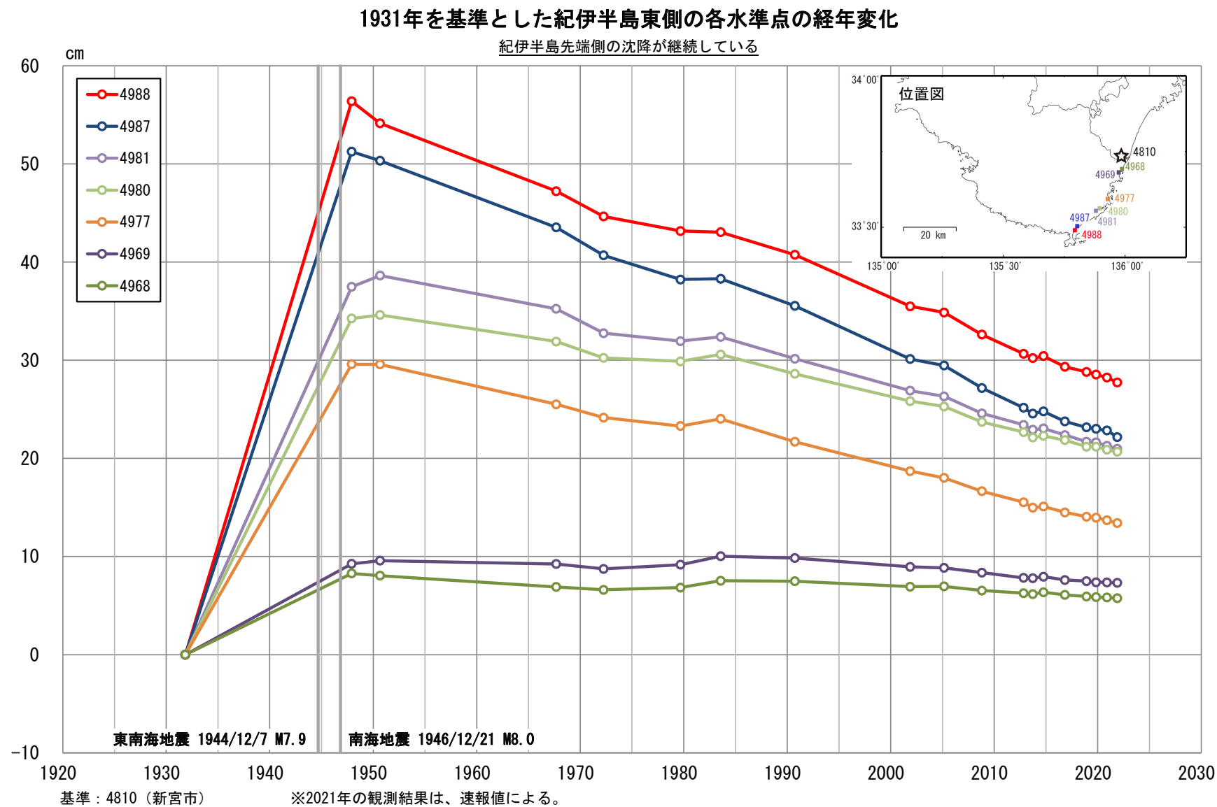
第 12 図 水準点 4810（新宮市）を基準とした紀伊半島東側の各水準点の高さの上下変動時系列
