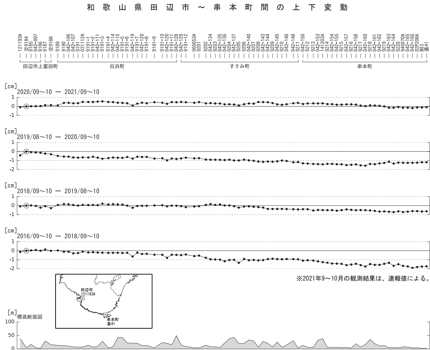
第 11 図 田辺市～串本町間の上下変動
