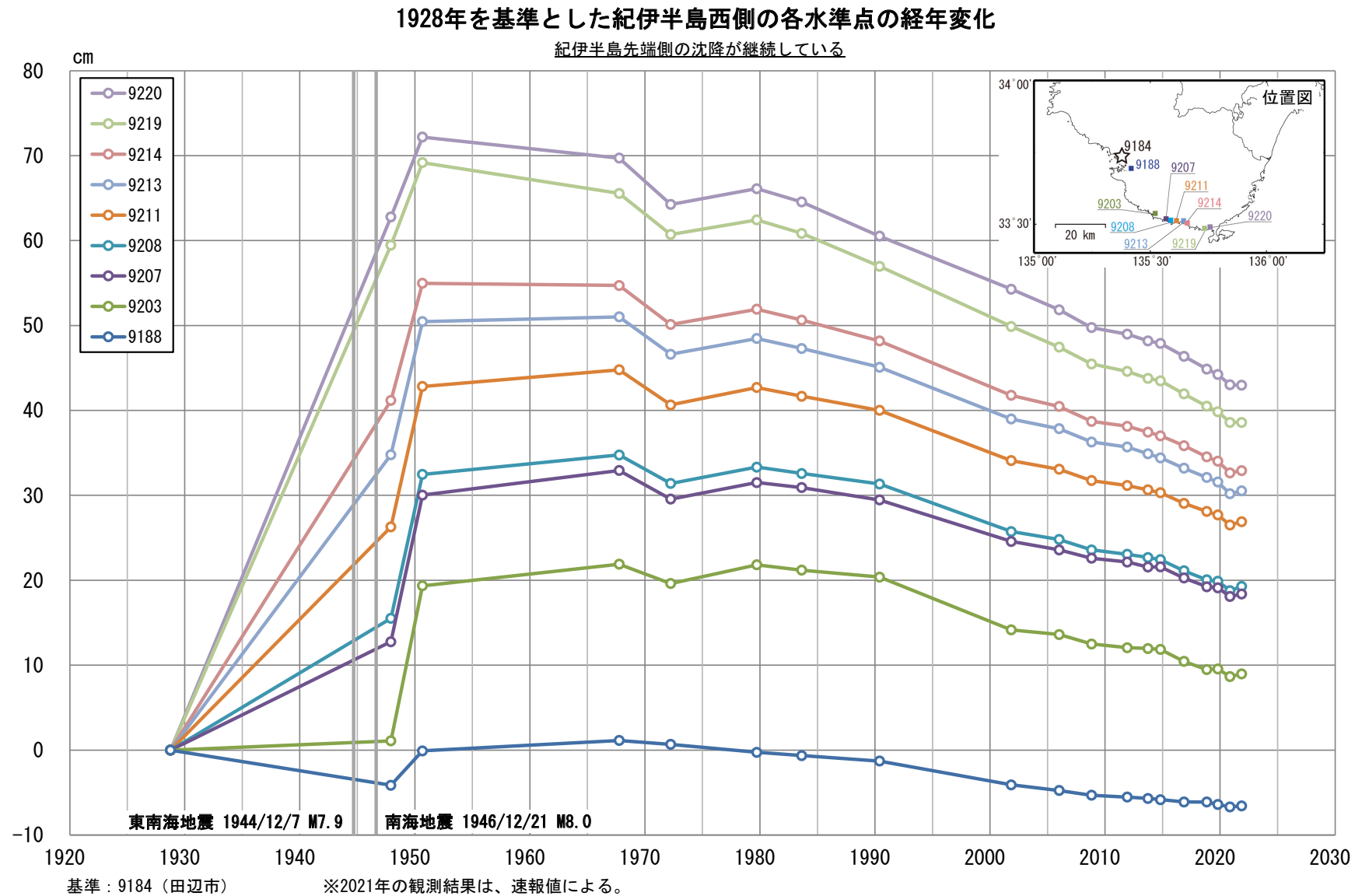
第 13 図 水準点 9184 (田辺市) を基準とした紀伊半島西側の各水準点の高さの上下変動時系列
