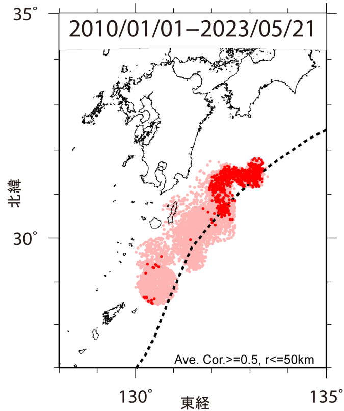
第 3 図 2010 年 1 月 1 日から 2023 年 5 月 21 日までの期間内に波形相関解析によって検出された超低周波イベントの震央分布。検出イベントを防災科研 Hi-net の手動または自動検測震源と照合して通常の地震を除去した後、それ以外を超低周波イベントとして桃色（2023 年 3 月 31 日以前）、および赤色（4 月 1 日以降）の点でそれぞれ示す。
