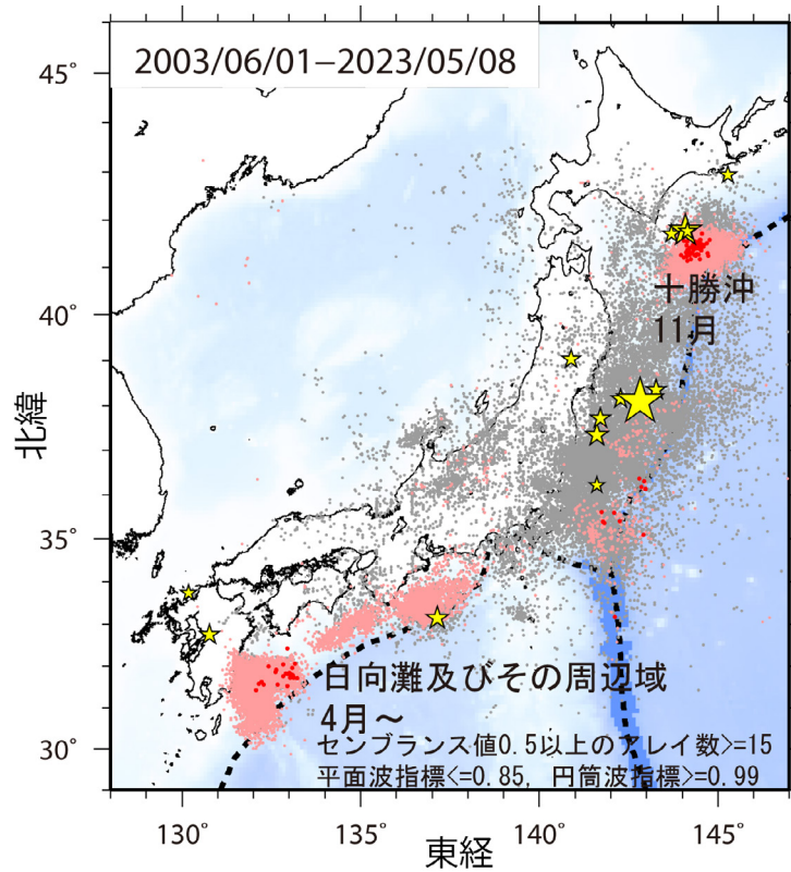
第 1 図 検出されたイベントの震央分布 (2003 年 6 月 1 日から 2023 年 5 月 8 日)。検出イベントを防災科研 Hi-net の手動または自動検測震源と照合し、対応する地震が見出されたイベントを灰色で、それ以外を桃色 (2022 年 10 月 31 日以前)、および赤色 (11 月 1 日以降) の点でそれぞれ示す。これらは主として周期 10 秒以上に卓越する超低周波地震を表すが、東北地方太平洋沖地震の発生以降は、除去しきれない通常地震を含む。期間内に発生した M7 以上の地震の震央を黄色星印で併せて示す (ただし、2011 年 3 月 11 日から 2015 年までの東日本は東北地方太平洋沖地震の本震のみ図示)。
