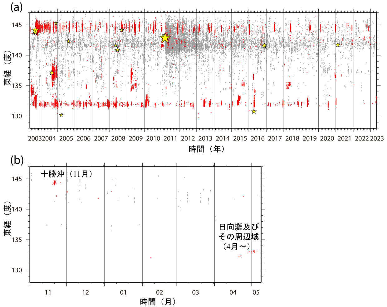
第 2 図 (a) 2003 年 6 月 1 日から 2023 年 5 月 8 日までの期間, (b) 2022 年 11 月 1 日から 2023 年 5 月 8 日までの期間に検出されたイベントの時空間分布. 検出されたイベントを防災科研 Hi-net 手動または自動検測震源と照合し, 対応する地震が見出されたイベントを灰色丸印で, それ以外を赤色丸印で示す.
