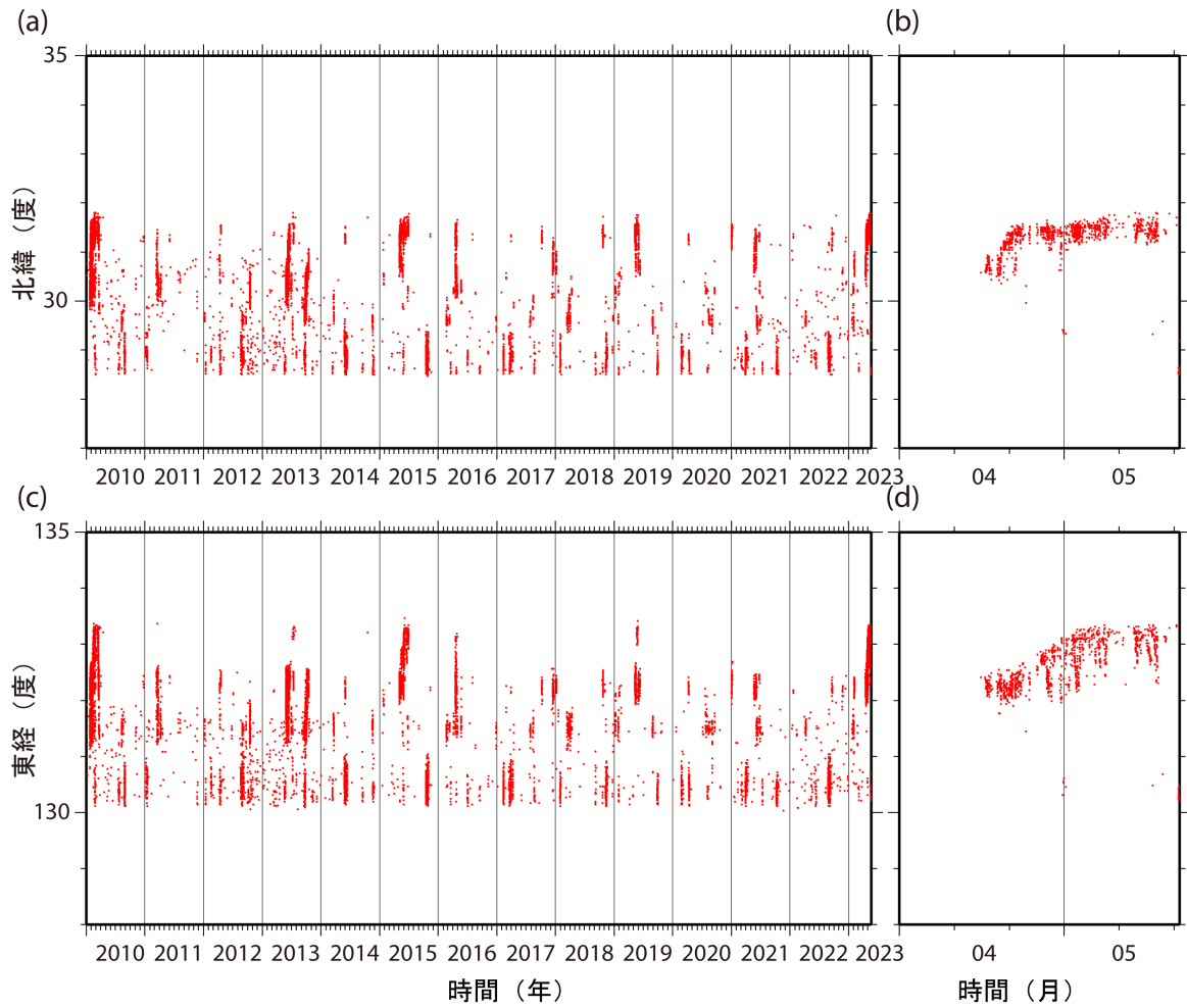
第 4 図 第 3 図と同じ期間内に検出された超低周波イベントの時空間分布。超低周波イベントを赤色の点で示す。(a) および (b) に緯度分布の、(c) および (d) に経度分布の時間変化をそれぞれ示す。また、(a) および (c) に 2010 年 1 月 1 日以降、(b) および (d) には 2023 年 4 月 1 日以降の分布をそれぞれ示す。
