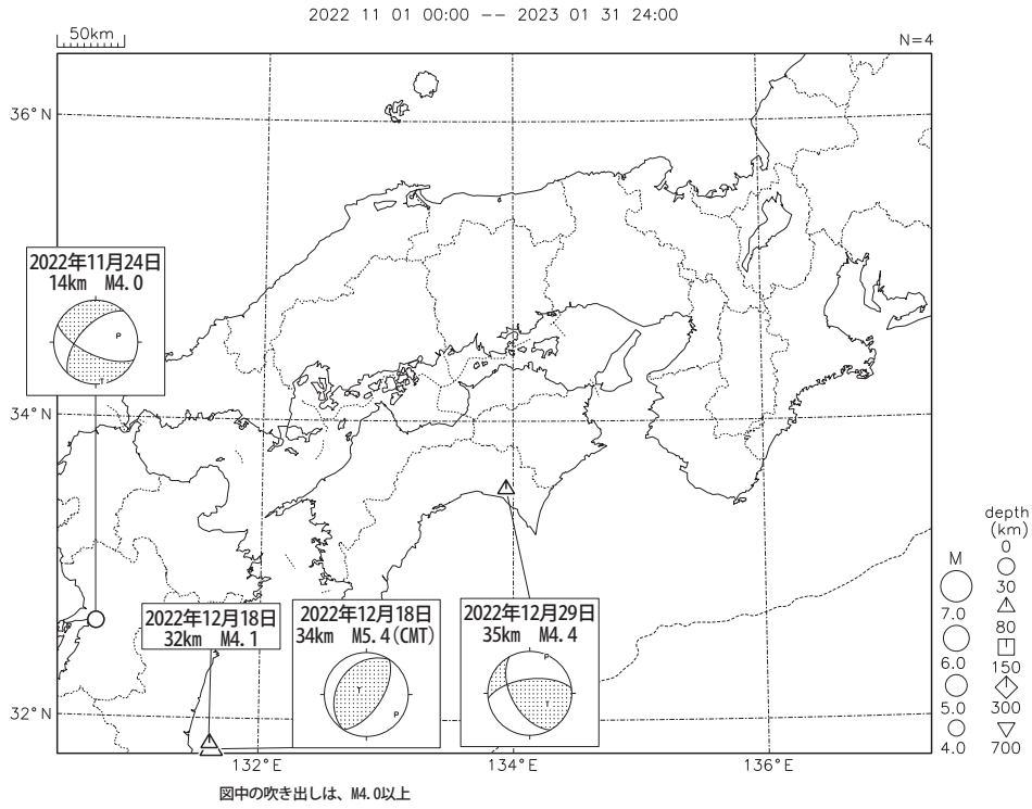
第 1 図 (a) 近畿・中国・四国地方とその周辺の地震活動 (2022 年 11 月 ~ 2023 年 1 月, M \geq 4.0 , 深さ \leq 700 km) Fig.1(a) Seismic activity in and around the Kinki, Chugoku and Shikoku districts (November 2022 – January 2023, M \geq 4.0 , depth \leq 700 km)
