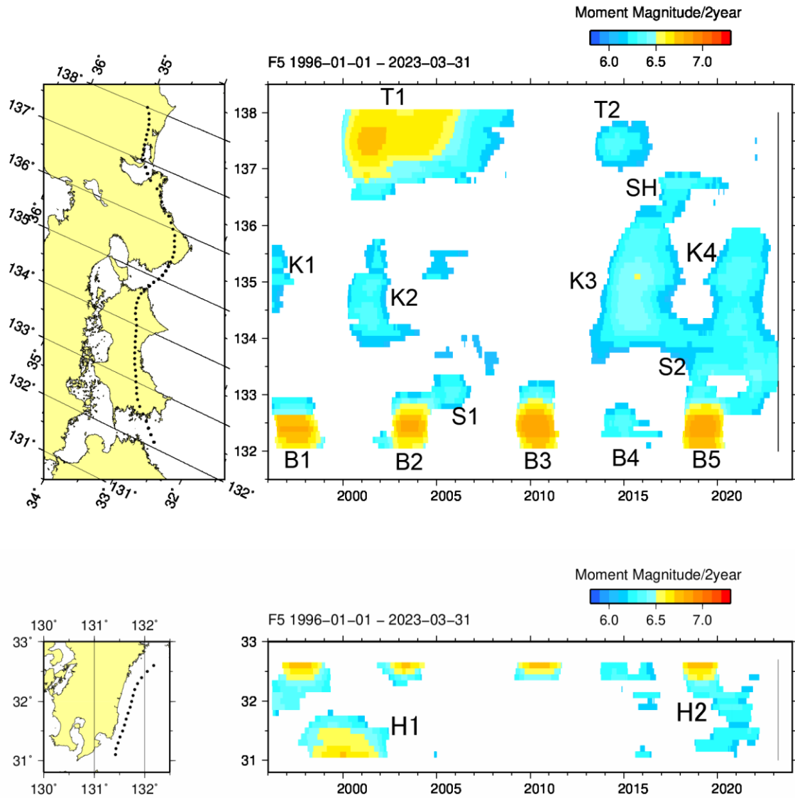
第 2 図 長期的スロースリップの規模分布 (1996 年から 2023 年 3 月) 2 年間あたりの変化量から推定したモーメントマグニチュード。イベントの略号は第 1 図と同じ。 Fig. 2 Moment magnitude distribution of long-term slow slip events. The event abbreviations are the same as in Fig. 1.
