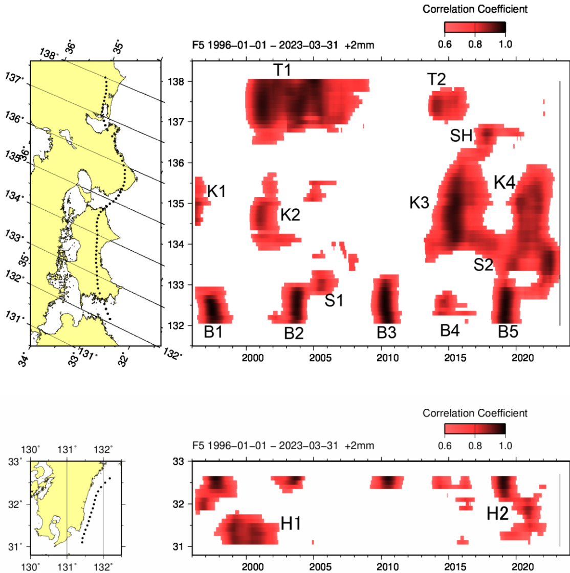
第 1 図 長期的スロースリップ客観検知図（1996 年から 2023 年 3 月）
