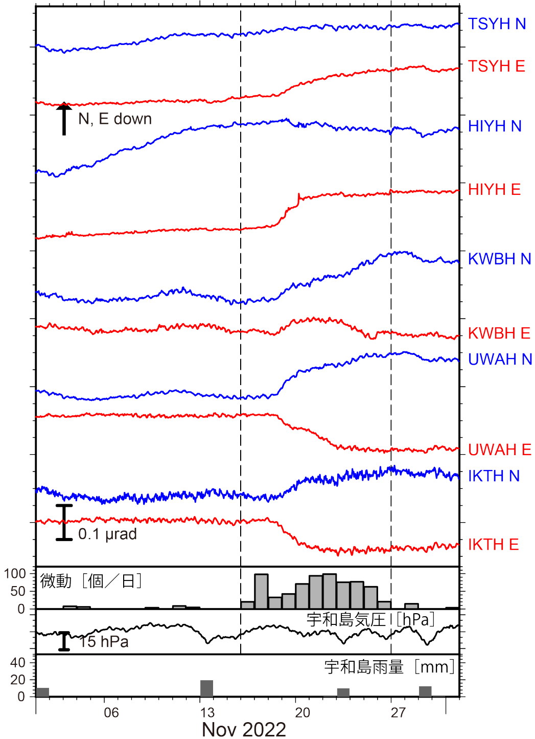
第 2 図 2022 年 11 月 1 日から 12 月 1 日までの傾斜時系列. 観測点位置は第 3 図に示した. 記録は上方向への変化が北・東下がりの傾斜変動を表す. 気圧応答・潮汐成分を BAYTAP-G 4) により除去し, 直線トレンドを補正した後の記録を示した. 11 月 16 日～11 月 26 日の傾斜変化量を SSE によるものと仮定した. 四国西部～中部での微動活動度・気象庁宇和島観測点での気圧変化および雨量をあわせて表示した.
