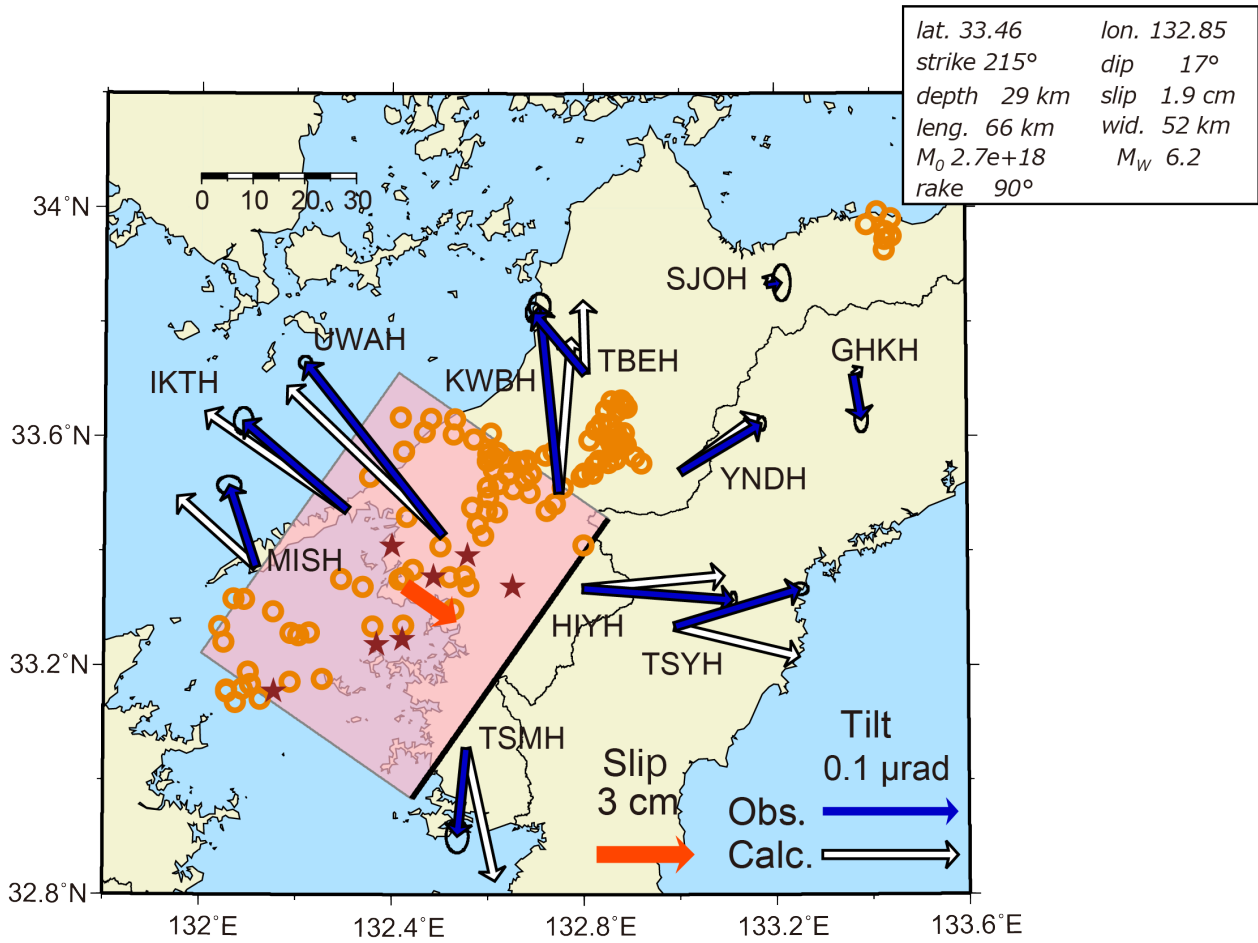
第 3 図 2022 年 11 月四国西部の短期的 SSE の断層モデル。第 2 図の破線で示された期間に観測された傾斜変化ベクトル (青矢印)・このデータから推定された SSE の断層モデル (赤矩形・矢印)・モデルから計算される傾斜変化ベクトル (白抜き矢印) を示す。同じ期間の微動と VLFE の震央を橙円と茶星印で示した。
