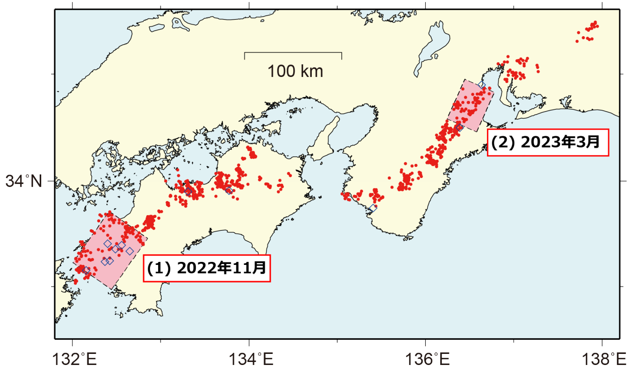
第 1 図 2022 年 11 月 1 日～2023 年 4 月 30 日の期間に検知された短期的 SSE (ピンク矩形)、同期間に発生した深部低周波微動 (赤点) 及び VLFE の震央 (青菱形) を重ねて表示した。 Fig. 1. Distribution of SSEs detected from November 1, 2022, to April 30, 2023. Red dots and blue diamonds show epicenters of tremors and VLFEs, respectively.
