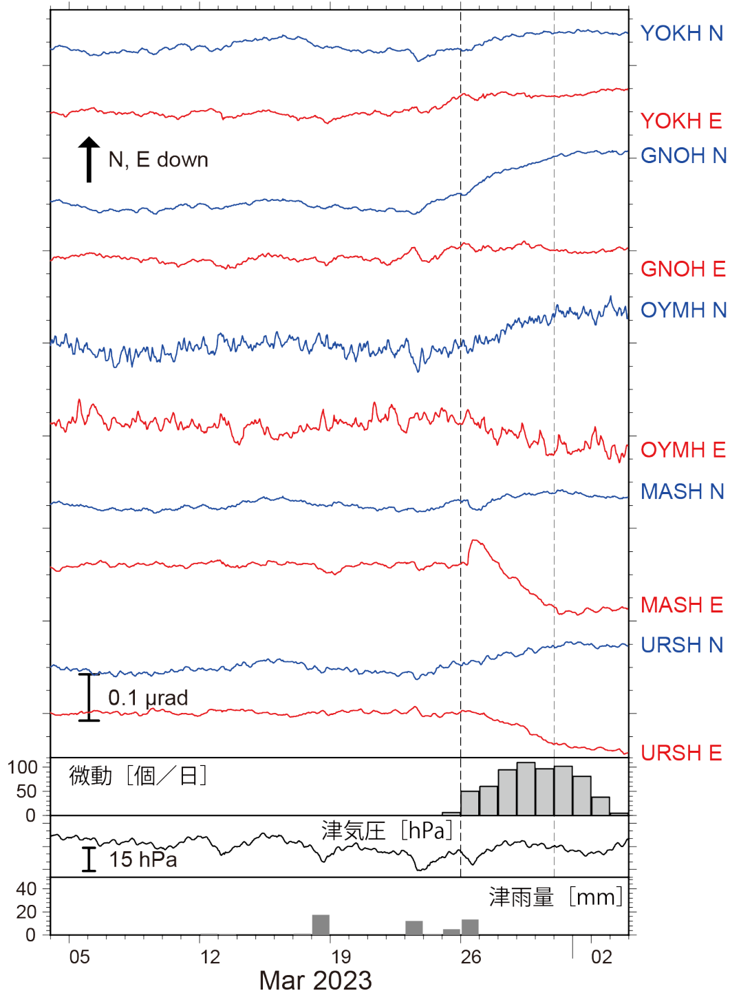
第 4 図 2023 年 3 月 4 日～4 月 3 日までの傾斜時系列. 図の見方は第 2 図と同様. 観測点位置は第 5 図に示した. 3 月 26 日～3 月 30 日の傾斜変化量を SSE によるものと仮定した. 紀伊半島～愛知県での微動活動度・気象庁津観測点での気圧変化および雨量をあわせて表示した.
