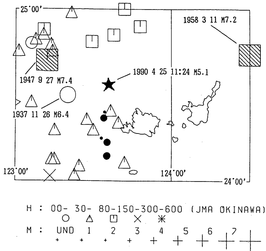
第1図 石垣島近海の地震 (M: 5.1) とその余震及びその付近における過去 (M: ≥ 5) の地震の震央分布 (1926~1989年)
