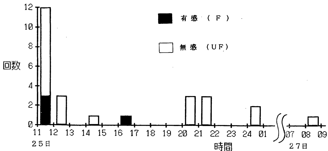
第2図 与那国島及び石垣島で観測された時間別地震発生回数 (67型・1,000倍) F:有感, UF:無感
