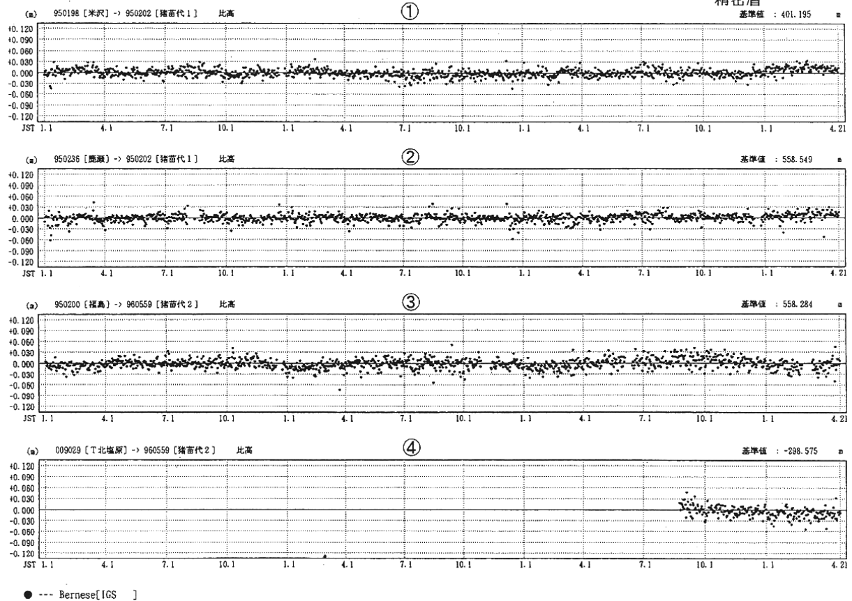
第4図-(2) 磐梯山周辺GPS連続観測結果(2)
