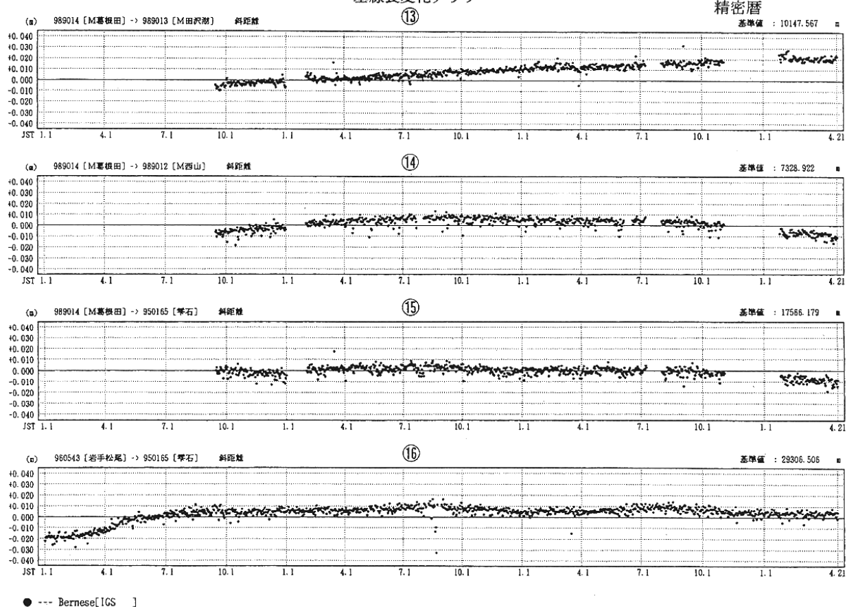
第2図-(2) 岩手山周辺GPS連続観測結果(2)
