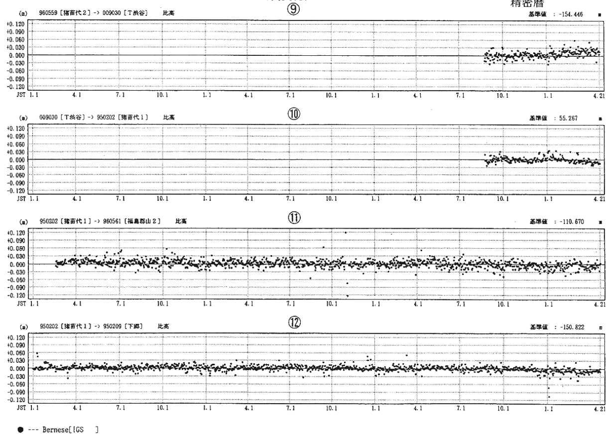
第4図-(3) 磐梯山周辺GPS連続観測結果(3)
