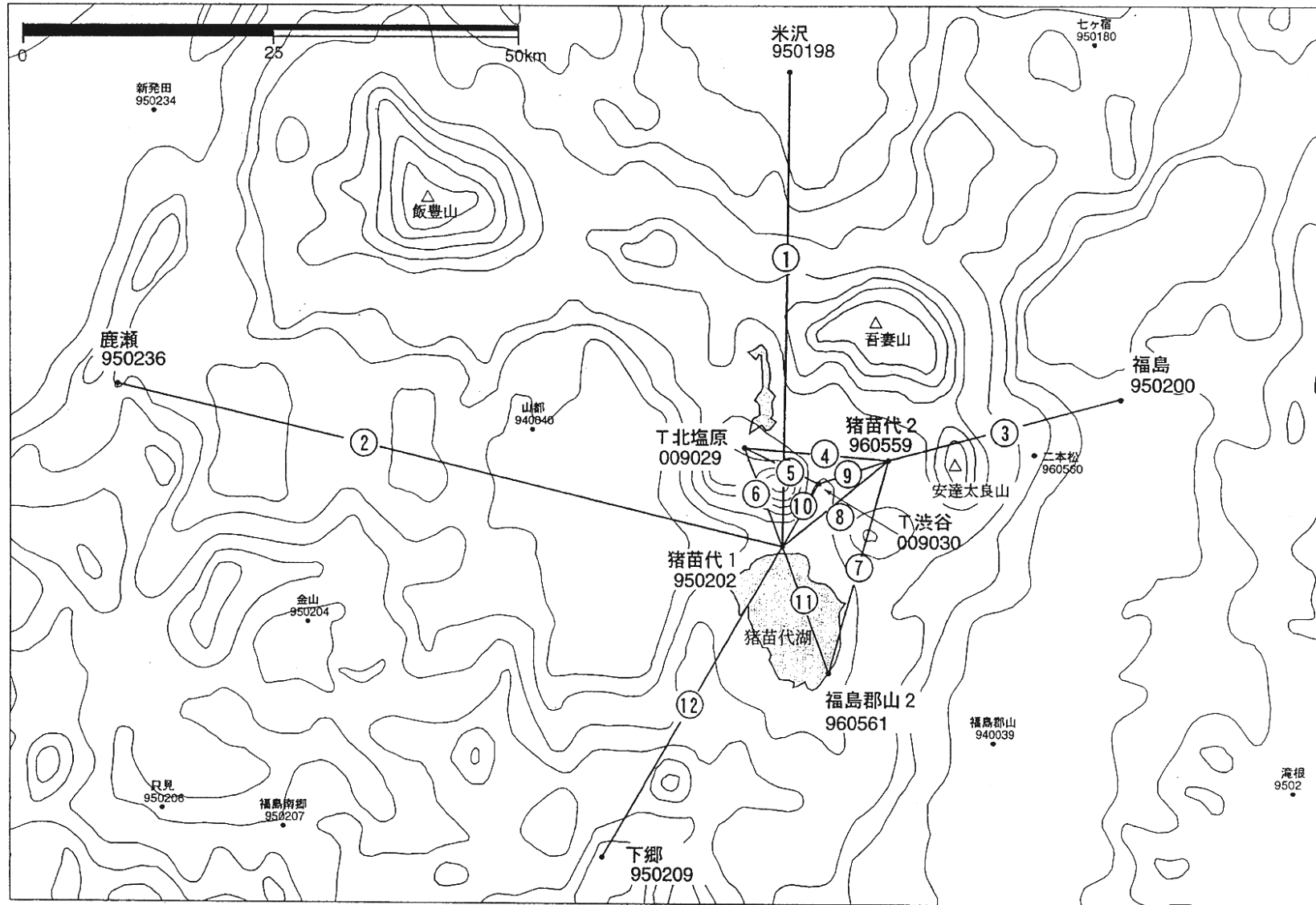
第3図 磐梯山周辺GPS連続観測結果
