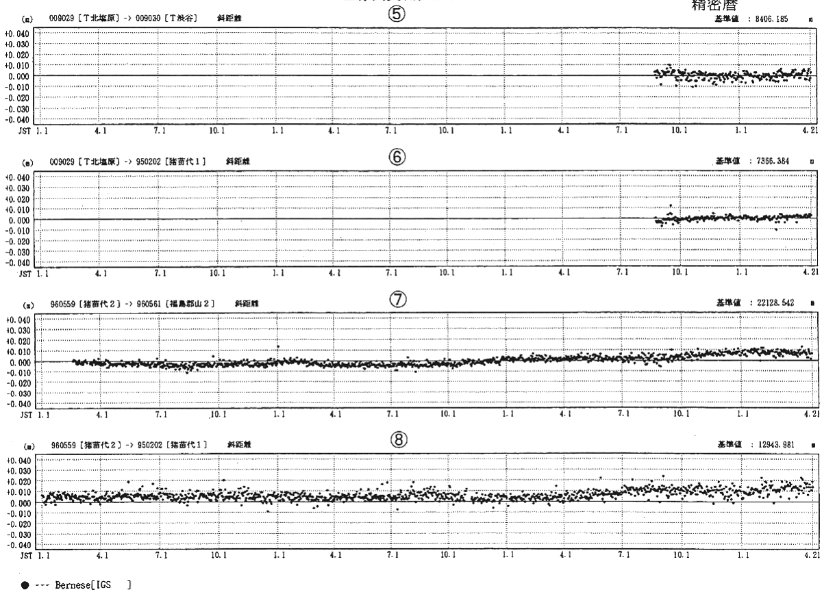
第4図-(1) 磐梯山周辺GPS連続観測結果(1)
