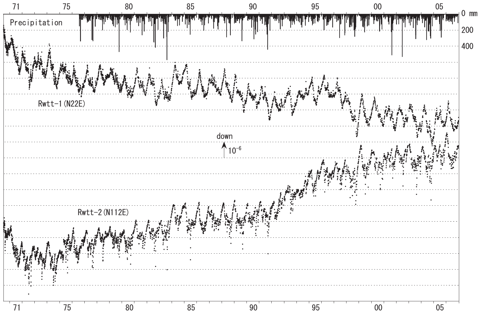
第3図 富士川観測所における読取型水管傾斜計により観測された傾斜変化の読取值および日雨量 Fig.3 Daily mean tilt data observed water-tube tiltmeters and daily precipitation data
