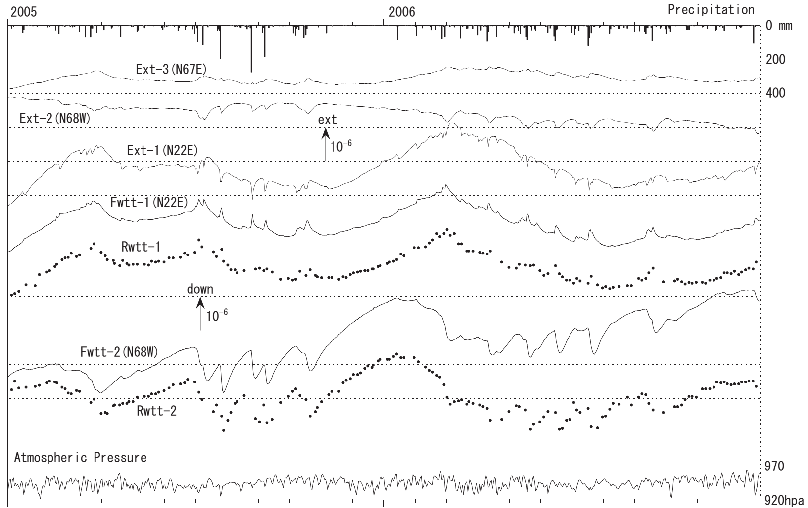
第1図 富士川観測所における水晶管伸縮計・水管傾斜計（実線=フロート型・黒丸=読取型）記録、 気圧の日平均記録および日降雨量（2005, 2006年） Fig.1 The earth's strain, tilt (solid=float type WTT, dots=reading type WTT), atmospheric pressure (daily mean) and daily precipitation at the Fujigawa observatory in 2005-2006.
