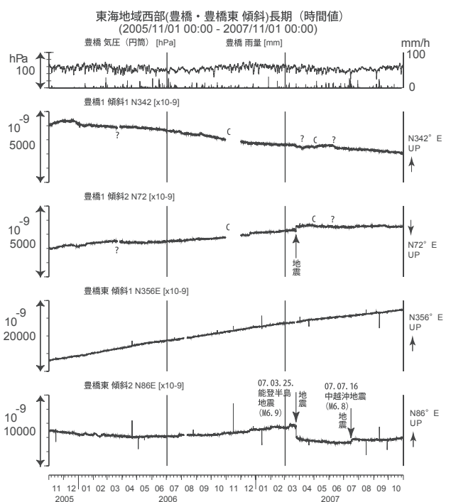
第 24 図 東海地域西部 (豊橋・豊橋東) の傾斜の観測結果 (2005 年 11 月～2007 年 10 月) Fig.24 Observed tilts at the Toyohashi and Toyohashi-higashi observation sites from Nov. 2005 to Oct. 2007.
