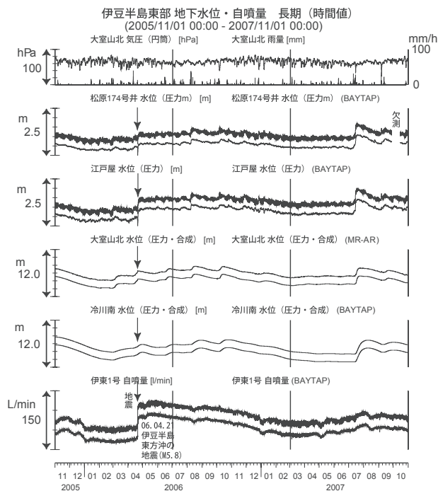
第27図 伊豆半島東部の地下水等の観測結果(2005 年11月～2007年10月) Fig.27 Observed groundwater levels and others in the eastern Izu peninsula from Nov. 2005 to Oct. 2007.
