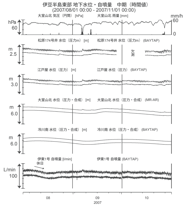
第 18 図 伊豆半島東部の地下水等の観測結果 (2007 年 8 月～2007 年 10 月)
