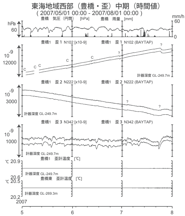
第13図 東海地域西部(豊橋)の歪等の観測結果 (2007年5月～2007年7月)
