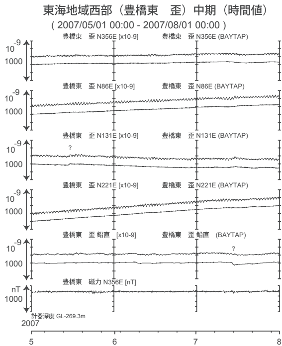
第15図 東海地域西部(豊橋東)の歪等の観測結果 (2007年5月～2007年7月)
