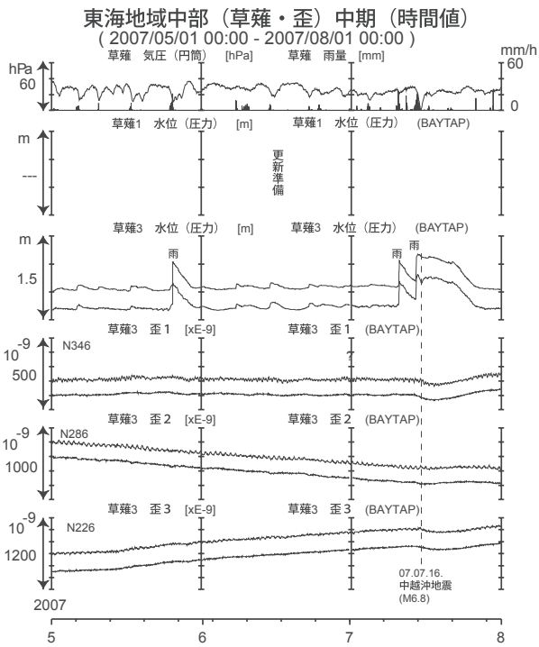
第5図 草薙観測井の地下水・歪の観測結果(2007年5月～2007年7月) Fig.5 Observed groundwater levels and strain at the Kusanagi observation site from May 2007 to July 2007.
