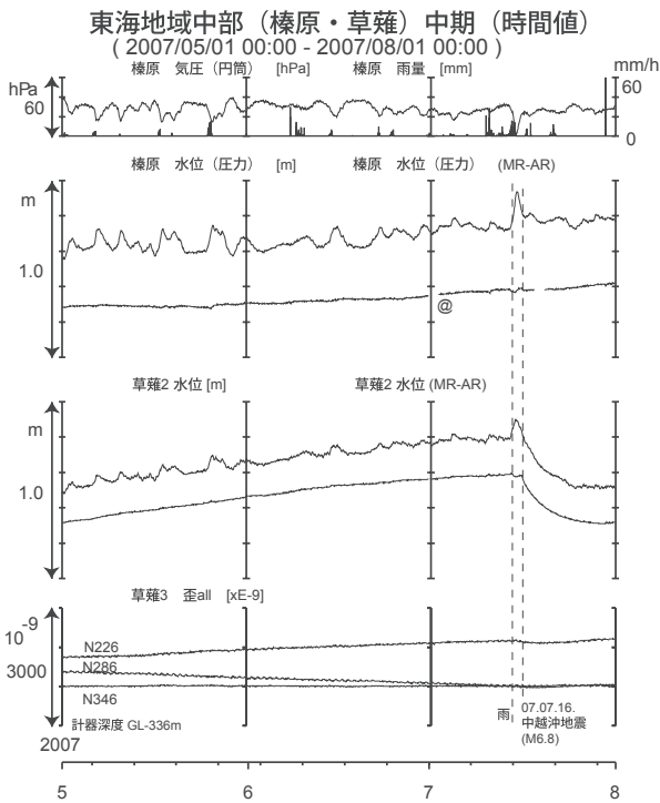
第3図 東海地域中部の地下水等の観測結果(2007年5月～2007年7月)
