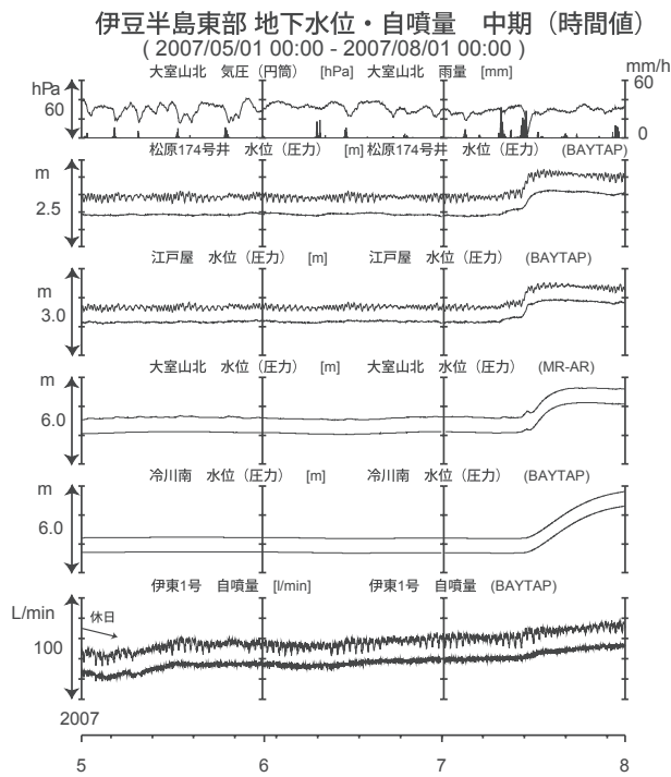
第 17 図 伊豆半島東部の地下水等の観測結果 (2007 年 5 月～2007 年 7 月)
