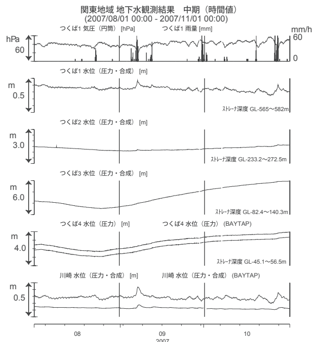
第 20 図 関東地域の地下水等の観測結果 (2007 年 8 月～2007 年 10 月)
