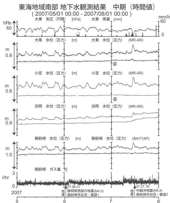
第7図 東海地域南部の地下水等の観測結果(2007年5月～2007年7月) Fig.7 Observed groundwater levels and others in the southern Tokai district from May 2007 to July 2007.
