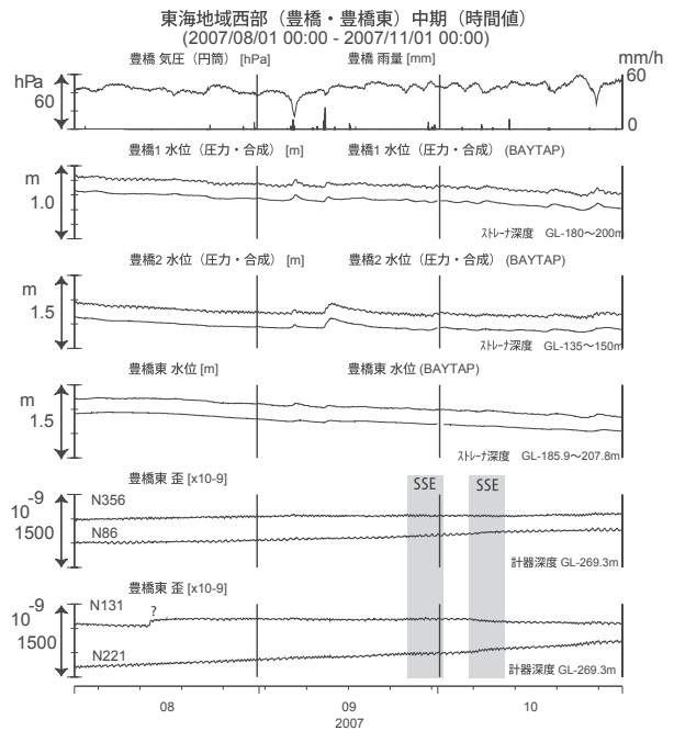
第10図 東海地域西部(豊橋・豊橋東)の地下水等の観測結果(2007年8月~2007年10月) Fig.10 Observed groundwater levels and others at the Toyohashi and Toyohashi-higashi observation sites from Aug. 2007 to Oct. 2007.
