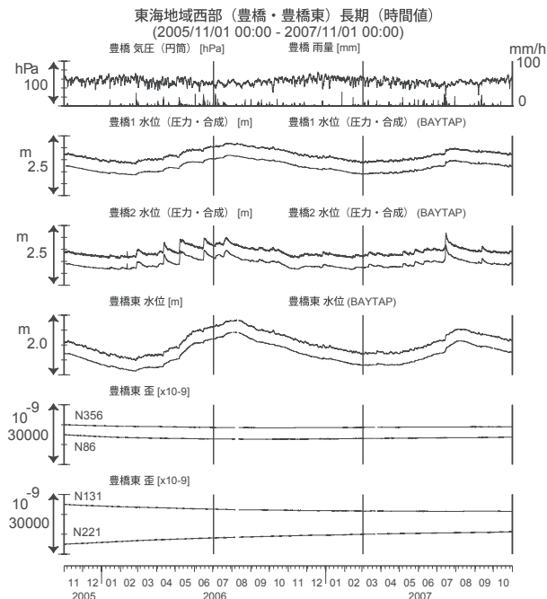
第 23 図 東海地域西部 (豊橋・豊橋東) の地下水等の観測結果 (2005 年 11 月～2007 年 10 月) Fig.23 Observed groundwater levels and others at the Toyohashi and Toyohashi-higashi observation sites in the western Tokai district from Nov. 2005 to Oct. 2007.
