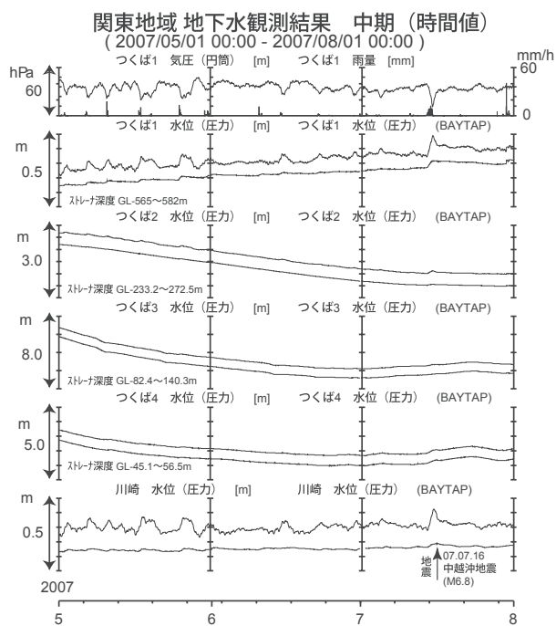
第 19 図 関東地域の地下水等の観測結果 (2007 年 5 月～2007 年 7 月)
