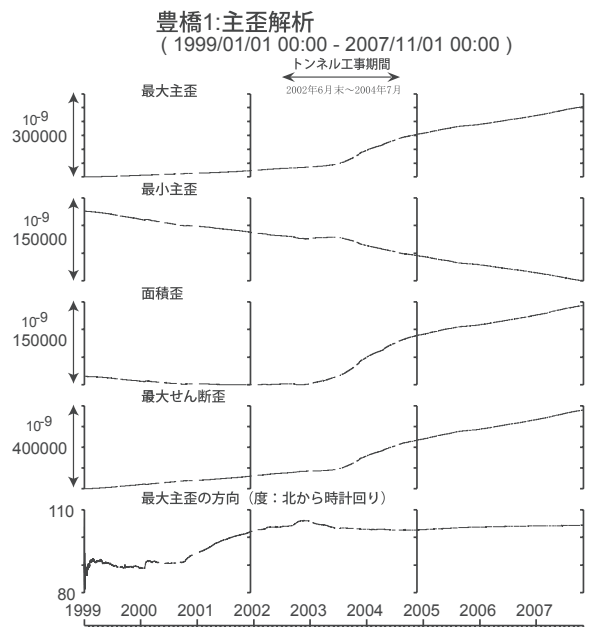
第32図 豊橋における主歪解析の結果(1999年1月～2007年10月) Fig.32 Result of the principal strain analysis at the Toyohashi observation well from Jan. 1999 to Oct. 2007.
