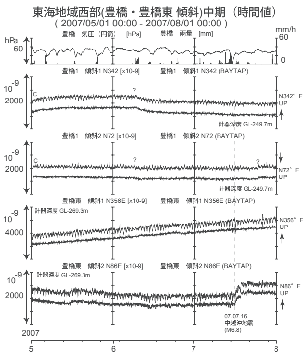
第11図 東海地域西部(豊橋・豊橋東)の傾斜の観測結果(2007年5月~2007年7月) Fig.11 Observed tilts at the Toyohashi and Toyohashi-higashi observation sites from May 2007 to July 2007.
