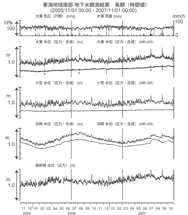
第 22 図 東海地域南部の地下水等の観測結果 (2005 年 11 月～2007 年 10 月) Fig.22 Observed groundwater levels and others in the southern Tokai district from Nov. 2005 to Oct. 2007.
