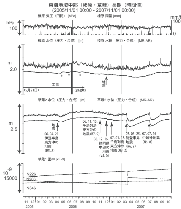
第 21 図 東海地域中部の地下水等の観測結果 (2005 年 11 月～2007 年 10 月) Fig.21 Observed groundwater levels and others in the central Tokai district from Nov. 2005 to Oct. 2007.
