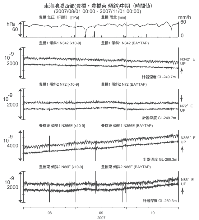
第12図 東海地域西部(豊橋・豊橋東)の傾斜の観測結果(2007年8月~2007年10月) Fig.12 Observed tilts at the Toyohashi and Toyohashi-higashi observation sites from Aug. 2007 to Oct. 2007.
