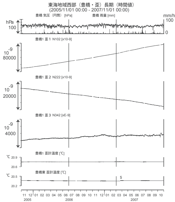
第25図 東海地域西部(豊橋)の歪等の観測結果 (2005年11月～2007年10月) Fig.25 Observed strain and others at the Toyohashi observation site from Nov. 2005 to Oct. 2007.
