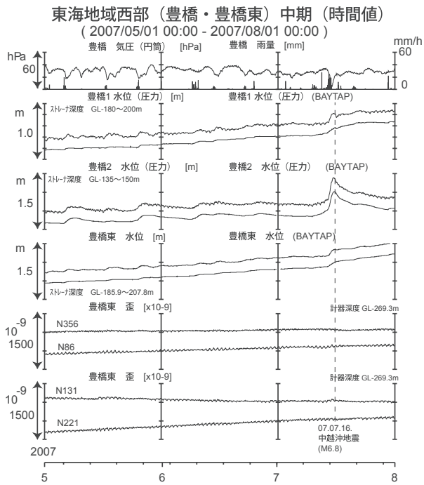
第9図 東海地域西部(豊橋・豊橋東)の地下水等の観測結果(2007年5月~2007年7月) Fig.9 Observed groundwater levels and others at the Toyohashi and Toyohashi-higashi observation sites from May 2007 to July 2007.
