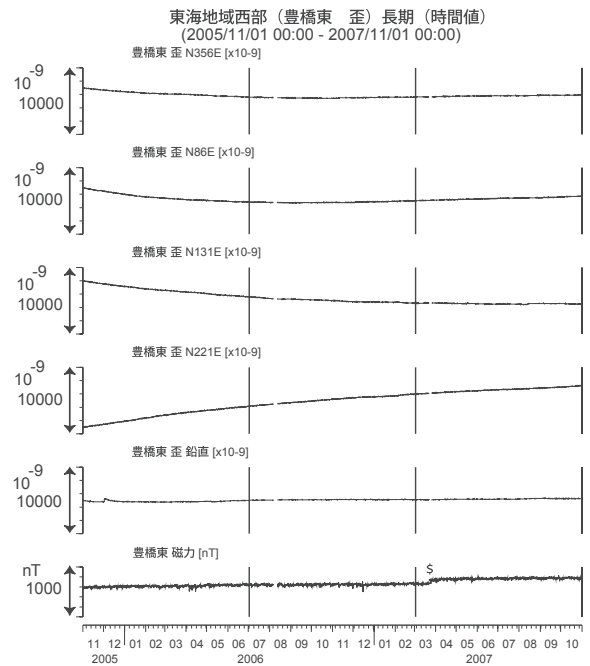
第26図 東海地域西部(豊橋東)の歪等の観測結果 (2005年11月～2007年10月) Fig.26 Observed strain and others at the Toyohashi- higashi observation site from Nov. 2005 to Oct. 2007.
