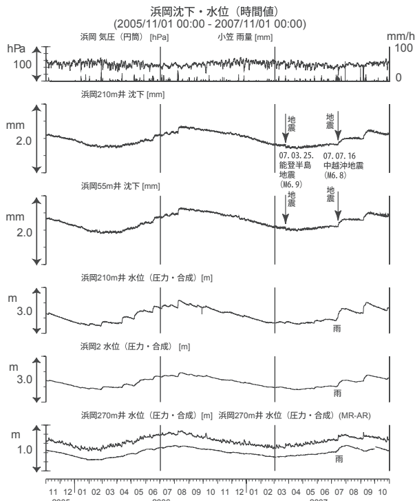
第29図 浜岡における沈下等の観測結果(2005年11月～2007年10月) Fig.29 Observed subsidence data and others at the Hamaoka observation well from Nov. 2005 to Oct. 2007.
