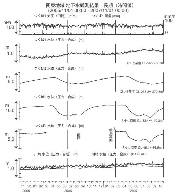
第28図 関東地域の地下水等の観測結果(2005年11 月～2007年10月) Fig.28 Observed groundwater levels and others in the Kanto district from Nov. 2005 to Oct. 2007.
