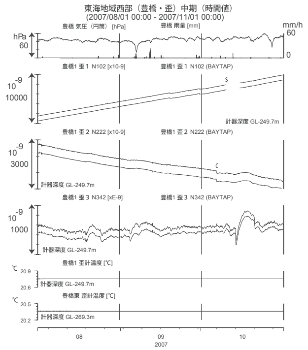
第14図 東海地域西部(豊橋)の歪等の観測結果 (2007年8月～2007年10月)
