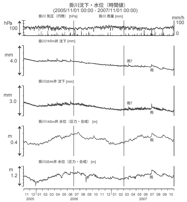
第30図 掛川における沈下等の観測結果(2005年11月～2007年10月) Fig.30 Observed subsidence data and others at the Kakegawa observation well from Nov. 2005 to Oct. 2007.
