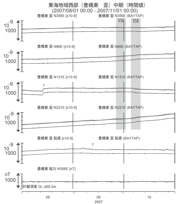
第16図 東海地域西部(豊橋東)の歪等の観測結果 (2007年8月～2007年10月)
