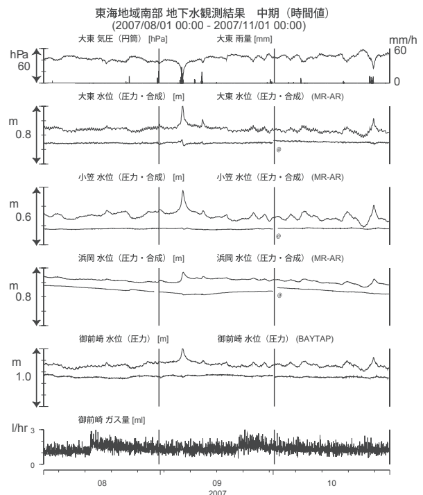
第8図 東海地域南部の地下水等の観測結果(2007年8月～2007年10月) Fig.8 Observed groundwater levels and others in the southern Tokai district from Aug. 2007 to Oct. 2007.
