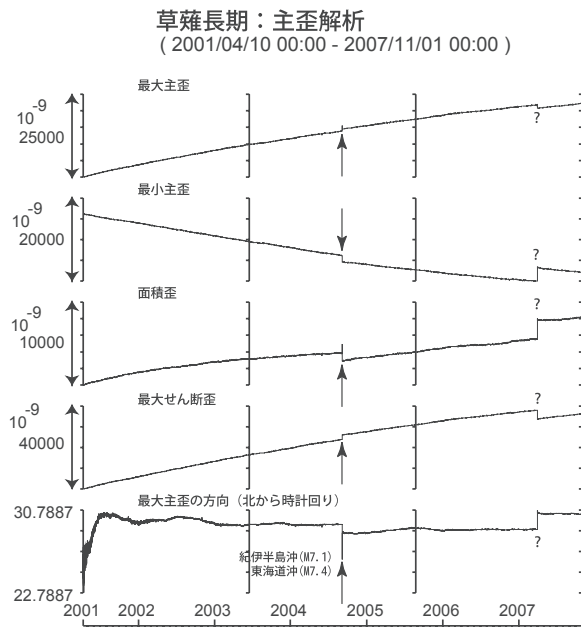
第31図 草薙における主歪解析の結果(2001年4月～2007年10月) Fig.31 Result of the principal strain analysis at the Kusanagi observation well from Apr. 2001 to Oct. 2007.
