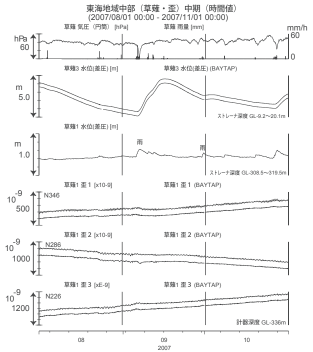
第6図 草薙観測井の地下水・歪の観測結果(2007年8月～2007年10月) Fig.6 Observed groundwater levels and strain at the Kusanagi observation site from Aug. 2007 to Oct. 2007.
