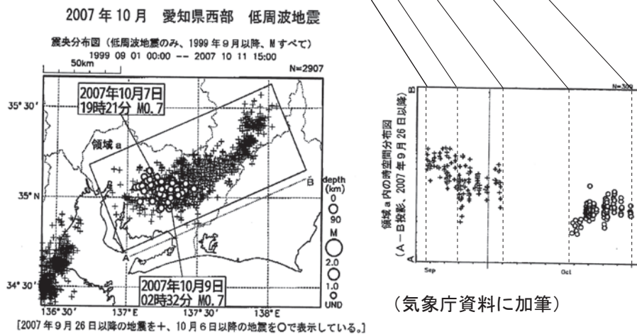
第 33 図 2007 年 9-10 月愛知県での低周波地震活動・短期的スロースリップに伴う豊橋東観測井の地殻歪変化 Fig.33 Strain change at the Toyohashi-higashi observation well induced by the non-volcanic tremors and the transient slow slips occurred at Aichi Pref. from Sep.- Oct., 2007.
