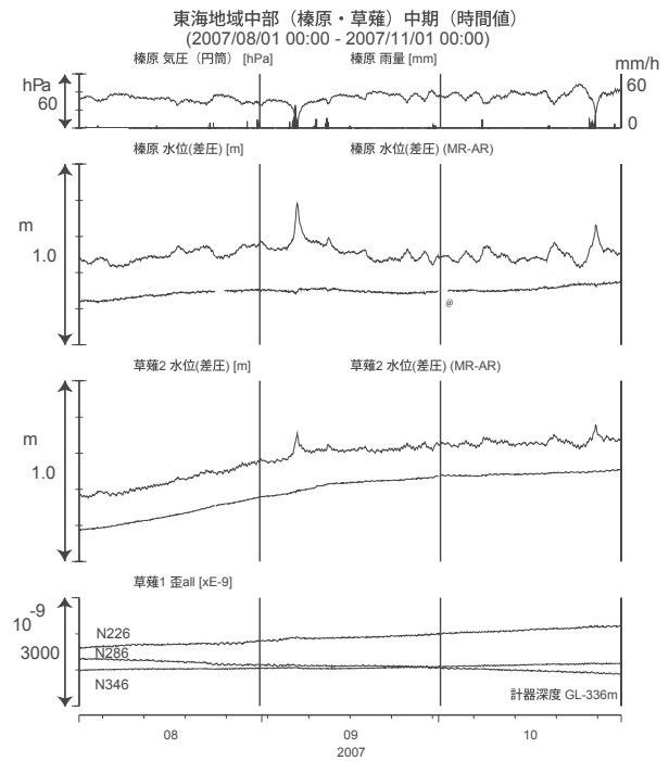
第4図 東海地域中部の地下水等の観測結果(2007年8月～2007年10月)
