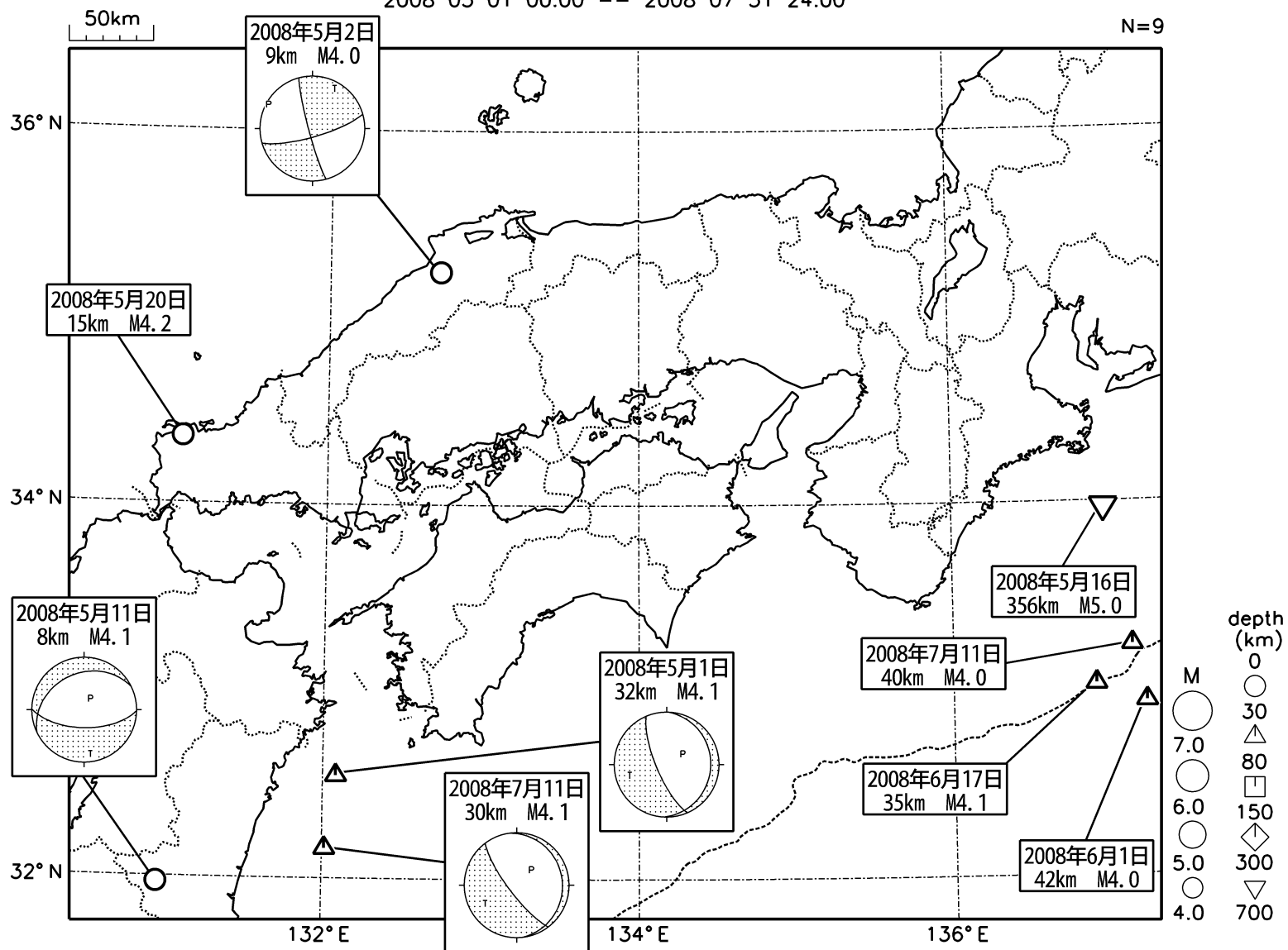
第1図(a) 近畿・中国・四国地方とその周辺の地震活動 (2008年5月~7月, M \geq 4.0 , 深さ \leq 700 km)
