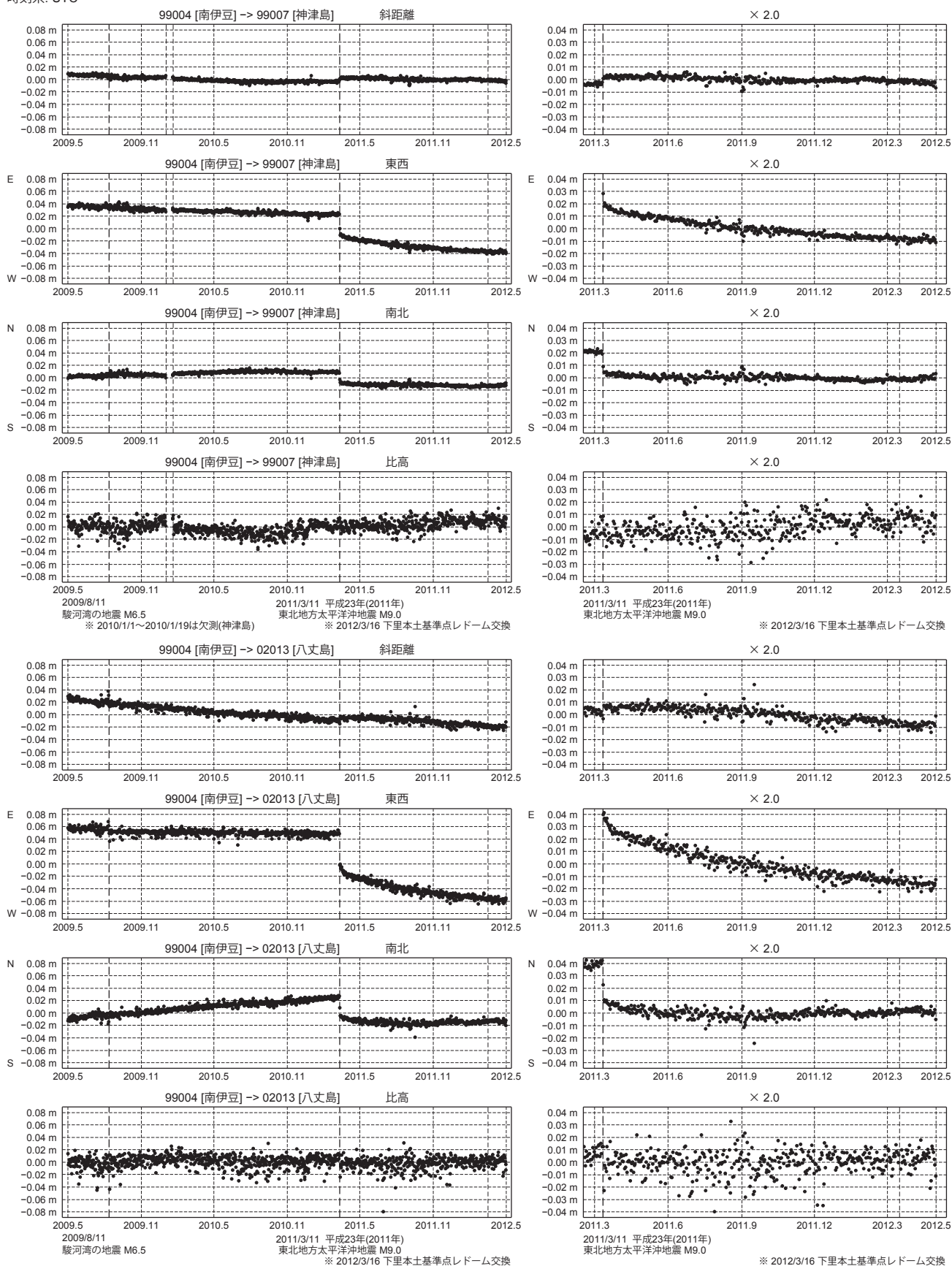
第4図 神津島および八丈島のGPS連続観測結果 (2009/5/1 ~ 2012/4/30)
