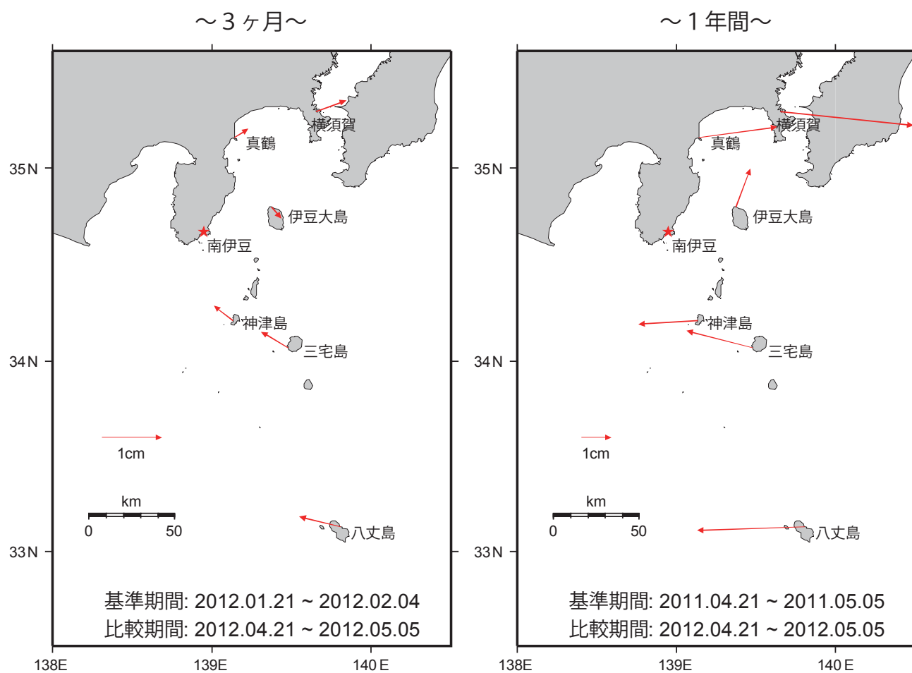
第1図 伊豆諸島海域 GPS 測点及び水平変動ベクトル図 (★固定局: 南伊豆) Fig.1 Locations and horizontal displacements at GPS stations in the Izu Islands. (★: Reference station Minami Izu)
