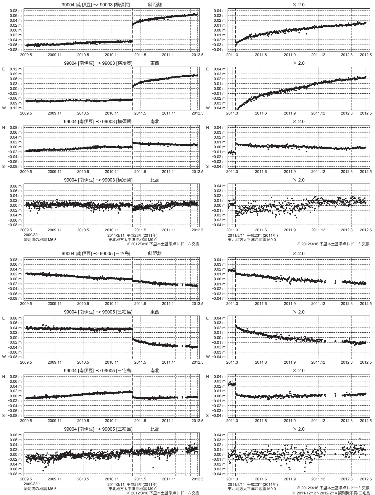
第3図 横須賀および三宅島の GPS 連続観測結果 (2009/5/1 ~ 2012/4/30)
