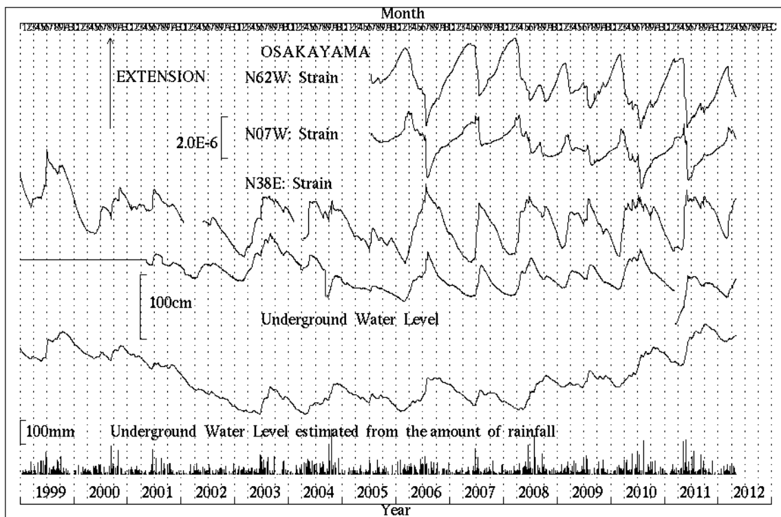
第5図 b 逢坂山観測所における歪変化と日雨量 (1999 年 1 月～2012 年 4 月) Fig.5b Strain change, underground water level, daily precipitation and estimated underground water level from precipitation at Osakayama observatory. (Jan.01,1999～Apr.30,2012).
