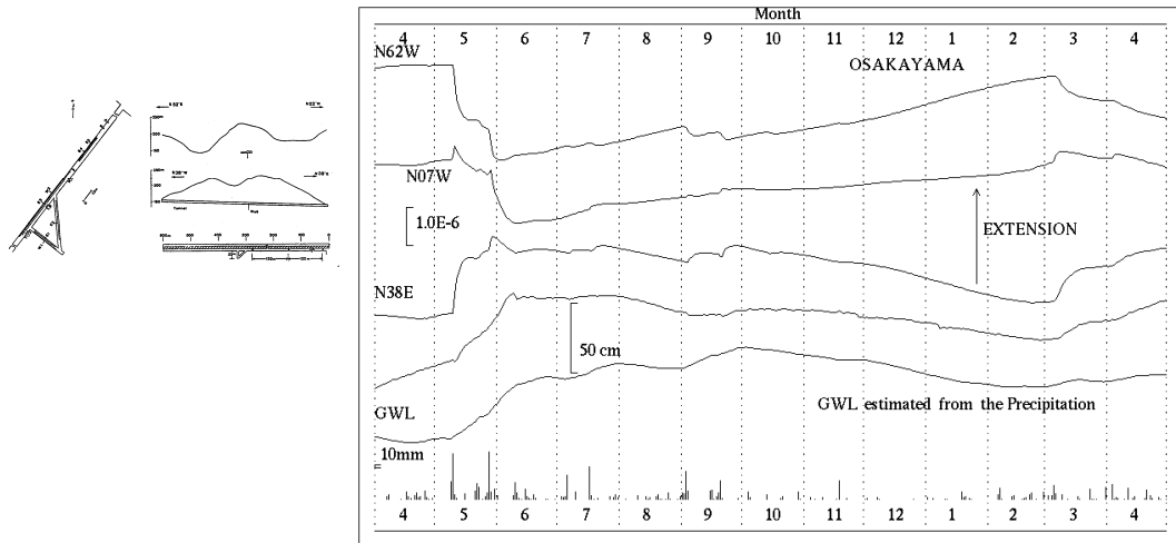
第5図 a 逢坂山観測所における歪変化と日雨量 (2011 年 4 月～2012 年 4 月) Fig.5a Strain change, underground water level and daily precipitation at Osakayama observatory. (Apr.01,2011～Apr.30,2012).
