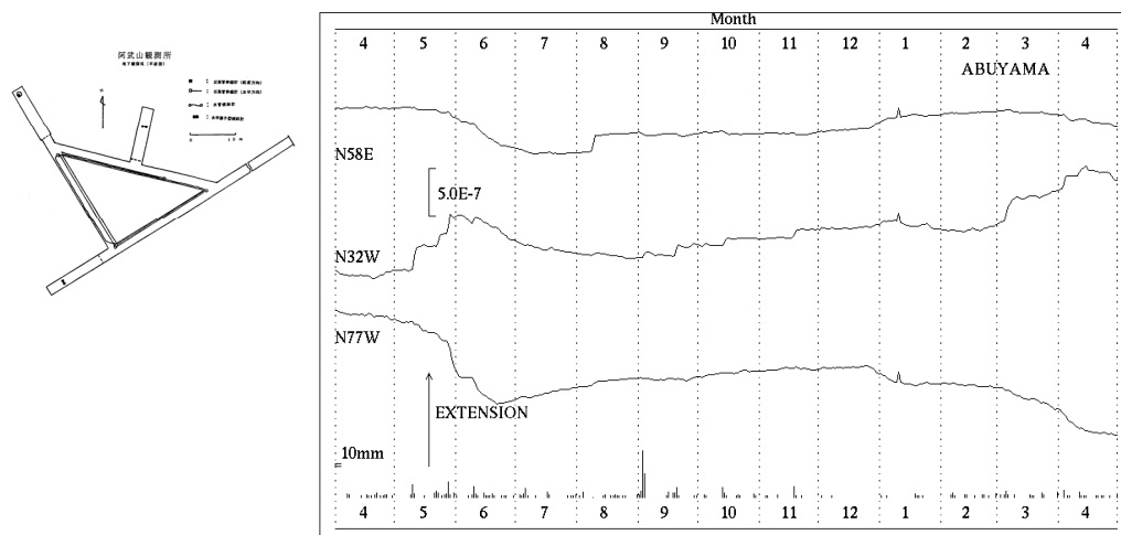
第3図 a 阿武山観測所における歪変化と日雨量（2011年4月～2012年4月） Fig.3a Strain changes and daily precipitation at Abuyama observatory. (Apr.01,2011～Apr.30,2012).
