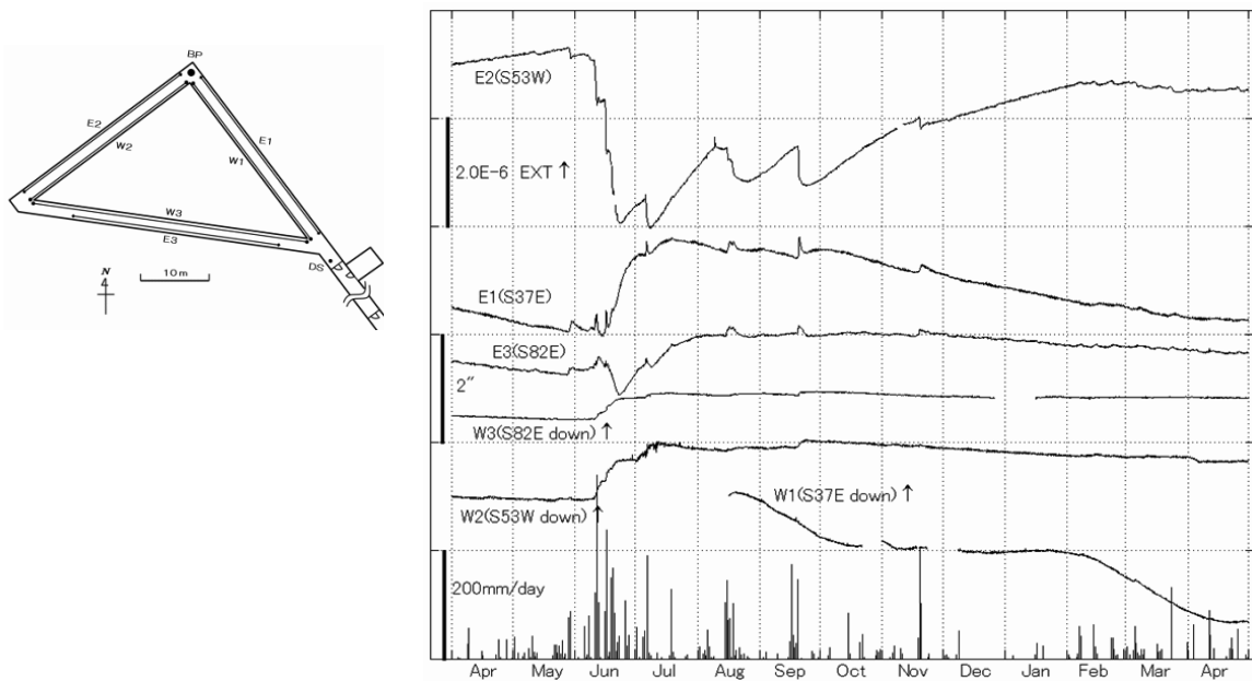
第 7 図 伊佐観測所における歪・傾斜変化と日雨量（2011 年 4 月～2012 年 4 月） Fig. 7 Strain changes, tilt changes and daily precipitation at Isa station. (Apr.01,2011～Apr.30,2012).
