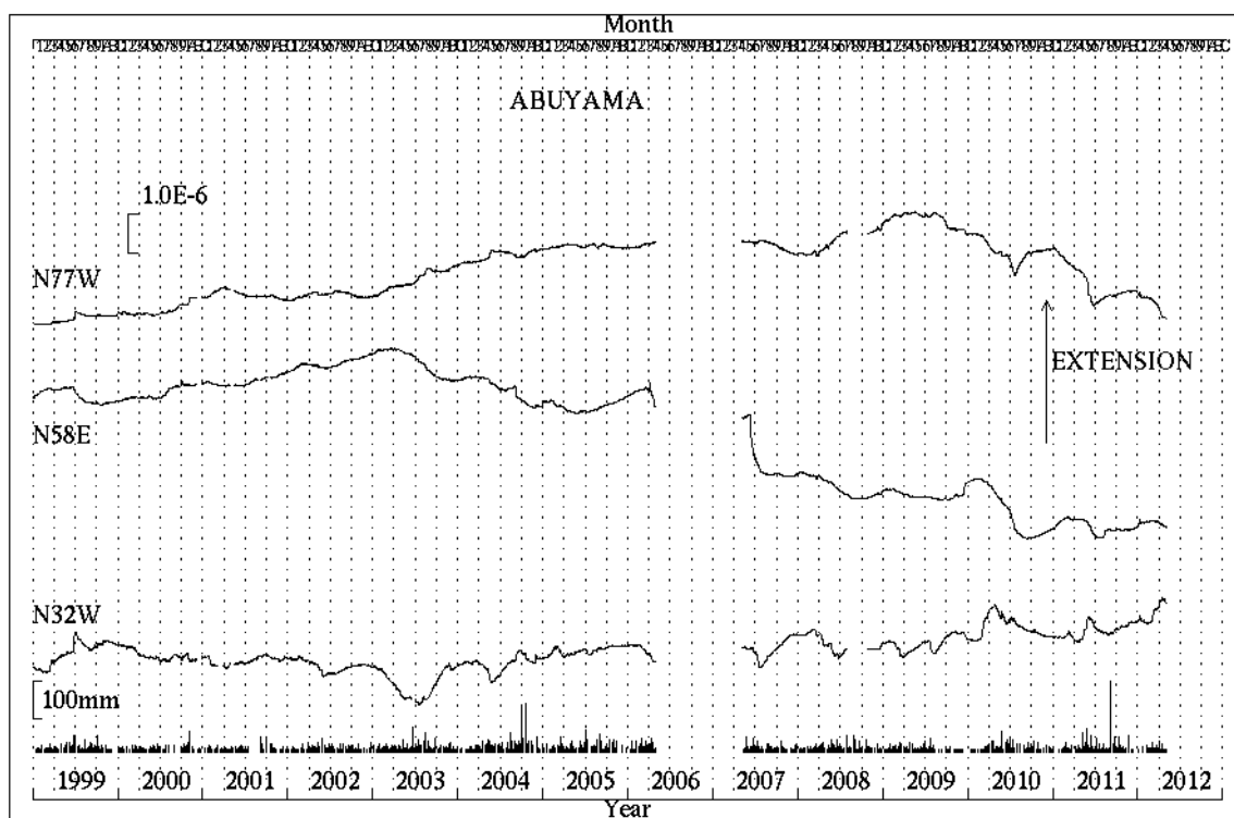
第3図 b 阿武山観測所における歪変化と日雨量（1999年1月～2012年4月） Fig.3b Strain changes and daily precipitation at Abuyama observatory. (Jan.01,1999～Apr.30,2012).
