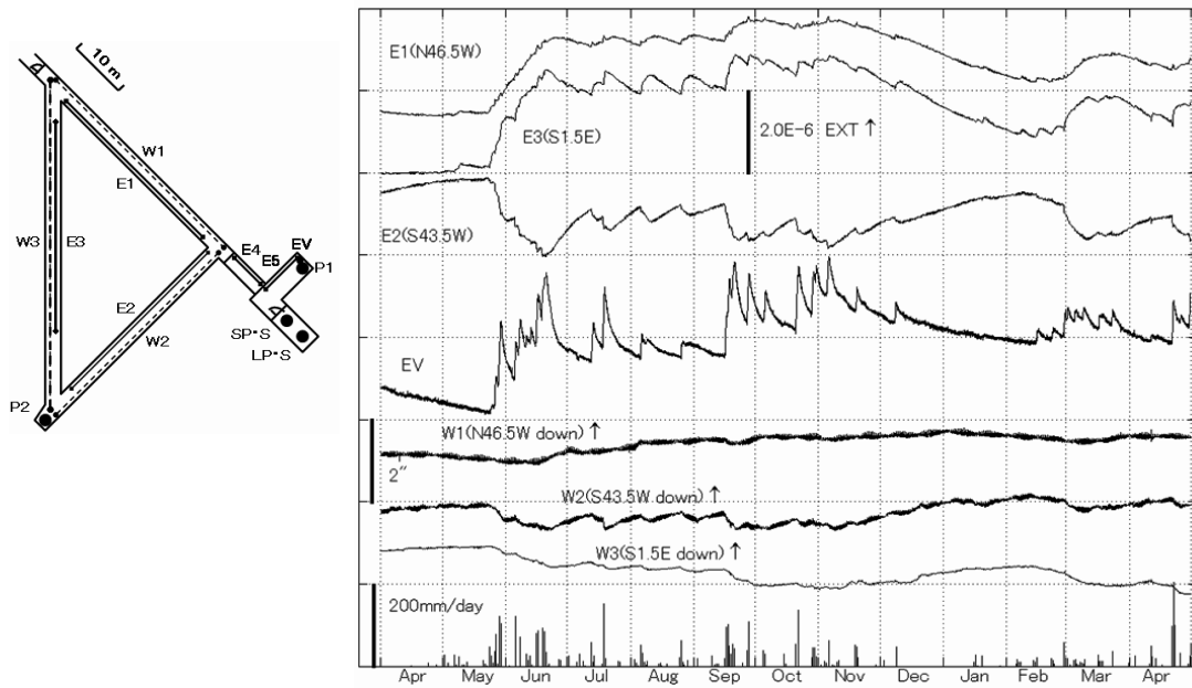
第 6 図 宮崎観測所における歪・傾斜変化と日雨量（2011 年 4 月～2012 年 4 月） Fig.6 Strain changes, tilt changes and daily precipitation at Miyazaki observatory. (Apr.01,2011～Apr.30,2012).
