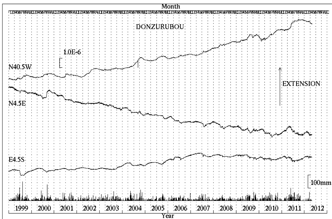
第4図 b 屯鶴峯観測所における歪変化と日雨量（1999年1月～2012年4月） Fig.4b Strain changes and daily precipitation at Donzurubo observatory. (Jan.01,1999～Apr.30,2012).
