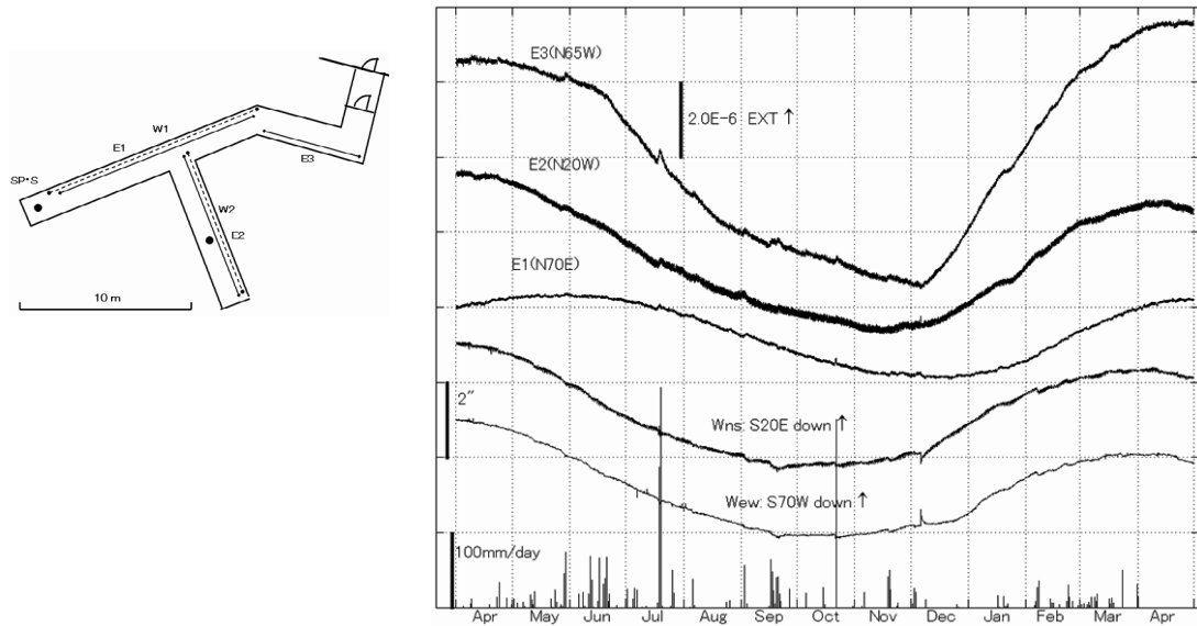
第 8 図 宿毛観測所における歪変化と日雨量 (2011 年 4 月～2012 年 4 月) Fig.8 Strain changes, tilt changes and daily precipitation at Sukumo station. (Apr.01,2011～Apr.30,2012).
