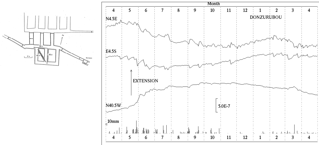
第4図 a 屯鶴峯観測所における歪変化と日雨量（2011年4月～2012年4月） Fig.4a Strain changes and daily precipitation at Donzurubo observatory. (Apr.01,2011～Apr.30,2012).
