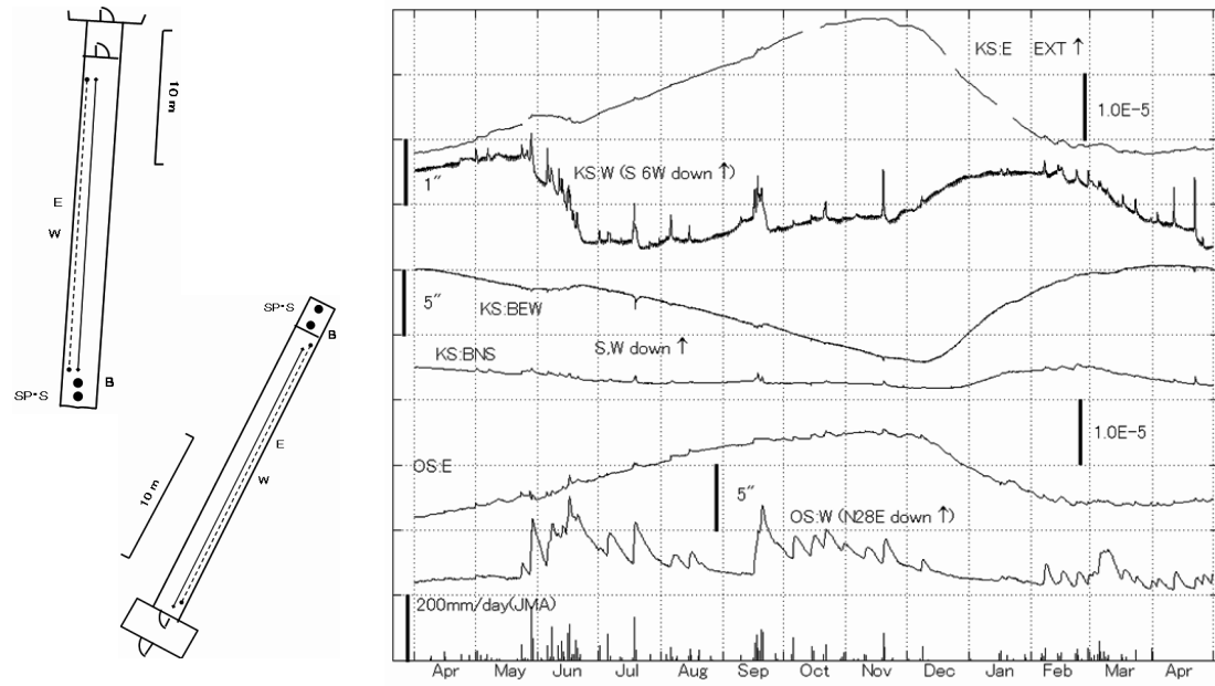
第 10 図 串間・大隈観測所における歪・傾斜変化 (2011 年 4 月～2012 年 4 月) Fig.10 Strain changes and tilt changes at Kushima, and Ohsumi station. Lowest bar graph is daily precipitation at Tashiro, nearest station by JMA. (Apr.01,2011～Apr.30,2012).
