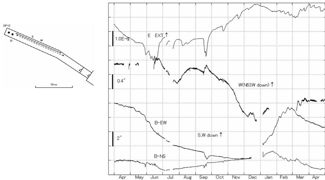
第 9 図 高城観測所における歪変化と傾斜変化 (2011 年 4 月～2012 年 4 月) Fig.9 Strain changes and tilt changes at Takajo station. (Apr.01,2011～Apr.30,2012).
