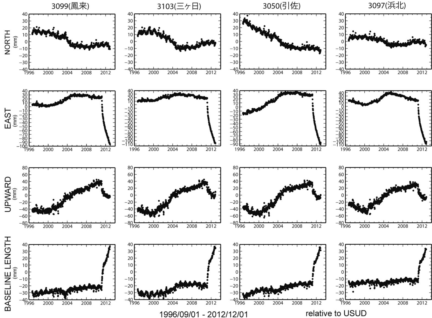
第4図 浜名湖周辺の GEONET の4観測点の、IGS白田観測点を基準とした南北成分・東西成分・上下成分・基線長の1996年9月1日から2012年12月1日までの時間変動。
