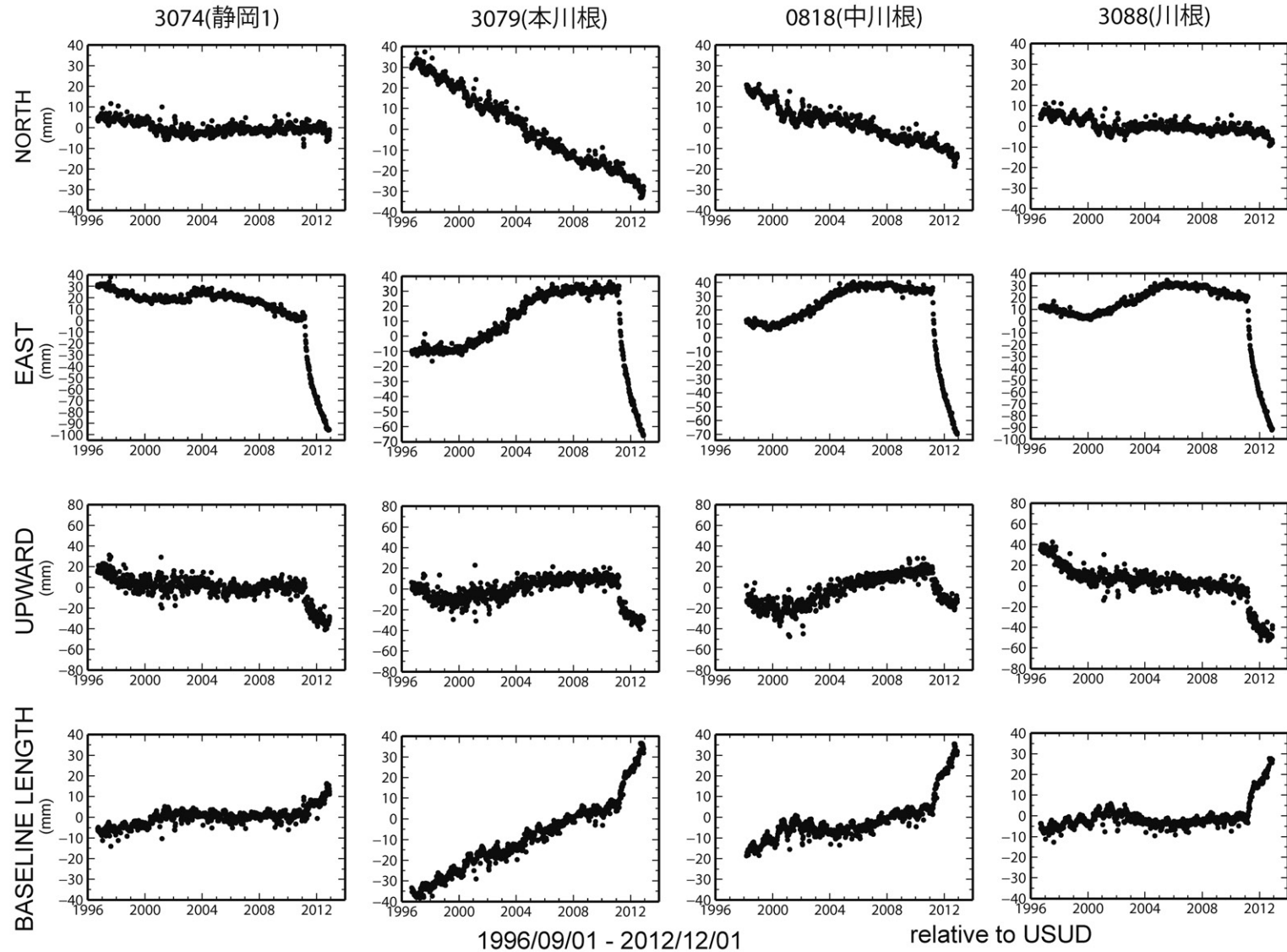
第2図 東海地震のヒンジライン想定域近傍東側の4観測点の、IGS白田観測点を基準とした南北成分・東西成分・上下成分・基線長の1996年9月1日から2012年12月1日までの時間変動。 Fig. 2 Time variations of N-S, E-W, U-D components and baseline length of the eastern four GPS sites near the hinge line of hypothesized Tokai earthquake relative to the USUD site.
