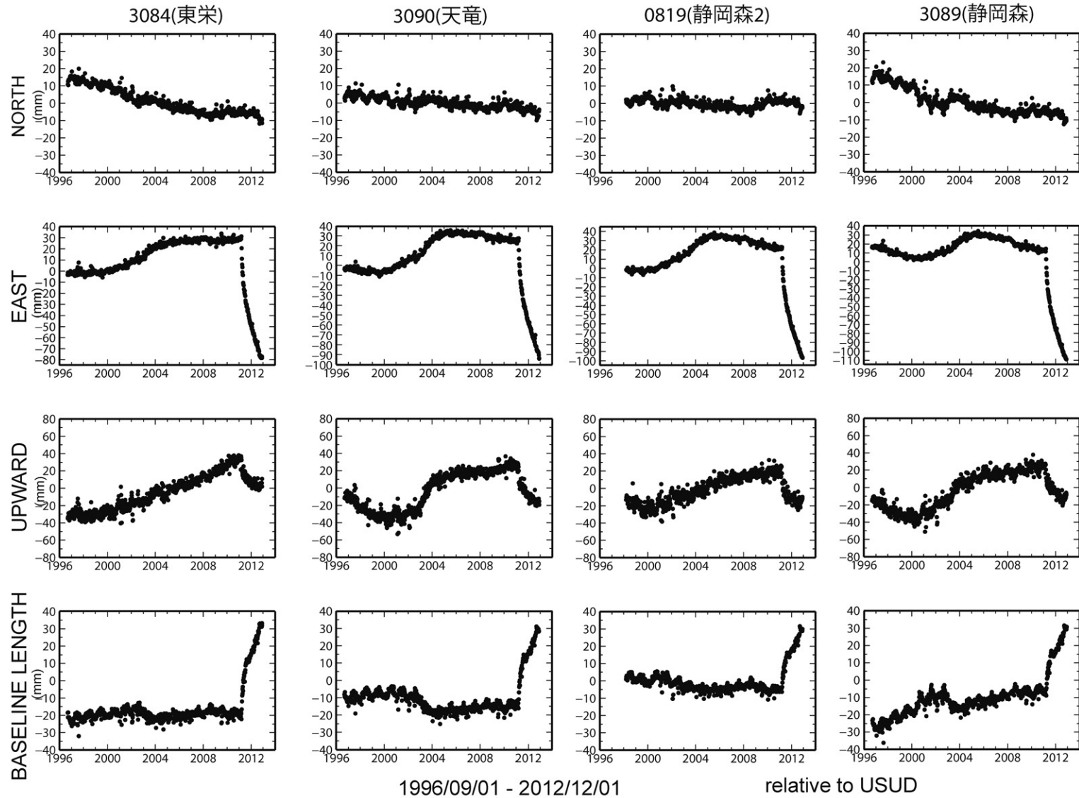
第3図 東海地震のヒンジライン想定域近傍西側の4観測点の、IGS白田観測点を基準とした南北成分・東西成分・上下成分・基線長の1996年9月1日から2012年12月1日までの時間変動。
