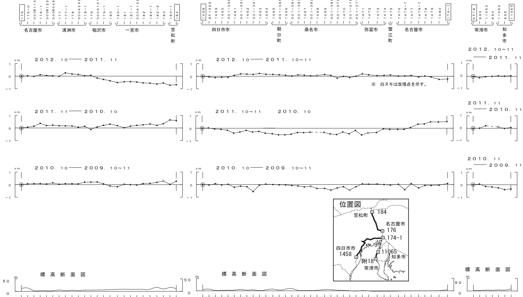
第1図 中京の上下変動
