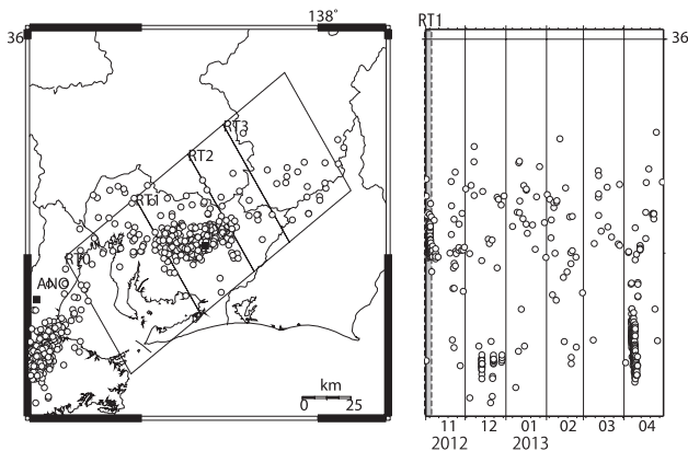
第35図 東海地方における低周波微動の震央分布と時空間分布(2012年11月～2013年4月)
