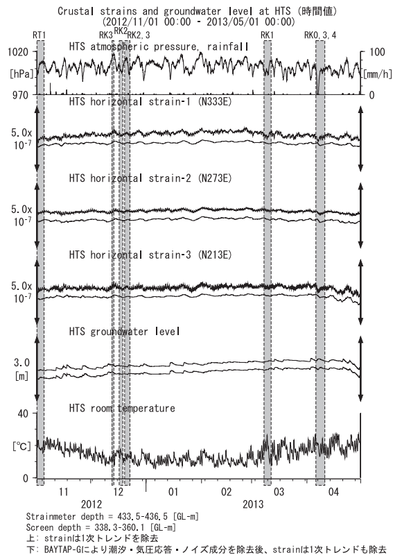
第6図 HTSにおける歪・地下水位観測結果 (2012年11月～2013年4月)
