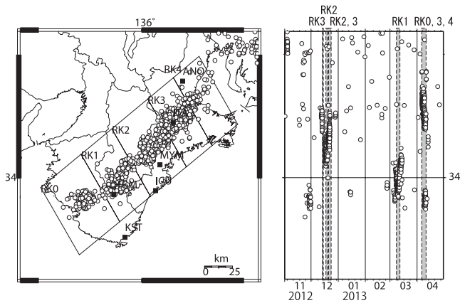
第37図 紀伊半島における低周波微動の震央分布と時空間分布(2012年11月～2013年4月)
