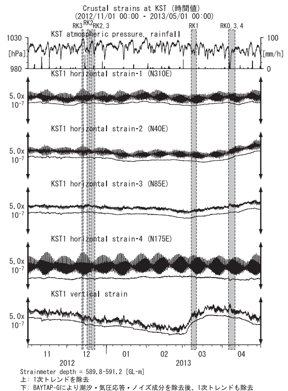
第17図 KSTにおける歪観測結果 (2012年11月～2013年4月) Fig.17 Observed strains at the KST observation site from November 2012 to April 2013.
