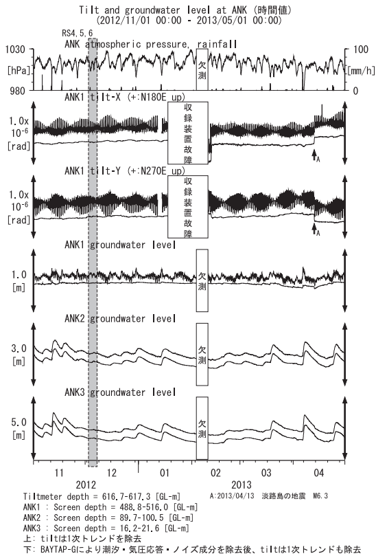
第22図 ANKにおける傾斜・地下水位観測結果 (2012年11月～2013年4月) Fig.22 Observed tilts and groundwater levels at the ANK observation site from November 2012 to April 2013.
