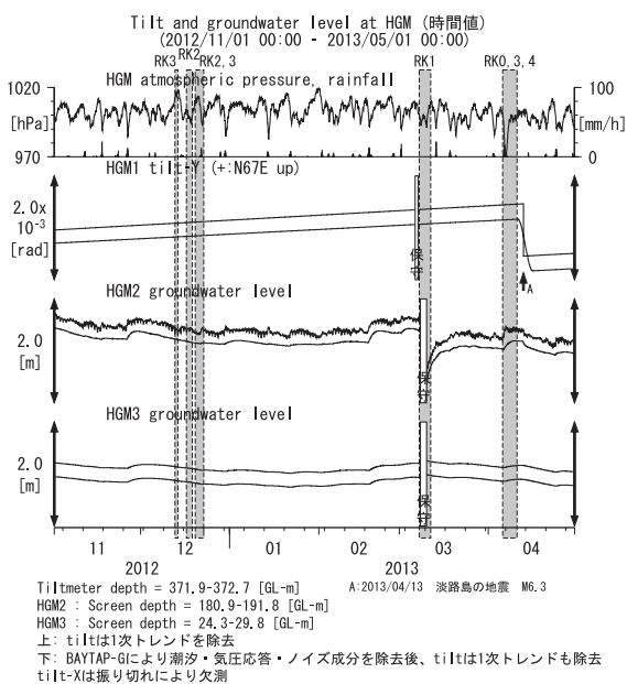
第16図 HGMにおける傾斜・地下水位観測結果 (2012年11月～2013年4月) Fig.16 Observed tilt and groundwater levels at the HGM observation site from November 2012 to April 2013.
