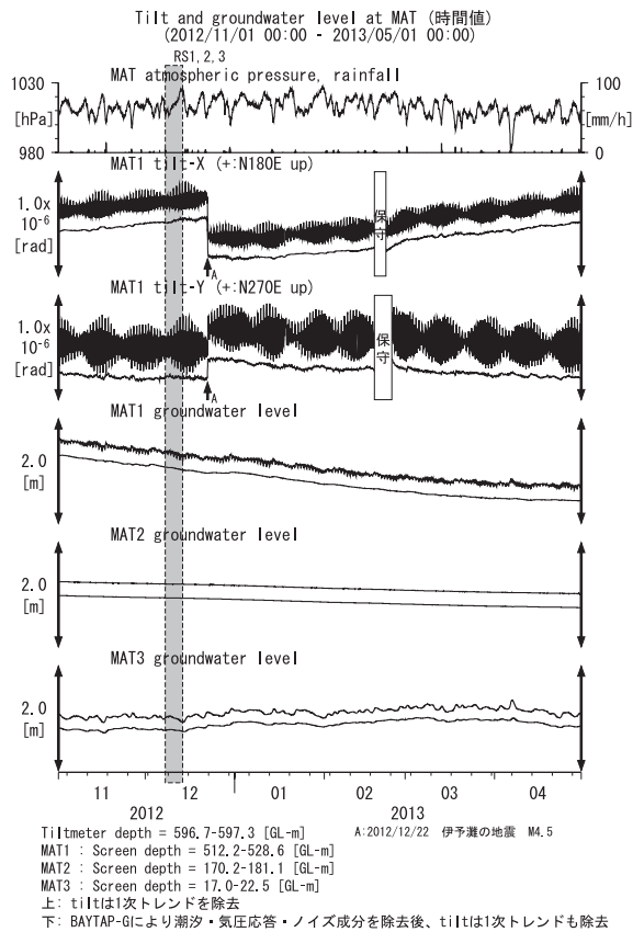
第34図 MATにおける傾斜・地下水位観測結果 (2012年11月～2013年4月)
