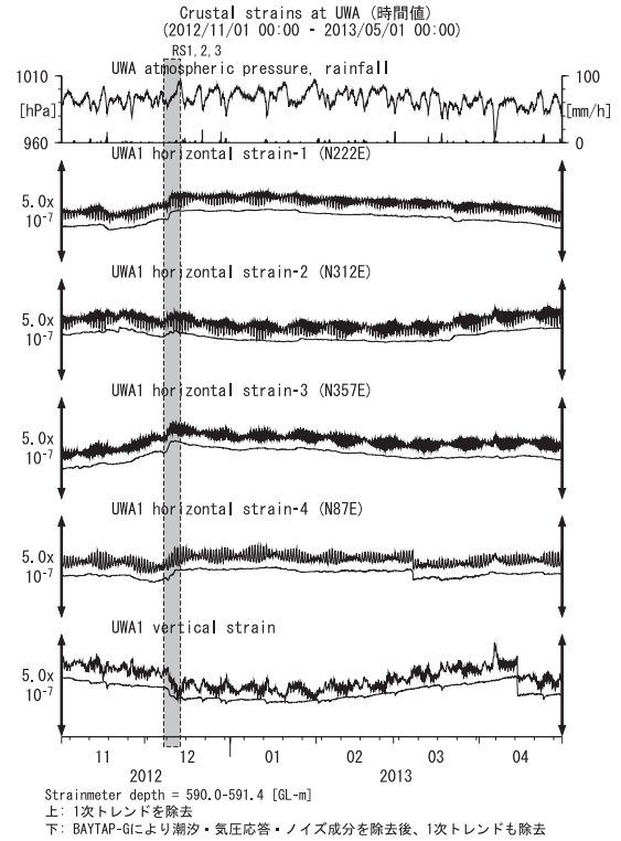
第31図 UWAにおける歪観測結果 (2012年11月～2013年4月) Fig.31 Observed strains at the UWA observation site from November 2012 to April 2013.
