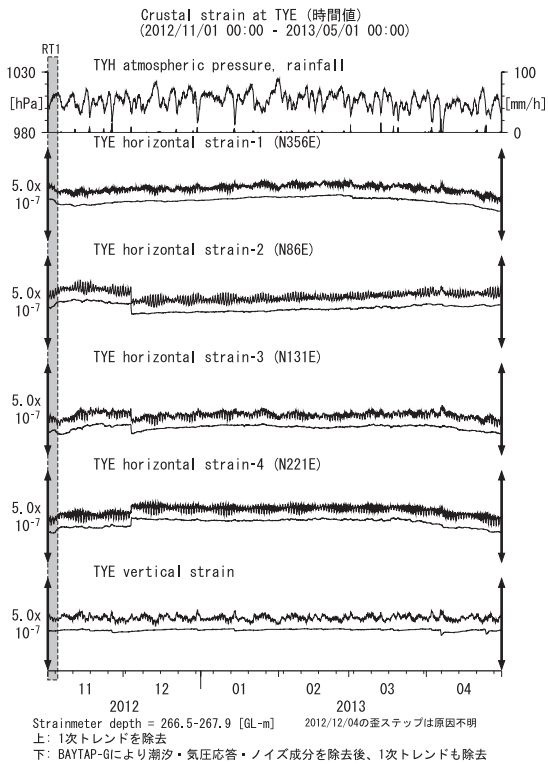
第4図 TYEにおける歪観測結果 (2012年11月～2013年4月) Fig.4 Observed strains at the TYE observation site from November 2012 to April 2013.
