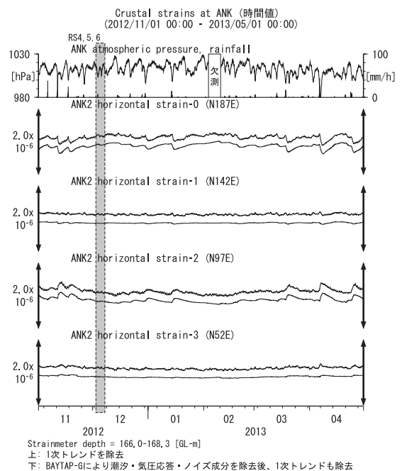
第21図 ANKにおける歪観測結果 (2012年11月～2013年4月) Fig.21 Observed strains at the ANK observation site from November 2012 to April 2013.
