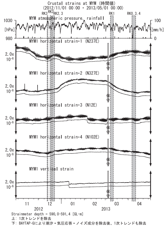
第11図 MYMにおける歪観測結果 (2012年11月～2013年4月) Fig.11 Observed strains at the MYM observation site from November 2012 to April 2013.
