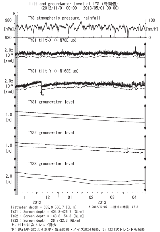
第3図 TYSにおける傾斜・地下水位観測結果 (2012年11月～2013年4月) Fig.3 Observed tilts and groundwater levels at the TYS observation site from November 2012 to April 2013.
