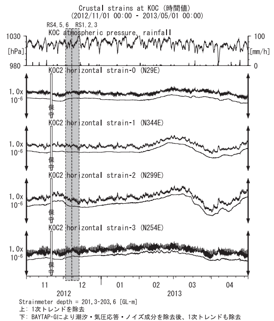
第25図 KOCにおける歪観測結果 (2012年11月～2013年4月) Fig.25 Observed strains at the KOC observation site from November 2012 to April 2013.
