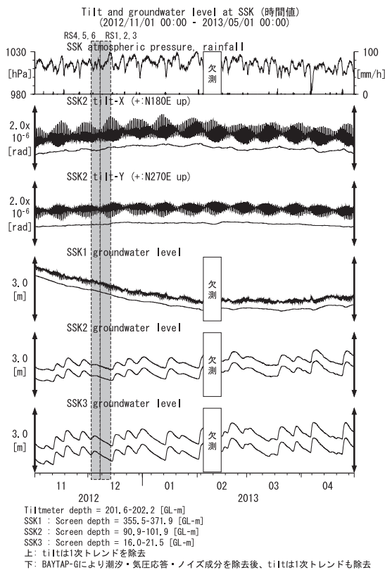
第28図 SSKにおける傾斜・地下水位観測結果 (2012年11月～2013年4月) Fig.28 Observed tilts and groundwater levels at the SSK observation site from November 2012 to April 2013.
