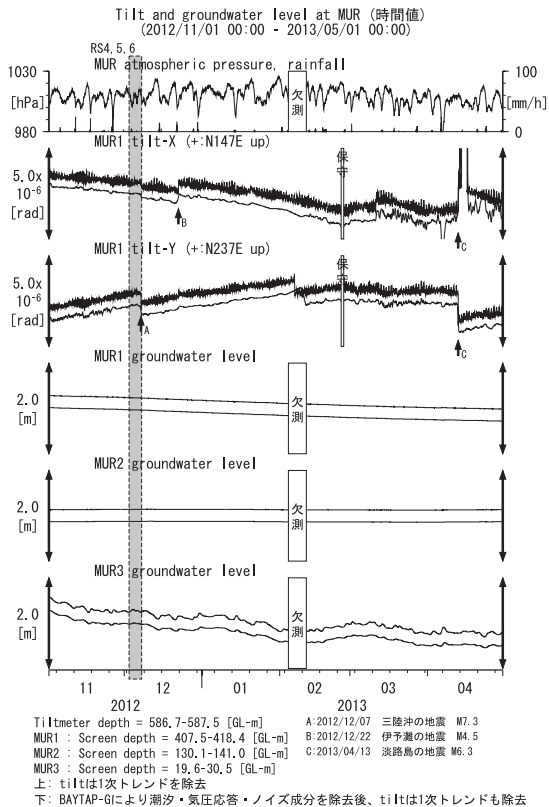
第24図 MURにおける傾斜・地下水位観測結果 (2012年11月～2013年4月) Fig.24 Observed tilts and groundwater levels at the MUR observation site from November 2012 to April 2013.
