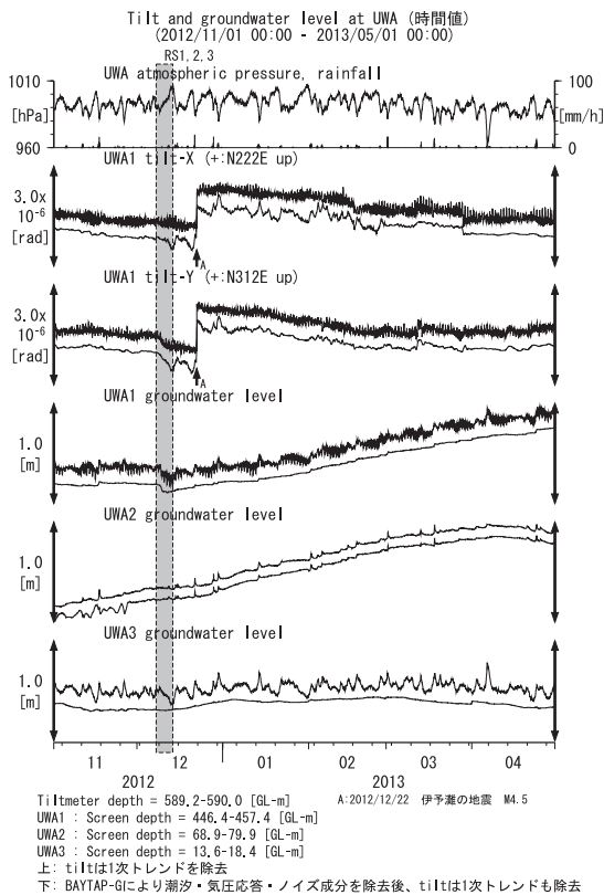
第32図 UWAにおける傾斜・地下水位観測結果 (2012年11月～2013年4月) Fig.32 Observed tilts and groundwater levels at the UWA observation site from November 2012 to April 2013.
