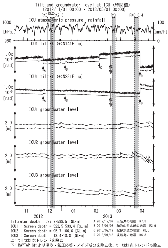
第14図 ICUにおける傾斜・地下水位観測結果 (2012年11月～2013年4月) Fig.14 Observed tilts and groundwater levels at the ICU observation site from November 2012 to April 2013.
