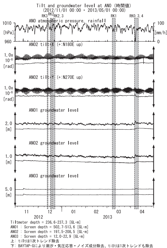
第8図 ANOにおける傾斜・地下水位観測結果 (2012年11月～2013年4月)
