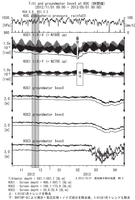
第26図 KOCにおける傾斜・地下水位観測結果 (2012年11月～2013年4月) Fig.26 Observed tilts and groundwater levels at the KOC observation site from November 2012 to April 2013.
