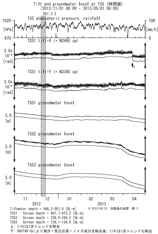
第30図 TSSにおける傾斜・地下水位観測結果 (2012年11月～2013年4月) Fig.30 Observed tilts and groundwater levels at the TSS observation site from November 2012 to April 2013.
