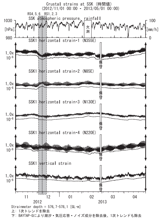
第27図 SSKにおける歪観測結果 (2012年11月～2013年4月) Fig.27 Observed strains at the SSK observation site from November 2012 to April 2013.
