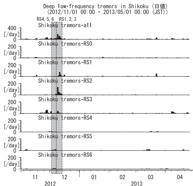
第40図 四国地方における低周波微動の発生個数(2012年11月～2013年4月)
