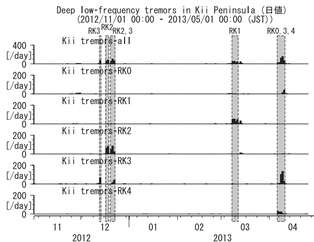
第38図 紀伊半島における低周波微動の発生個数(2012年11月～2013年4月)
