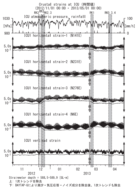
第13図 ICUにおける歪観測結果 (2012年11月～2013年4月) Fig.13 Observed strains at the ICU observation site from November 2012 to April 2013.
