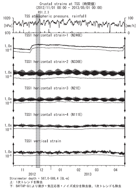
第29図 TSSにおける歪観測結果 (2012年11月～2013年4月) Fig.29 Observed strains at the TSS observation site from November 2012 to April 2013.
