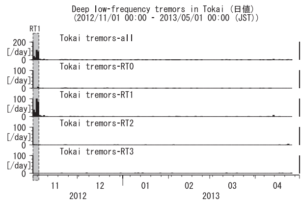
第36図 東海地方における低周波微動の発生個数(2012年11月～2013年4月)
