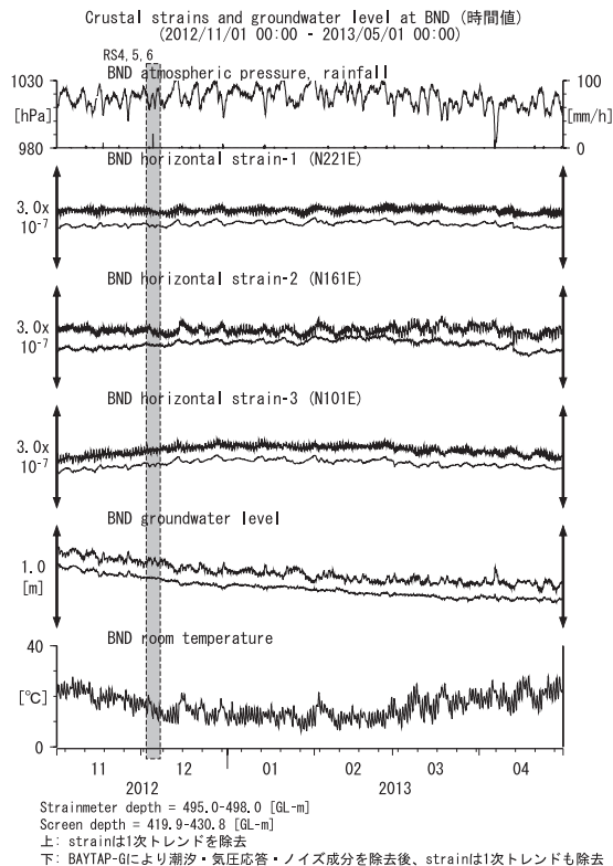
第20図 BNDにおける歪・地下水位観測結果 (2012年11月～2013年4月) Fig.20 Observed strains and groundwater levels at the BND observation site from November 2012 to April 2013.
