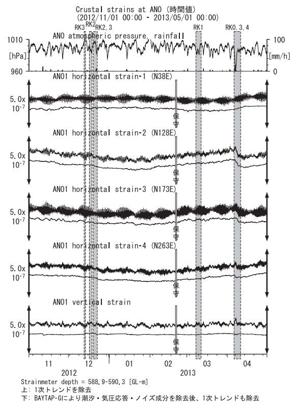
第7図 ANOにおける歪観測結果 (2012年11月～2013年4月)
