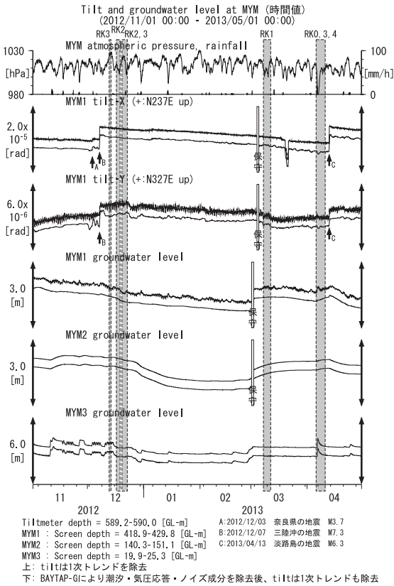
第12図 MYMにおける傾斜・地下水位観測結果 (2012年11月～2013年4月) Fig.12 Observed tilts and groundwater levels at the MYM observation site from November 2012 to April 2013.
