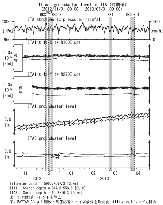
第10図 ITAにおける傾斜・地下水位観測結果 (2012年11月～2013年4月) Fig.10 Observed tilts and groundwater levels at the ITA observation site from November 2012 to April 2013.
