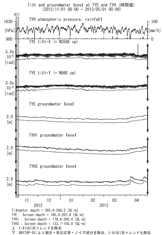
第5図 TYEおよびTYHにおける傾斜・地下水位観測結果 (2012年11月～2013年4月) Fig.5 Observed tilts and groundwater levels at the TYE and the TYH observation site from November 2012 to April 2013.
