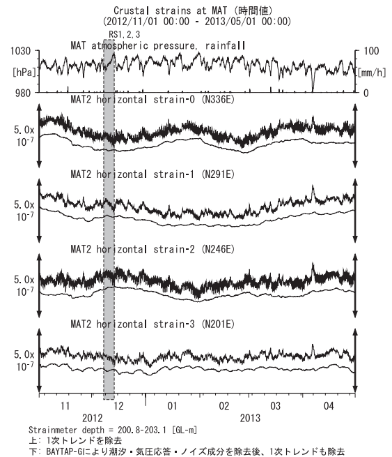
第33図 MATにおける歪観測結果 (2012年11月～2013年4月) Fig.33 Observed strains at the MAT observation site from November 2012 to April 2013.
