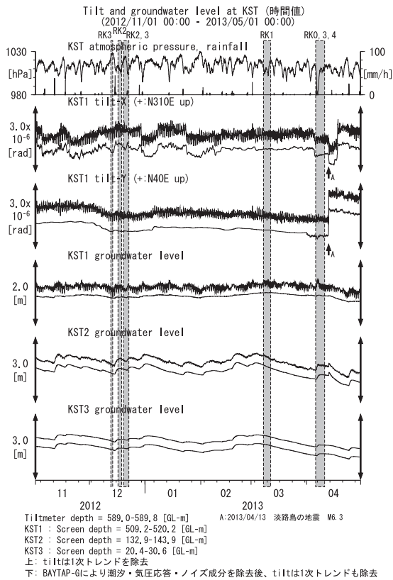
第18図 KSTにおける傾斜・地下水位観測結果 (2012年11月～2013年4月) Fig.18 Observed tilts and groundwater levels at the KST observation site from November 2012 to April 2013.
