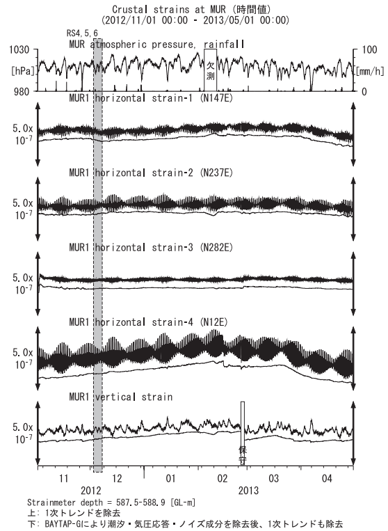
第23図 MURにおける歪観測結果 (2012年11月～2013年4月) Fig.23 Observed strains at the MUR observation site from November 2012 to April 2013.
