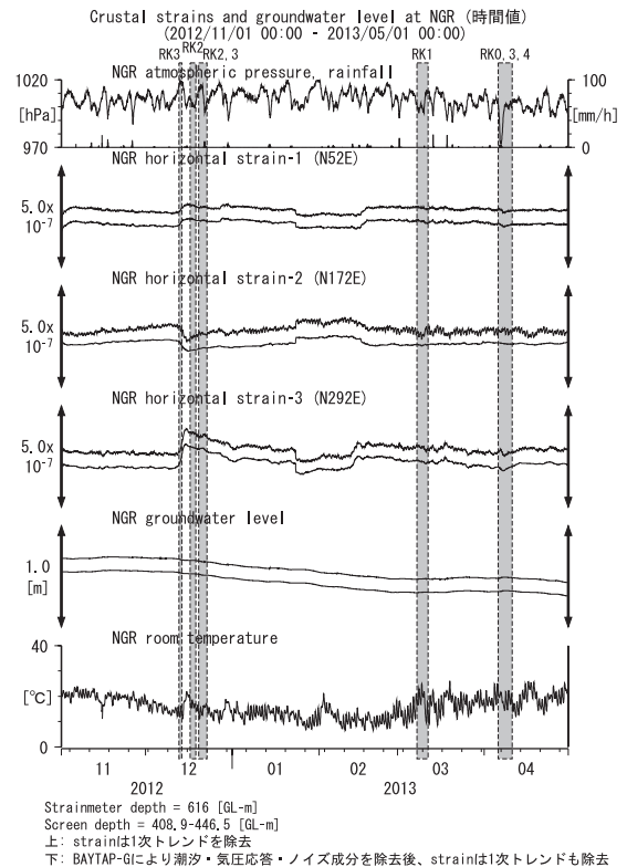
第19図 NGRにおける歪・地下水位観測結果 (2012年11月～2013年4月) Fig.19 Observed strains and groundwater levels at the NGR observation site from November 2012 to April 2013.
