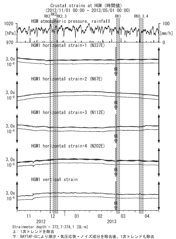
第15図 HGMにおける歪観測結果 (2012年11月～2013年4月) Fig.15 Observed strains at the HGM observation site from November 2012 to April 2013.
