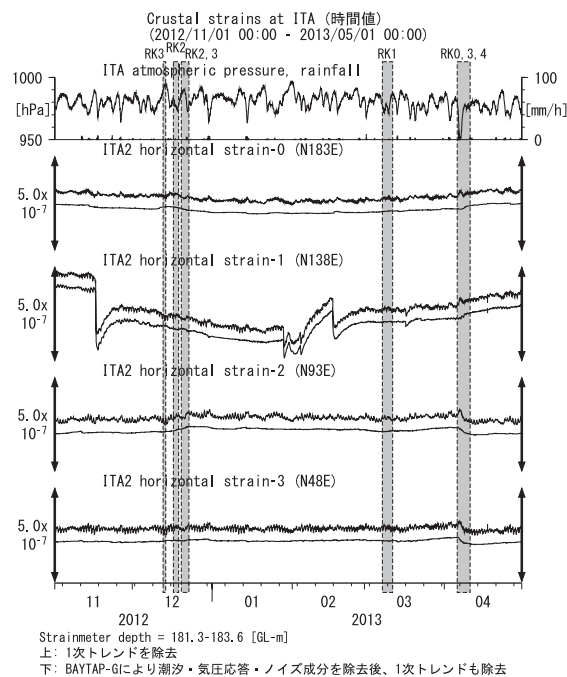
第9図 ITAにおける歪観測結果 (2012年11月～2013年4月)
