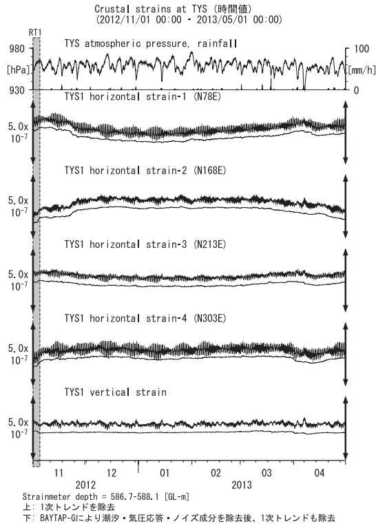
第2図 TYSにおける歪観測結果 (2012年11月～2013年4月) Fig.2 Observed strains at the TYS observation site from November 2012 to April 2013.
