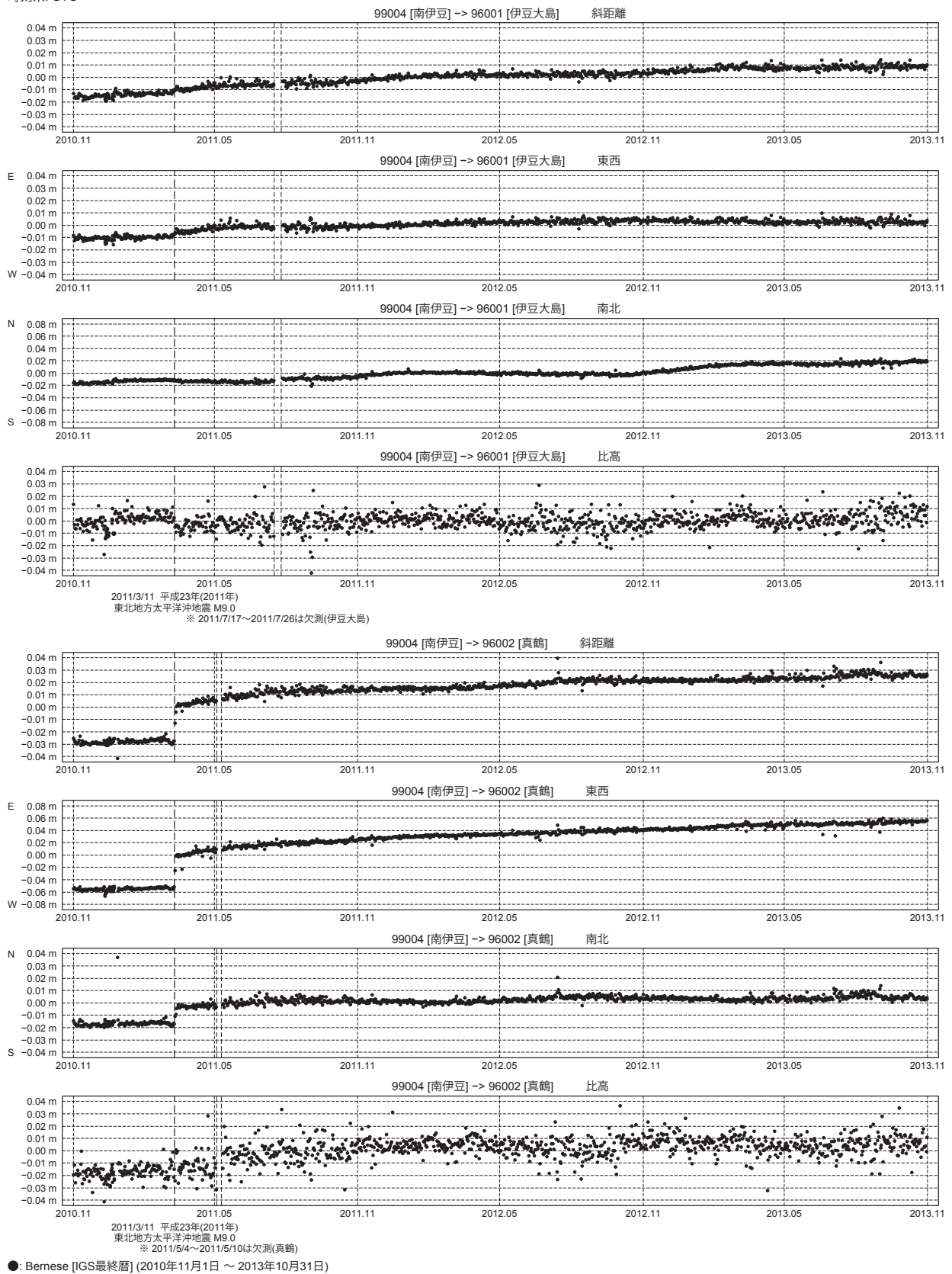
第2図 南伊豆基点での伊豆大島および真鶴のGPS連続観測結果 (2010/11/1~2013/10/31)
