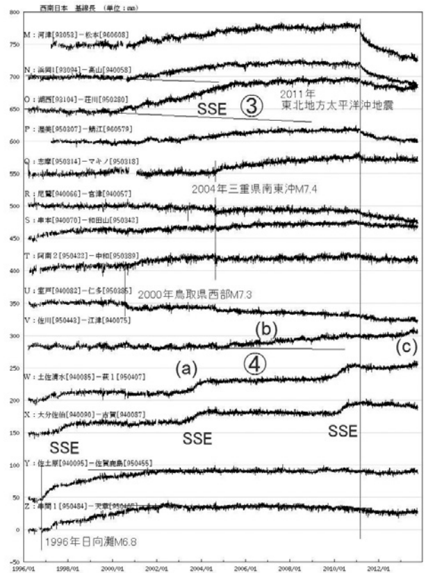
第2図(b) 基線長変化 (1996年から2013年10月). Fig. 2(b) Time series data of baseline length changes.
