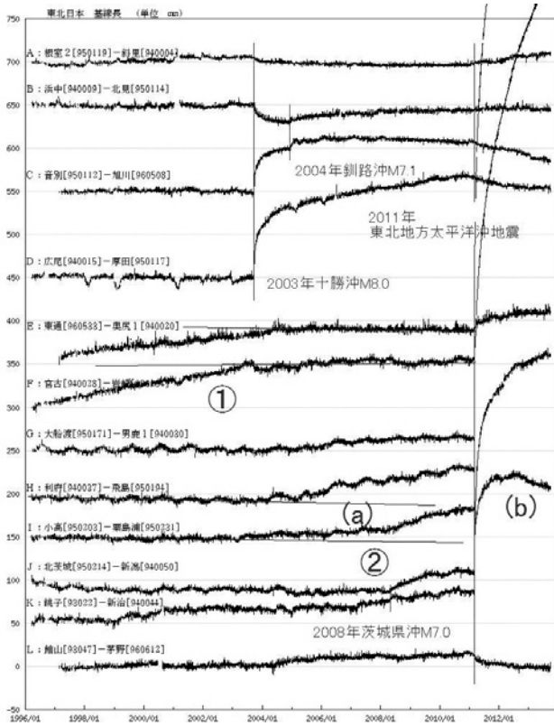
第2図(a) 基線長変化 (1996年から2013年10月). Fig. 2(a) Time series data of baseline length changes.
