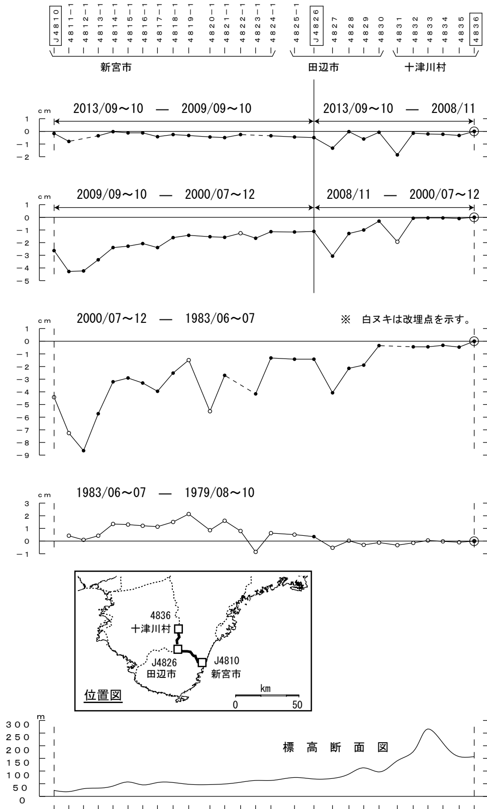
第1図 水準測量による新宮市～十津川村の上下変動
