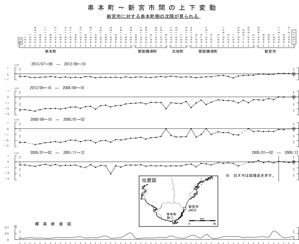
第 3 図 水準測量による串本町～新宮市の上下変動
