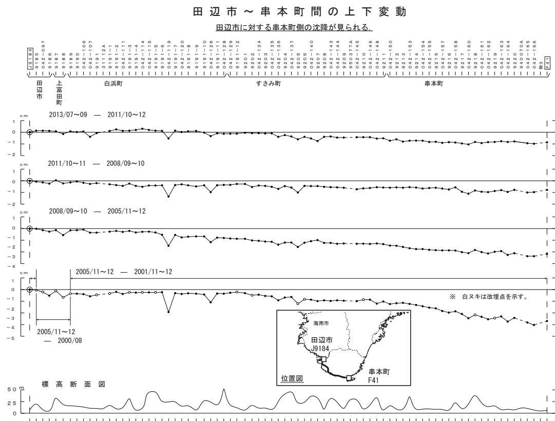
第 2 図 水準測量による田辺市～串本町の上下変動
