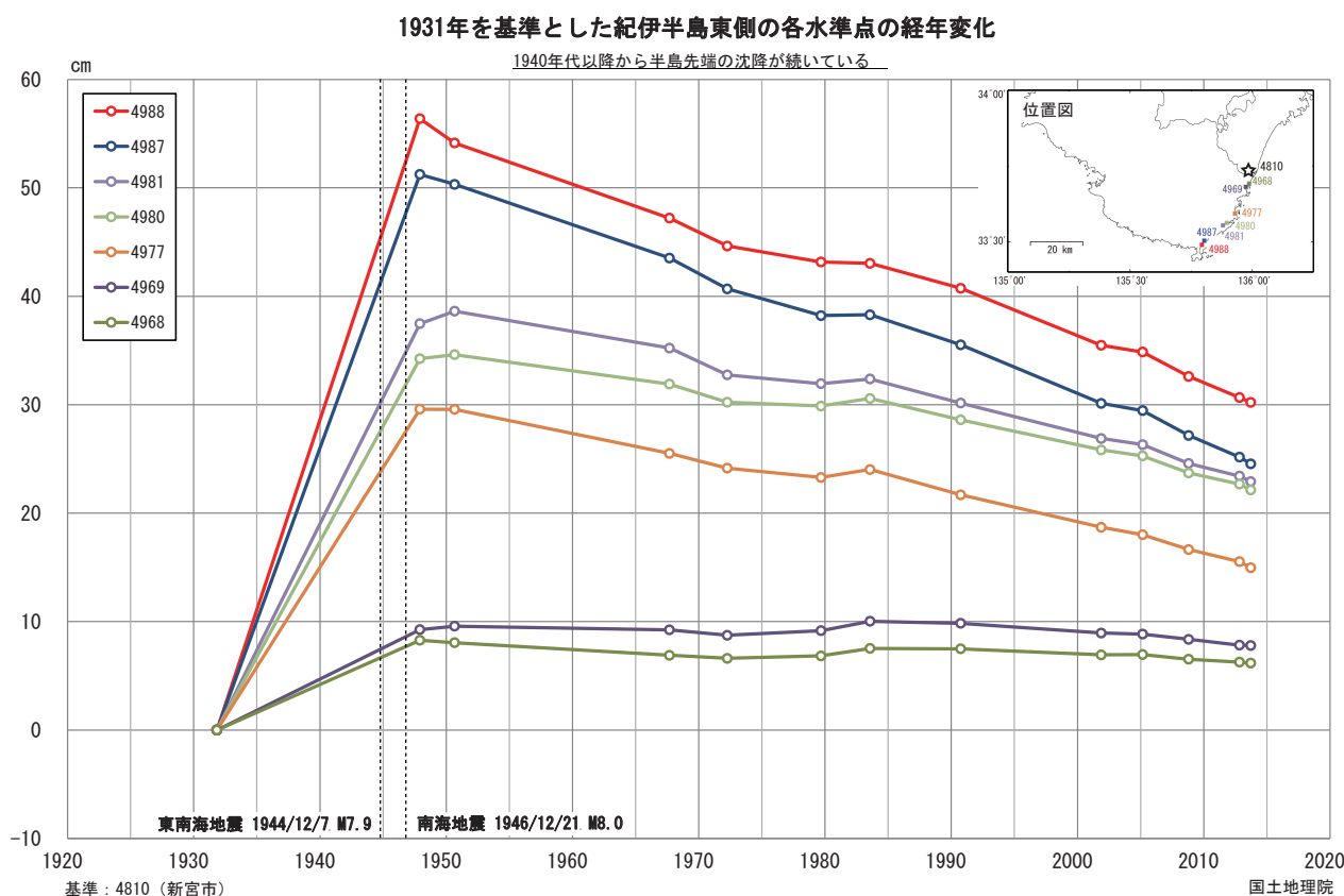
第5図 紀伊半島東側の水準点の上下変動経年変化 (1931年度基準・J4810 固定)
