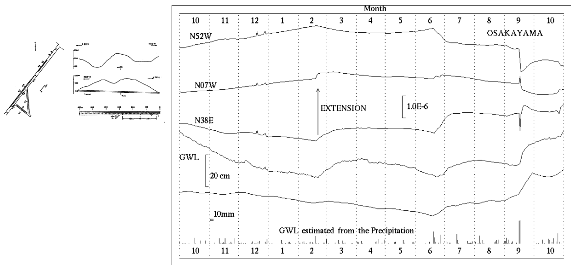
第5図 a 逢坂山観測所における歪変化と日雨量 (2012 年 10 月～2013 年 10 月) Fig.5a Strain change, underground water level and daily precipitation at Osakayama observatory. (Oct.01,2012～Oct.31,2013).
