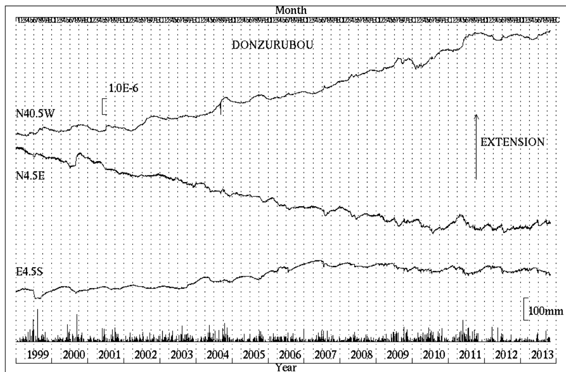
第4図 b 屯鶴峯観測所における歪変化と日雨量（1999年1月～2013年10月） Fig.4b Strain changes and daily precipitation at Donzurubo observatory. (Jan.01,1999～Oct.31,2013).
