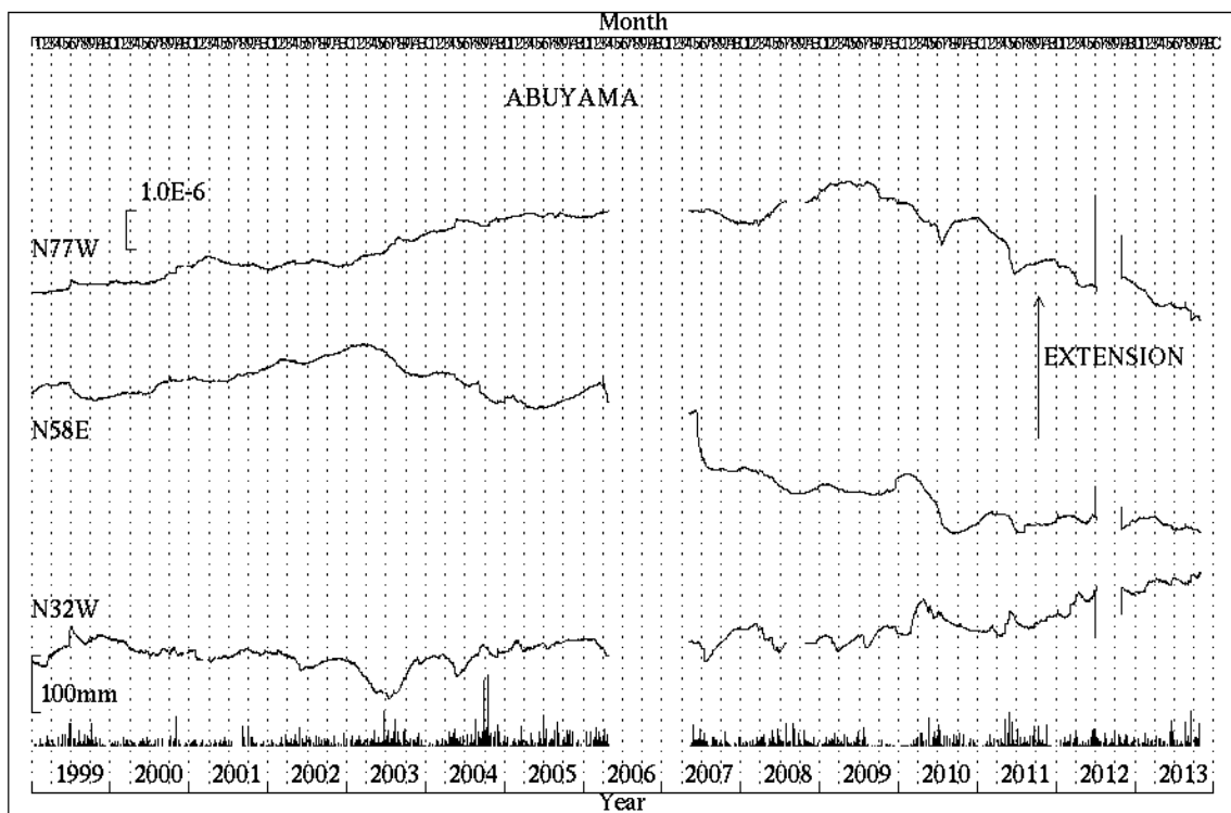
第3図 b 阿武山観測所における歪変化と日雨量（1999年1月～2013年10月） Fig.3b Strain changes and daily precipitation at Abuyama observatory. (Jan.01,1999～Oct.31,2013).
