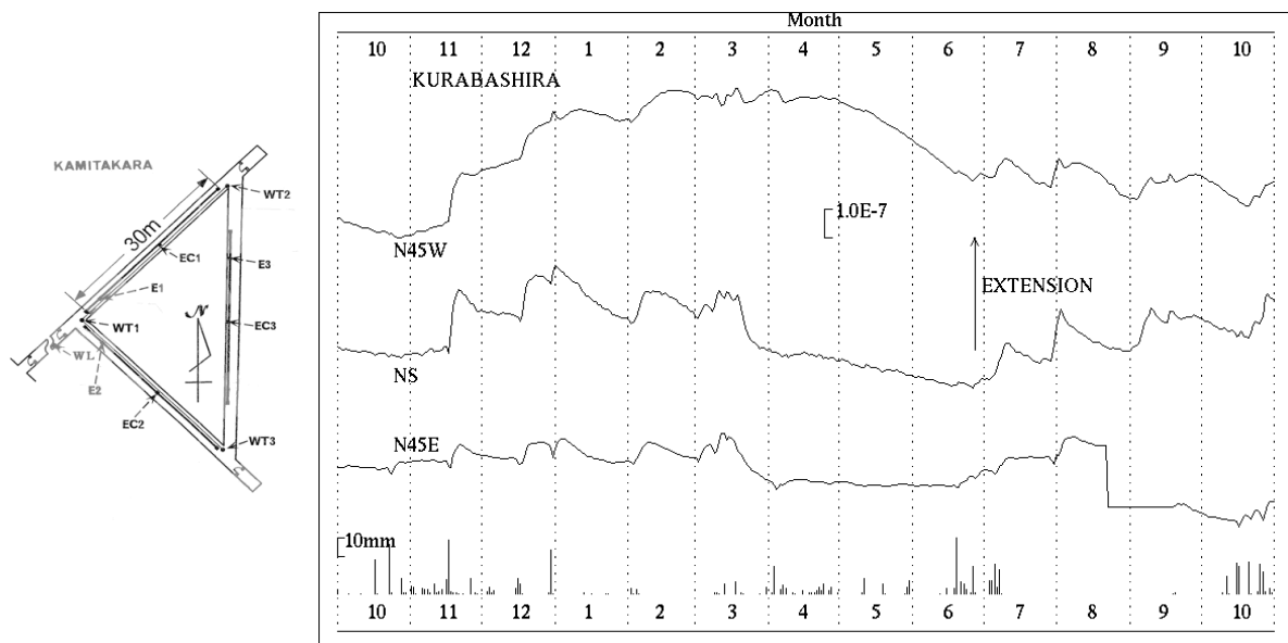
第 2 図 上宝観測所蔵柱観測室における歪変化と日雨量(2012 年 10 月～2013 年 10 月)
