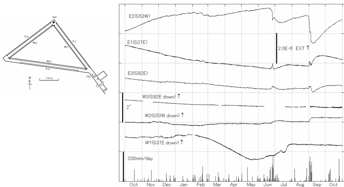
第7図 伊佐観測所における歪・傾斜変化と日雨量 (2012年10月～2013年10月) Fig. 7 Strain changes, tilt changes and daily precipitation at Isa station. (Oct.01,2012～Oct.31,2013).
