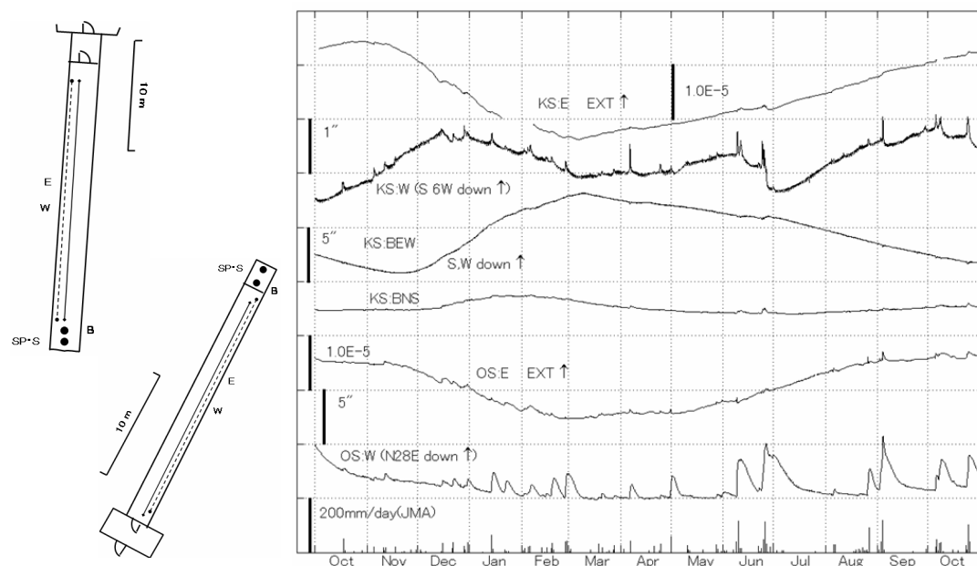
第 10 図 串間・大隈観測所における歪・傾斜変化 (2012 年 10 月～2013 年 10 月)
