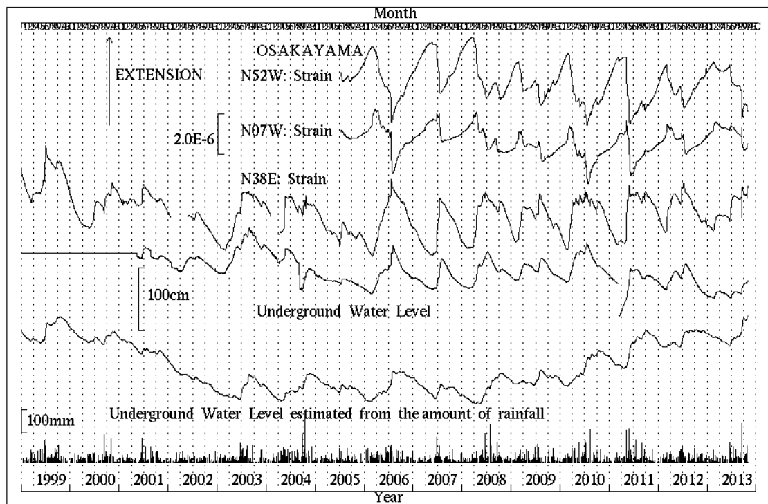
第5図 b 逢坂山観測所における歪変化と日雨量 (1999 年 1 月～2013 年 10 月) Fig.5b Strain change, underground water level, daily precipitation and estimated underground water level from precipitation at Osakayama observatory. (Jan.01,1999～Oct.31,2013).
