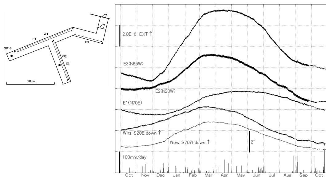
第8図 宿毛観測所における歪変化と日雨量（2012年10月～2013年10月） Fig.8 Strain changes, tilt changes and daily precipitation at Sukumo station. (Oct.01,2012～Oct.31,2013).
