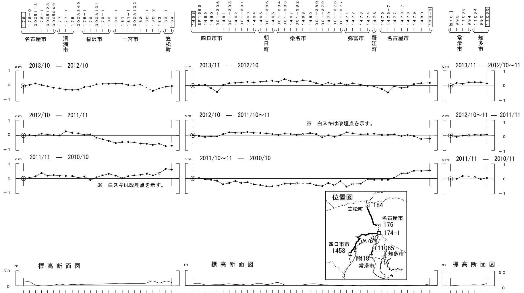
第1図 中京の上下変動 Fig. 1 Results of leveling survey around Nagoya city.
