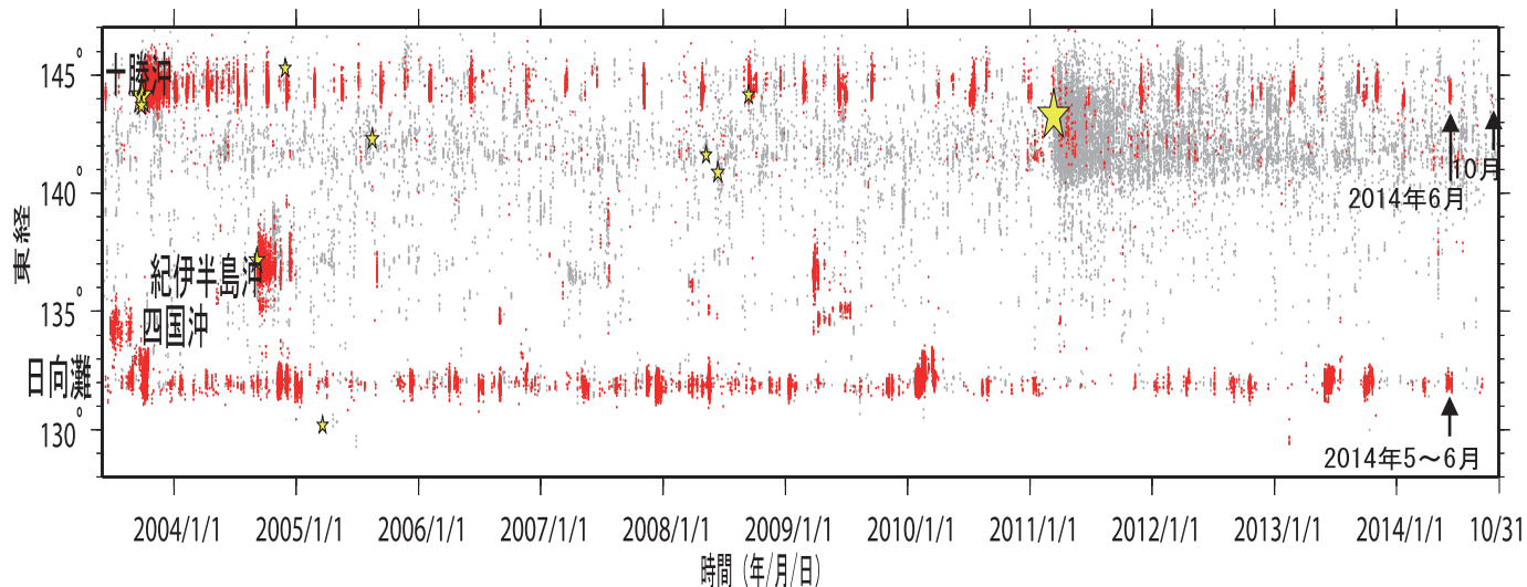
第2図. 2003年6月1日から2014年10月31日までの期間に検出されたイベントの時空間分布. 検出されたイベントを防災科研Hi-net手動検測震源と照合し, 対応する地震が見出されたイベントを灰色丸印で, それ以外を赤色丸印で示す.
