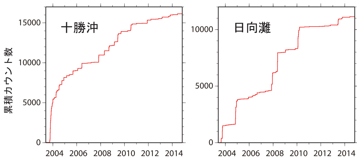
第3図. 十勝沖 (左) および日向灘 (右) における検出イベント累積カウント数の時間変化.
