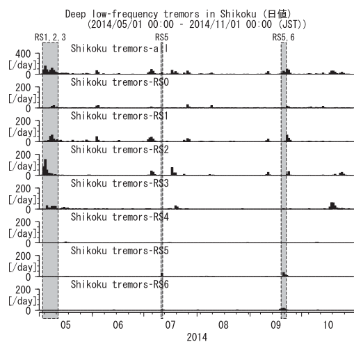
第44図 四国地方における低周波微動の発生個数(2014年5月～2014年10月) Fig.44 Number of deep low frequency tremors in the Shikoku district from May 2014 to October 2014.
