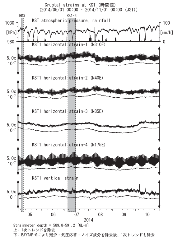
第19図 KSTにおける歪観測結果 (2014年5月～2014年10月) Fig.19 Observed strains at the KST observation site from May 2014 to October 2014.
