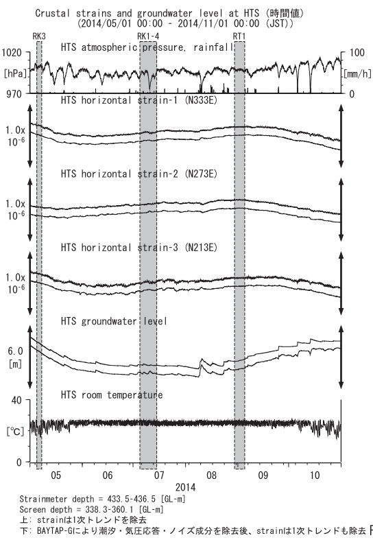
第8図 HTSにおける歪・地下水位観測結果 (2014年5月～2014年10月) Fig.8 Observed strains and groundwater levels at the HTS observation site from May 2014 to October 2014.
