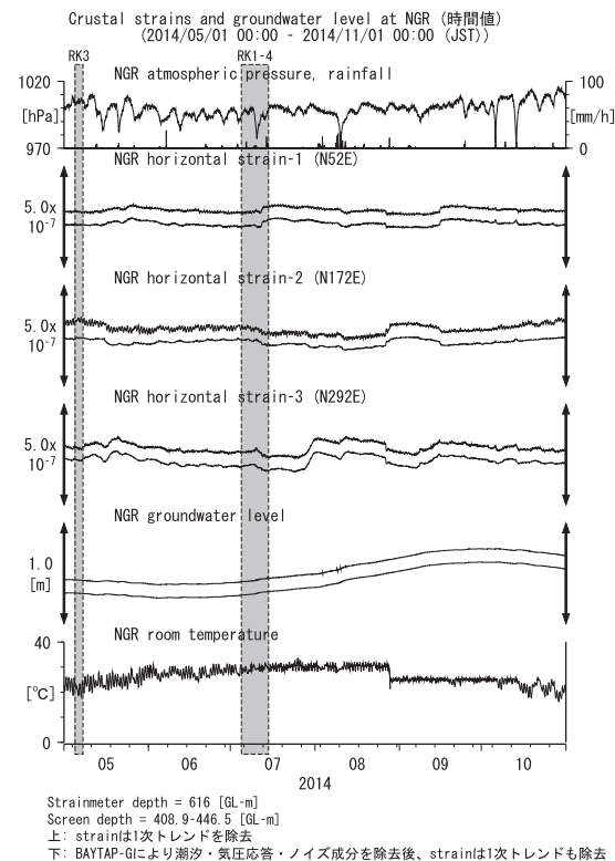
第21図 NGRにおける歪・地下水位観測結果 (2014年5月～2014年10月) Fig.21 Observed strains and groundwater levels at the NGR observation site from May 2014 to October 2014.
