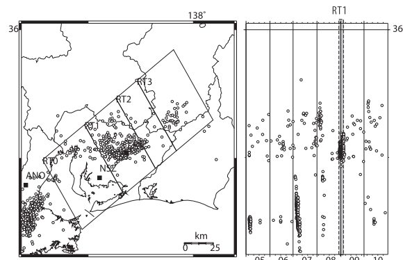
第39図 東海地方における低周波微動の震央分布と時空間分布(2014年5月～2014年10月) Fig.39 Epicentral and space-time distributions of deep low frequency tremors in the Tokai district from May 2014 to October 2014.
