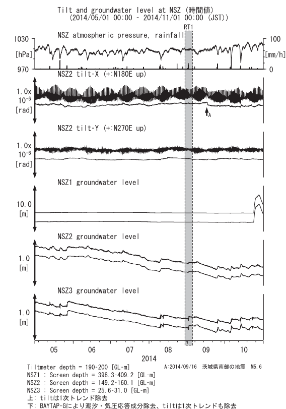
第5図 NSZにおける傾斜・地下水位観測結果 (2014年5月～2014年10月) Fig.5 Observed tilts and groundwater levels at the NSZ observation site from May 2014 to October 2014.
