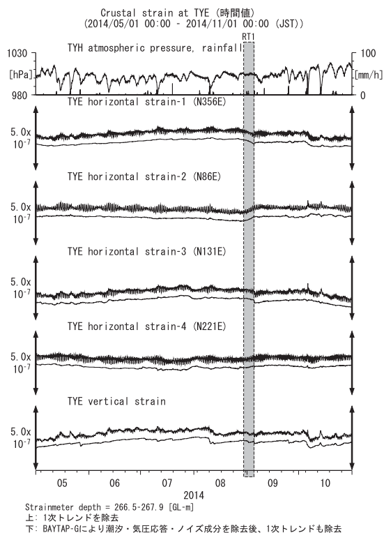
第6図 TYEにおける歪観測結果 (2014年5月～2014年10月) Fig.6 Observed strains at the TYE observation site from May 2014 to October 2014.
