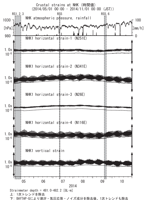
第37図 NHKにおける歪観測結果 (2014年5月～2014年10月)
