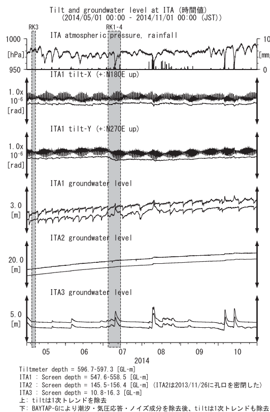
第12図 ITAにおける傾斜・地下水位観測結果 (2014年5月～2014年10月)
