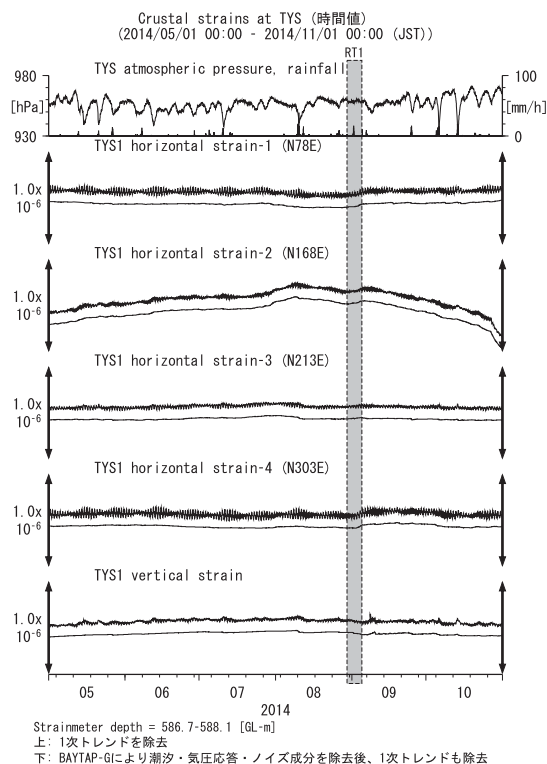
第2図 TYSにおける歪観測結果 (2014年5月～2014年10月) Fig.2 Observed strains at the TYS observation site from May 2014 to October 2014.
