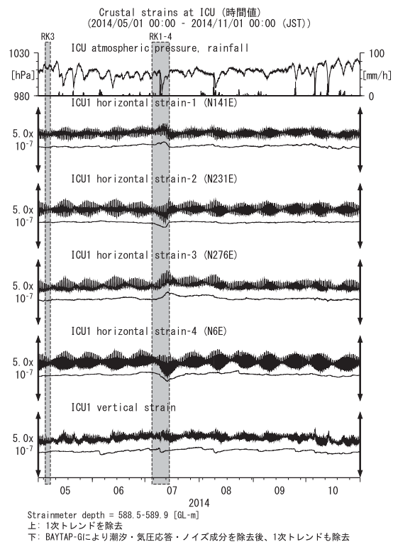
第15図 ICUにおける歪観測結果 (2014年5月～2014年10月) Fig.15 Observed strains at the ICU observation site from May 2014 to October 2014.
