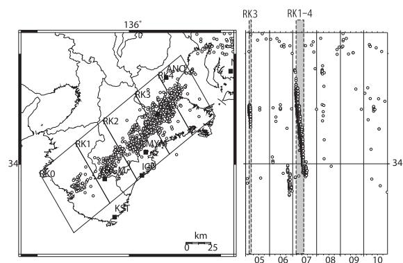
第41図 紀伊半島における低周波微動の震央分布と時空間分布(2014年5月～2014年10月) Fig.41 Epicentral and space-time distributions of deep low frequency tremors in the Kii Peninsula from May 2014 to October 2014.
