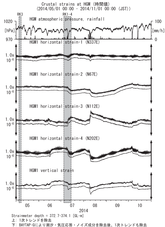
第17図 HGMにおける歪観測結果 (2014年5月～2014年10月) Fig.17 Observed strains at the HGM observation site from May 2014 to October 2014.
