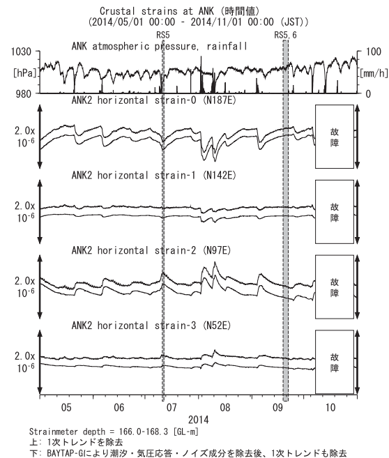
第23図 ANKにおける歪観測結果 (2014年5月～2014年10月) Fig.23 Observed strains at the ANK observation site from May 2014 to October 2014.
