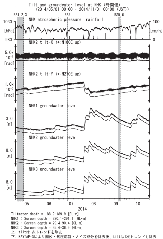
第38図 NHKにおける傾斜・地下水位観測結果 (2014年5月～2014年10月) Fig.38 Observed tilts and groundwater levels at the NHK observation site from May 2014 to October 2014.
