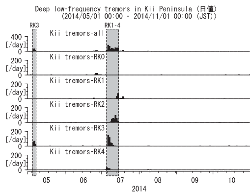
第42図 紀伊半島における低周波微動の発生個数(2014年5月～2014年10月) Fig.42 Number of deep low frequency tremors in the Kii Peninsula from May 2014 to October 2014.
