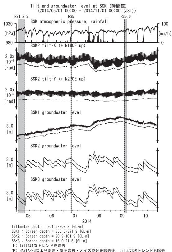
第30図 SSKにおける傾斜・地下水位観測結果 (2014年5月～2014年10月) Fig.30 Observed tilts and groundwater levels at the SSK observation site from May 2014 to October 2014.
