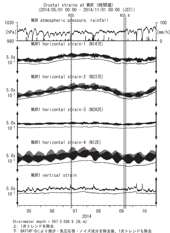
第25図 MURにおける歪観測結果 (2014年5月～2014年10月) Fig.25 Observed strains at the MUR observation site from May 2014 to October 2014.
