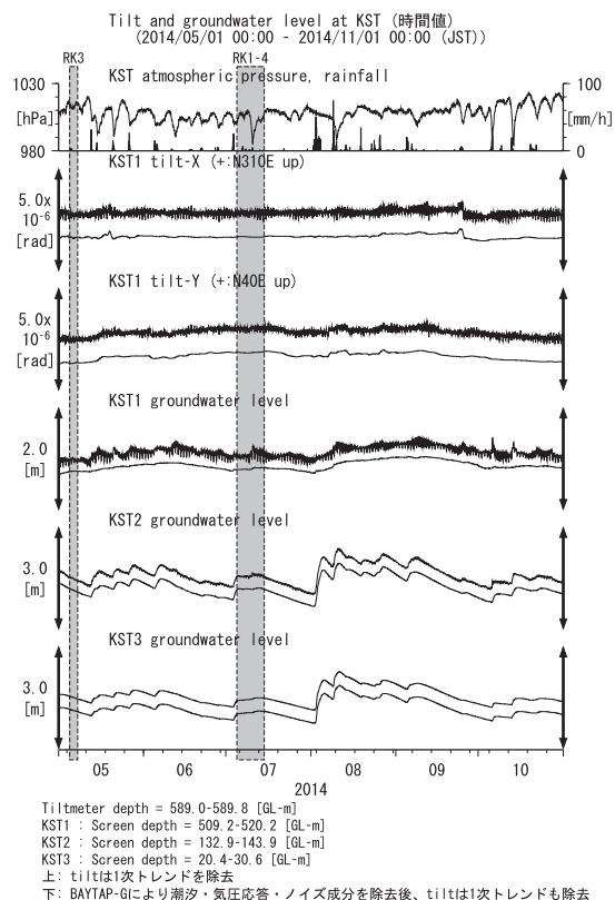
第20図 KSTにおける傾斜・地下水位観測結果 (2014年5月～2014年10月) Fig.20 Observed tilts and groundwater levels at the KST observation site from May 2014 to October 2014.
