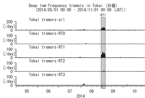
第40図 東海地方における低周波微動の発生個数(2014年5月～2014年10月) Fig.40 Number of deep low frequency tremors in the Tokai district from May 2014 to October 2014.
