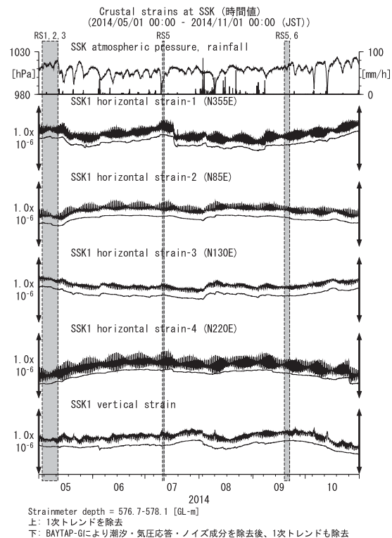
第29図 SSKにおける歪観測結果 (2014年5月～2014年10月) Fig.29 Observed strains at the SSK observation site from May 2014 to October 2014.
