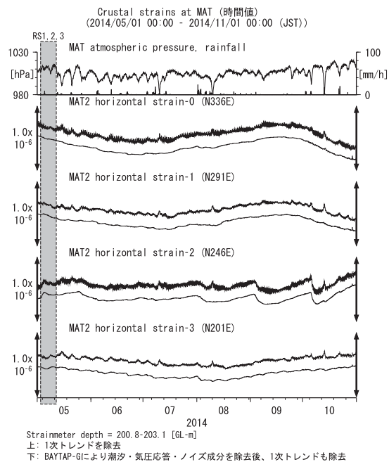
第35図 MATにおける歪観測結果 (2014年5月～2014年10月)
