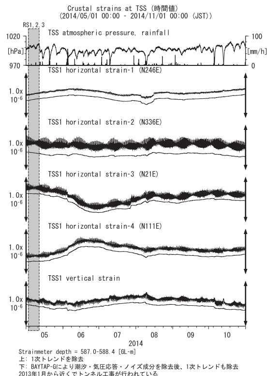
第31図 TSSにおける歪観測結果 (2014年5月～2014年10月) Fig.31 Observed strains at the TSS observation site from May 2014 to October 2014.
