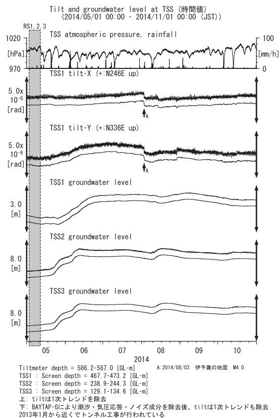
第32図 TSSにおける傾斜・地下水位観測結果 (2014年5月～2014年10月) Fig.32 Observed tilts and groundwater levels at the TSS observation site from May 2014 to October 2014.
