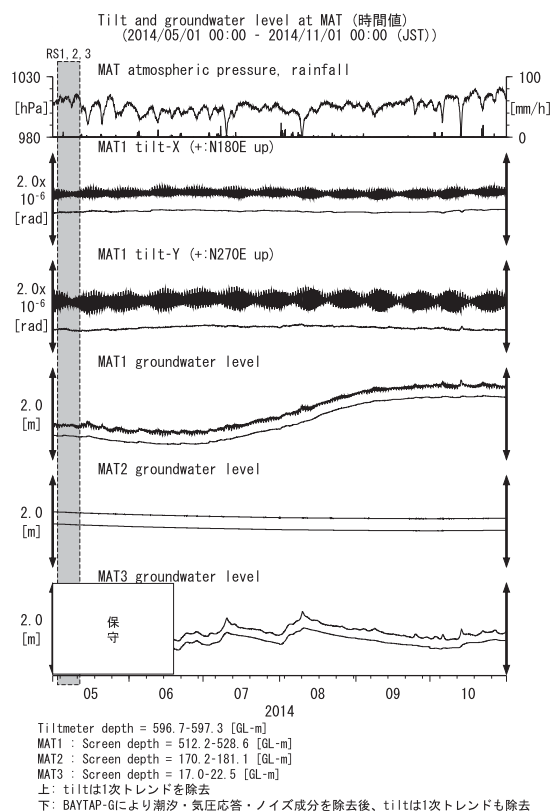
第36図 MATにおける傾斜・地下水位観測結果 (2014年5月～2014年10月)
