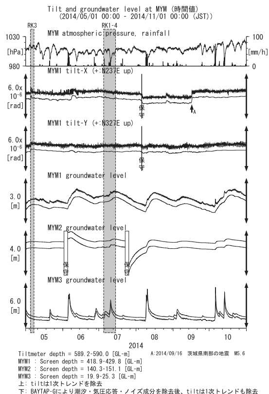
第14図 MYMにおける傾斜・地下水位観測結果 (2014年5月～2014年10月) Fig.14 Observed tilts and groundwater levels at the MYM observation site from May 2014 to October 2014.
