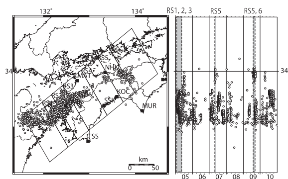
第43図 四国地方における低周波微動の震央分布と時空間分布(2014年5月～2014年10月) Fig.43 Epicentral and space-time distributions of deep low frequency tremors in the Shikoku district from May 2014 to October 2014.
