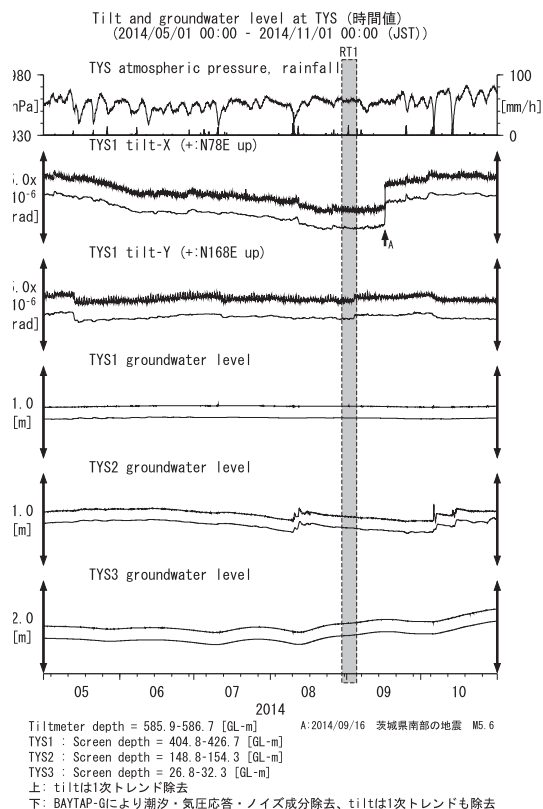
第3図 TYSにおける傾斜・地下水位観測結果 (2014年5月～2014年10月) Fig.3 Observed tilts and groundwater levels at the TYS observation site from May 2014 to October 2014.
