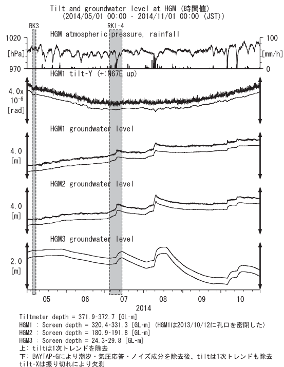
第18図 HGMにおける傾斜・地下水位観測結果 (2014年5月～2014年10月) Fig.18 Observed tilt and groundwater levels at the HGM observation site from May 2014 to October 2014.
