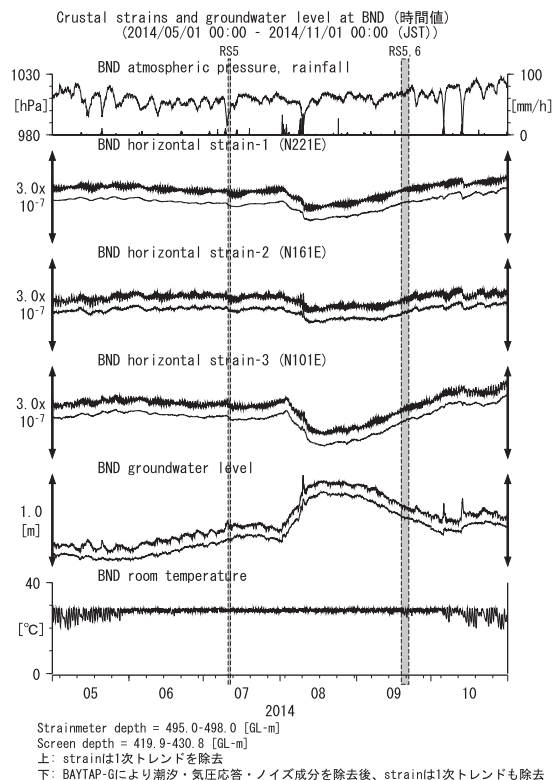
第22図 BNDにおける歪・地下水位観測結果 (2014年5月～2014年10月)
