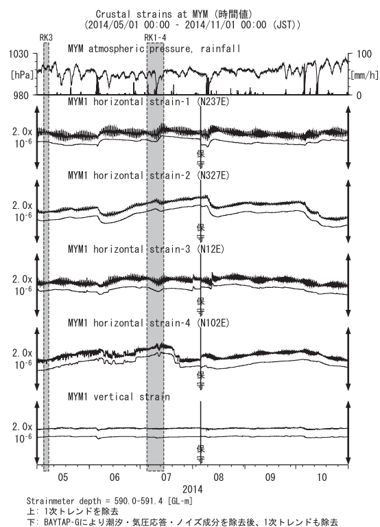
第13図 MYMにおける歪観測結果 (2014年5月～2014年10月)
