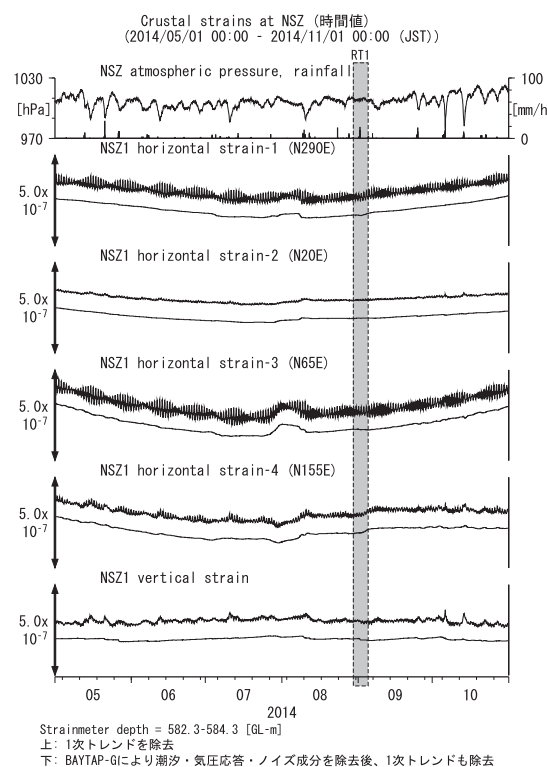
第4図 NSZにおける歪観測結果 (2014年5月～2014年10月) Fig.4 Observed strains at the NSZ observation site from May 2014 to October 2014.
