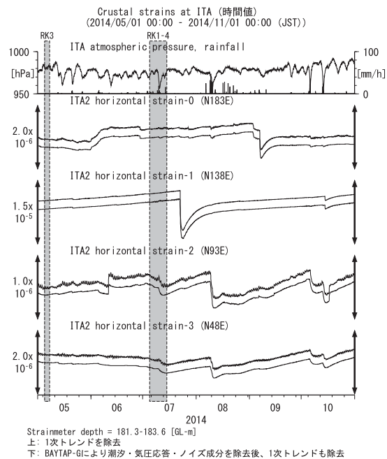
第11図 ITAにおける歪観測結果 (2014年5月～2014年10月)
