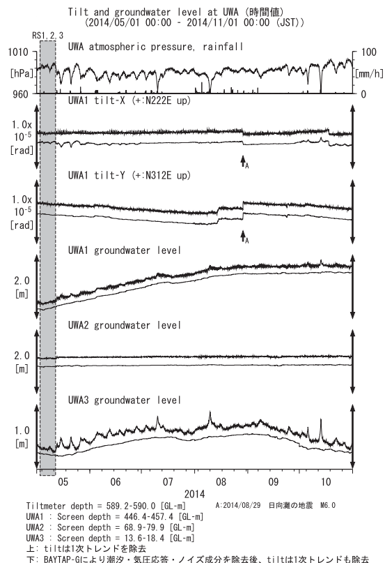
第34図 UWAにおける傾斜・地下水位観測結果 (2014年5月～2014年10月)
