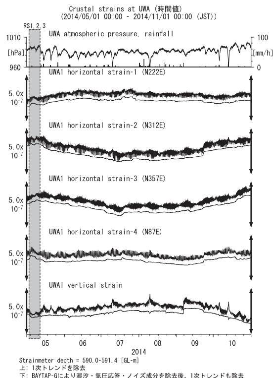
第33図 UWAにおける歪観測結果 (2014年5月～2014年10月) Fig.33 Observed strains at the UWA observation site from May 2014 to October 2014.
