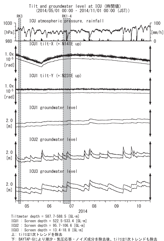
第16図 ICUにおける傾斜・地下水位観測結果 (2014年5月～2014年10月) Fig.16 Observed tilts and groundwater levels at the ICU observation site from May 2014 to October 2014.
