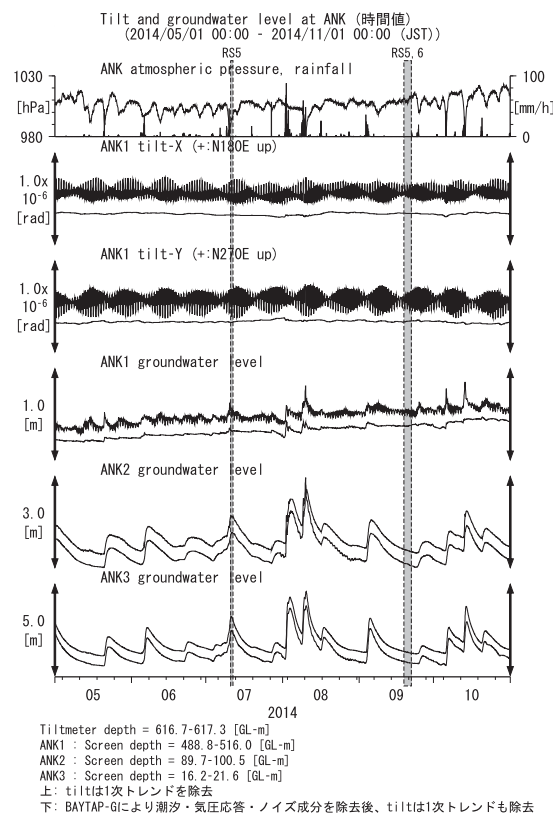
第24図 ANKにおける傾斜・地下水位観測結果 (2014年5月～2014年10月)
