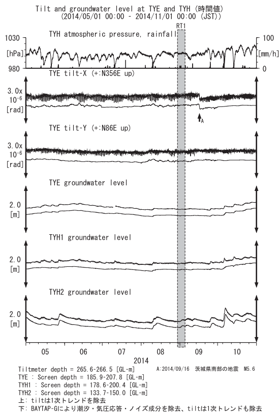
第7図 TYEおよびTYHにおける傾斜・地下水位観測結果 (2014年5月～2014年10月) Fig.7 Observed tilts and groundwater levels at the TYE and the TYH observation site from May 2014 to October 2014.
