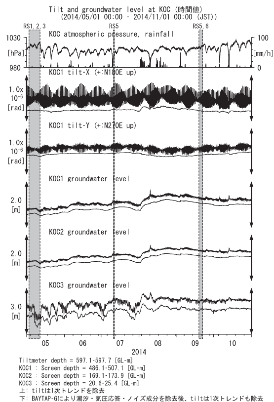
第28図 KOCにおける傾斜・地下水位観測結果 (2014年5月～2014年10月)
