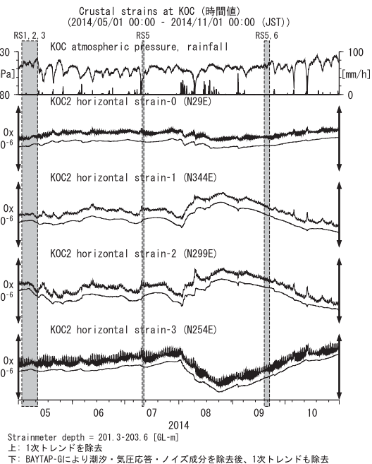
第27図 KOCにおける歪観測結果 (2014年5月～2014年10月) Fig.27 Observed strains at the KOC observation site from May 2014 to October 2014.
