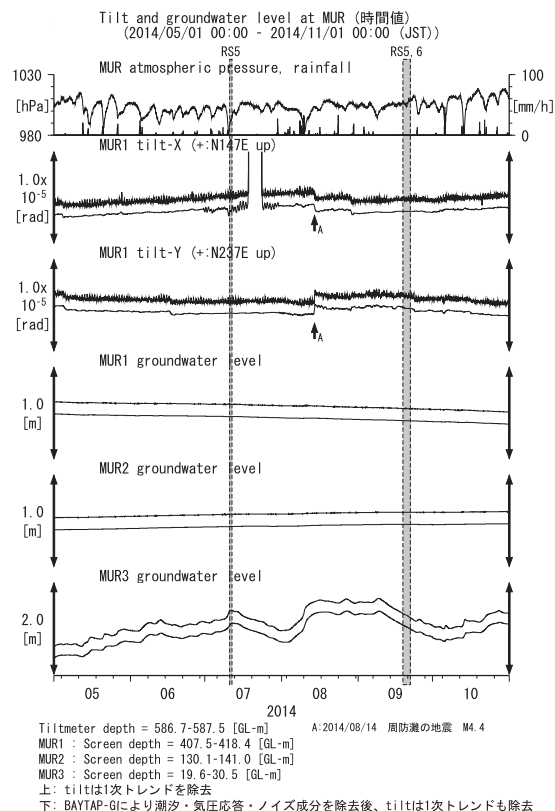
第26図 MURにおける傾斜・地下水位観測結果 (2014年5月～2014年10月)
