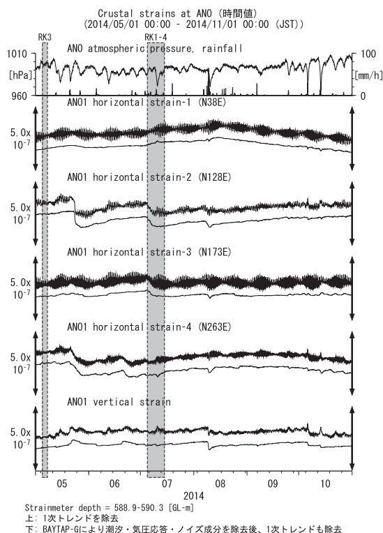
第9図 ANOにおける歪観測結果 (2014年5月～2014年10月) Fig.9 Observed strains at the ANO observation site from May 2014 to October 2014.
