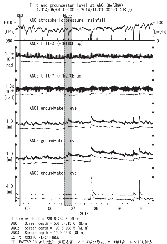
第10図 ANOにおける傾斜・地下水位観測結果 (2014年5月～2014年10月)
