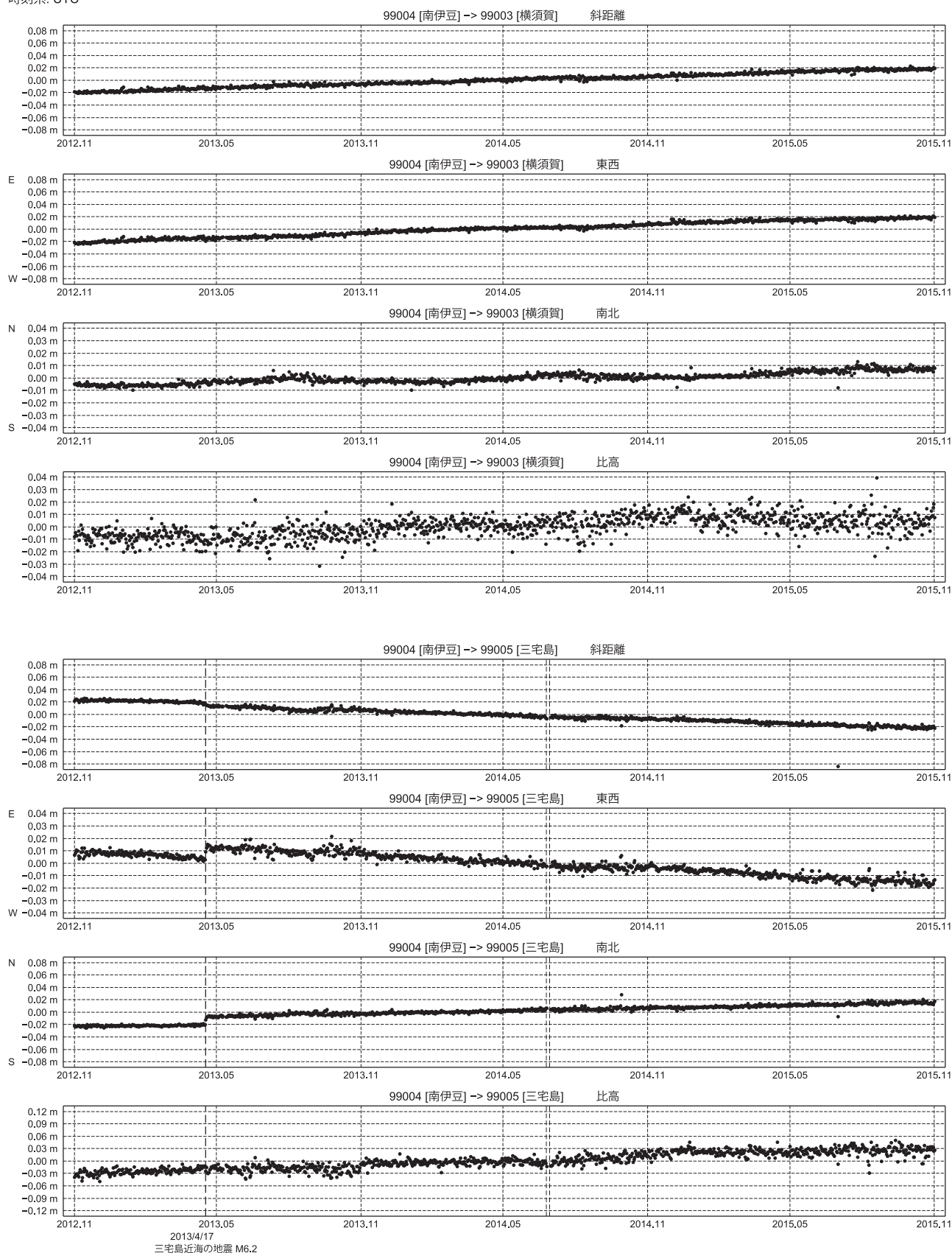
第3図 南伊豆基点での横須賀および三宅島のGPS連続観測結果 (2012/11/1~2015/10/31)
