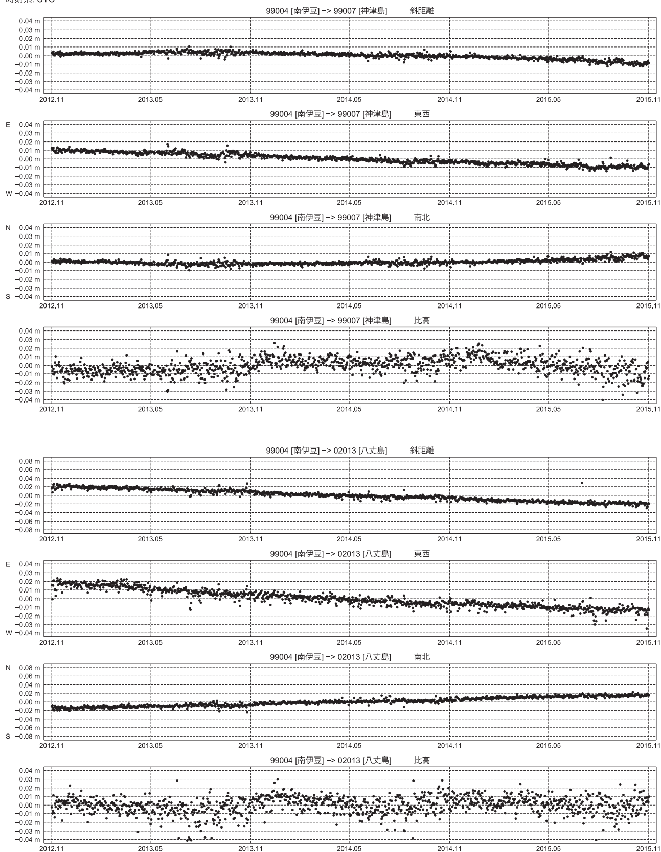
第4図 南伊豆基点での神津島および八丈島のGPS連続観測結果 (2012/11/1~2015/10/31)
