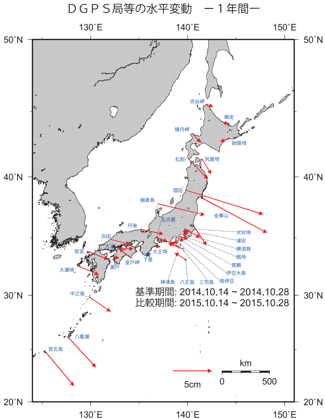
第 5 図 DGPS 局等の GPS 連続観測から求めた水平変動
