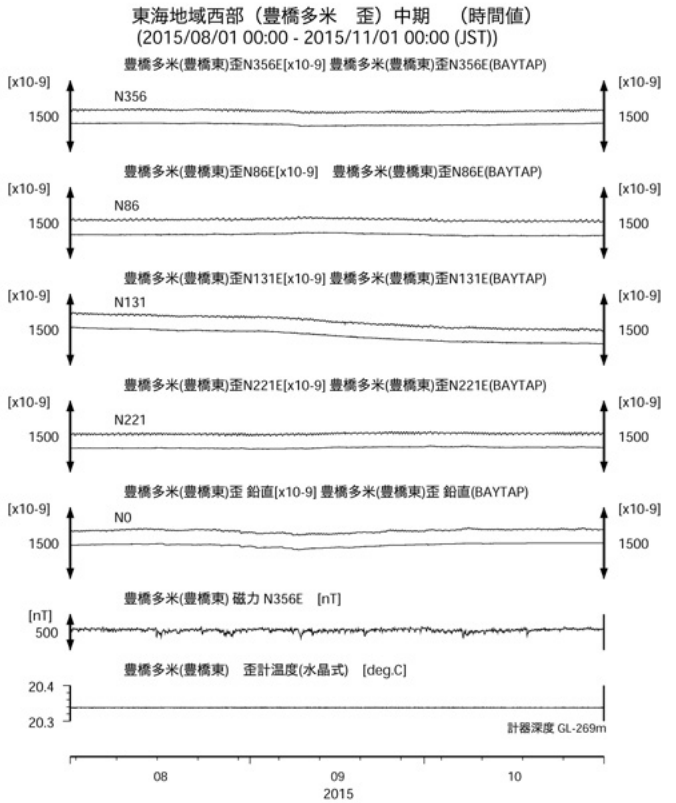
第10図 東海地域西部(豊橋多米)の歪等の観測結果(2015年8月～2015年10月)
