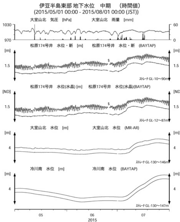
第11図 伊豆半島東部の地下水等の観測結果(2015年5月～2015年7月)
