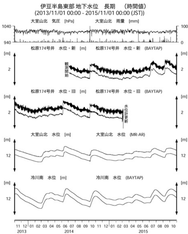
第19図 伊豆半島東部の地下水等の観測結果(2013年11月～2015年10月) Fig.19 Observed groundwater levels and others in the eastern Izu peninsula from Nov. 2013 to Oct. 2015.
