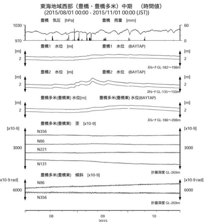
第8図 東海地域西部(豊橋・豊橋多米)の地下水等の観測結果(2015年8月～2015年10月) Fig.8 Observed groundwater levels and others at the Toyohashi and Toyohashi-tame observation sites in the western Tokai district from Aug. 2015 to Oct. 2015.
