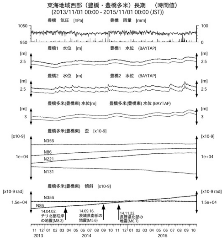
第17図 東海地域西部(豊橋・豊橋多米)の地下水等の観測結果(2013年11月～2015年10月) Fig.17 Observed groundwater levels and others at the Toyohashi and Toyohashi-tame observation sites in the western Tokai district from Nov. 2013 to Oct. 2015.
