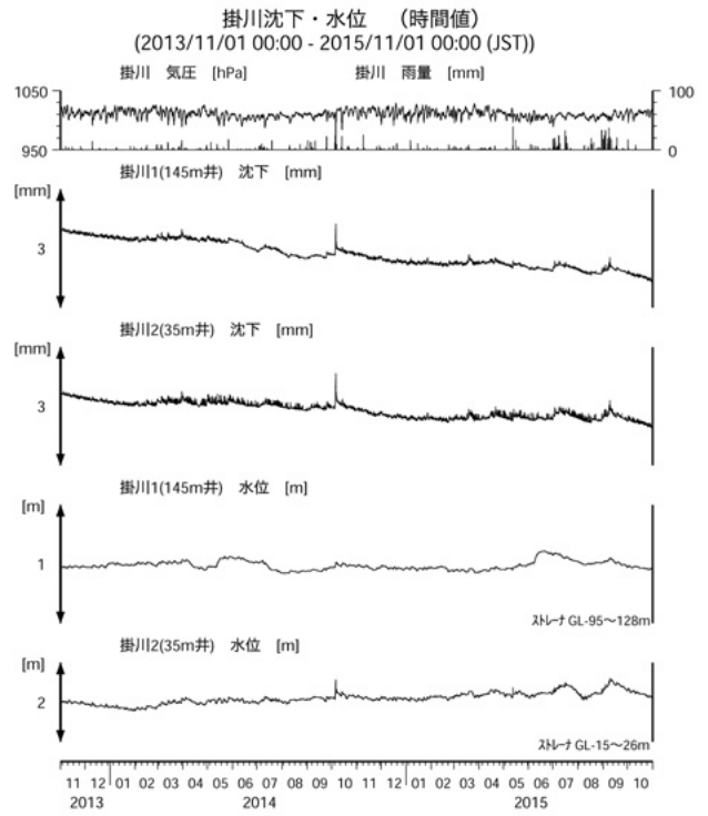
第22図 掛川における沈下等の観測結果(2013年11月～2015年10月) Fig.22 Observed subsidence data and others at the Kakegawa observation well from Nov. 2013 to Oct. 2015.
