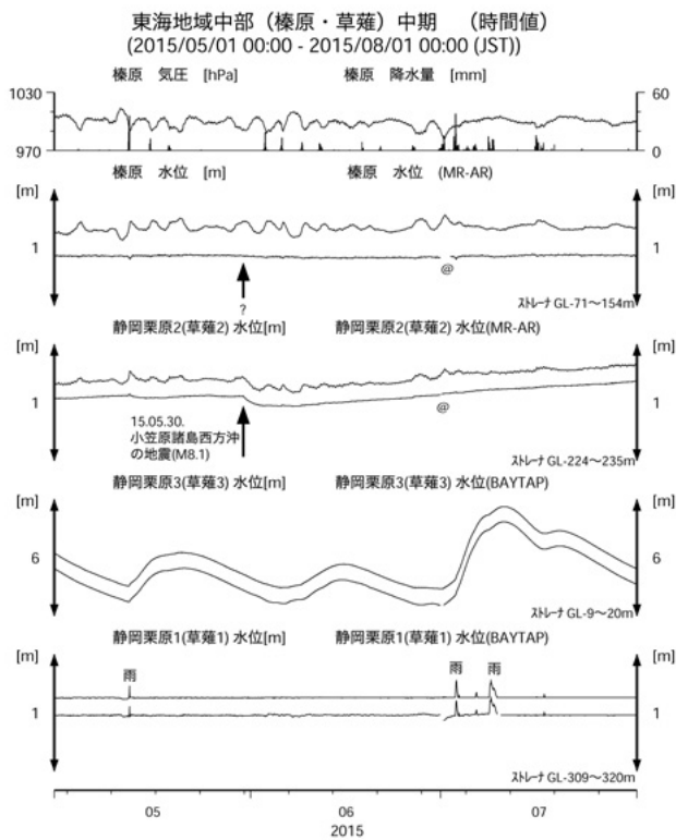
第3図 東海地域中部の地下水等の観測結果(2015年5月～2015年7月) Fig.3 Observed groundwater levels and others in the central Tokai district from May 2015 to Jul. 2015.
