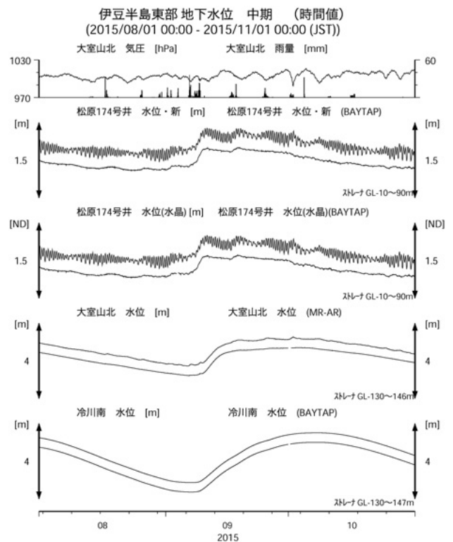
第12図 伊豆半島東部の地下水等の観測結果(2015年8月～2015年10月)
