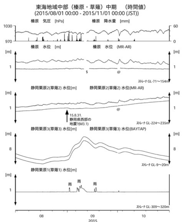
第4図 東海地域中部の地下水等の観測結果(2015年8月～2015年10月) Fig.4 Observed groundwater levels and others in the central Tokai district from Aug. 2015 to Oct. 2015.
