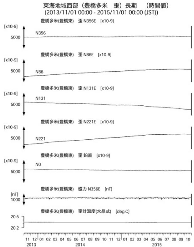
第18図 東海地域西部(豊橋多米)の歪等の観測結果(2013年11月～2015年10月) Fig.18 Observed strain and others at the Toyohashi-tame observation site in the western Tokai district from Nov. 2013 to Oct. 2015.
