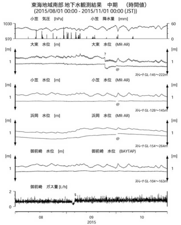
第6図 東海地域南部の地下水等の観測結果(2015年8月～2015年10月) Fig.6 Observed groundwater levels and others in the southern Tokai district from Aug. 2015 to Oct. 2015.
