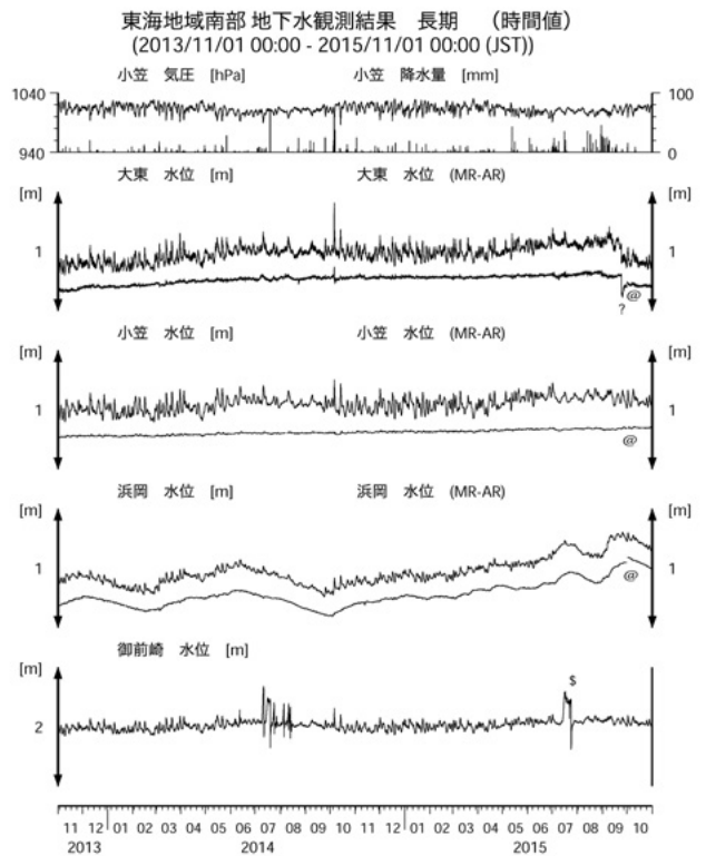
第16図 東海地域南部の地下水等の観測結果(2013年11月～2015年10月) Fig.16 Observed groundwater levels and others in the southern Tokai district from Nov. 2013 to Oct. 2015.
