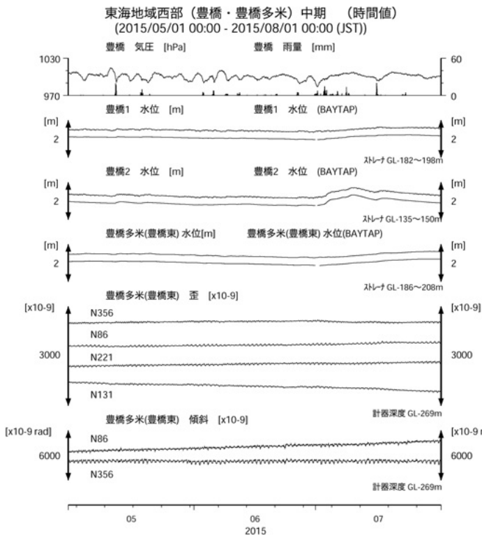
第7図 東海地域西部(豊橋・豊橋多米)の地下水等の観測結果(2015年5月～2015年7月) Fig.7 Observed groundwater levels and others at the Toyohashi and Toyohashi-tame observation sites in the western Tokai district from May 2015 to Jul. 2015.
