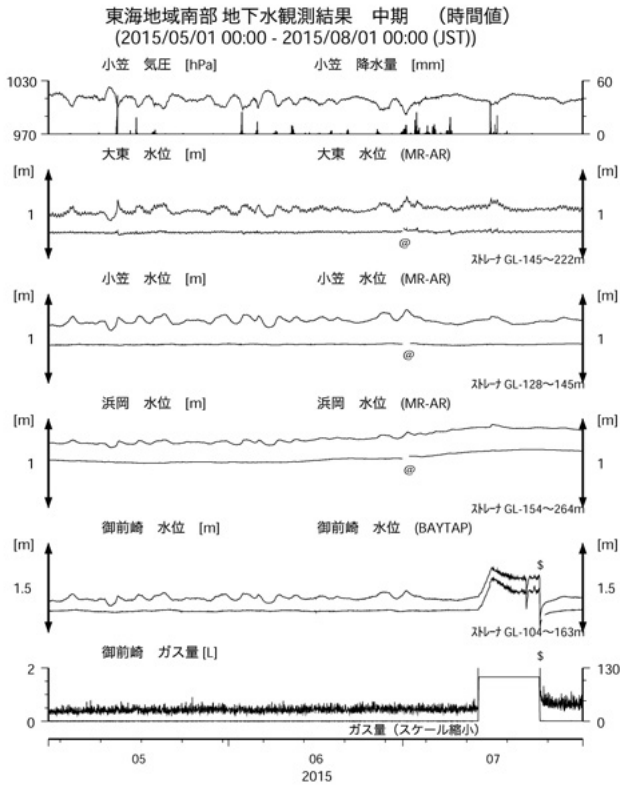
第5図 東海地域南部の地下水等の観測結果(2015年5月～2015年7月) Fig.5 Observed groundwater levels and others in the southern Tokai district from May 2015 to Jul. 2015.
