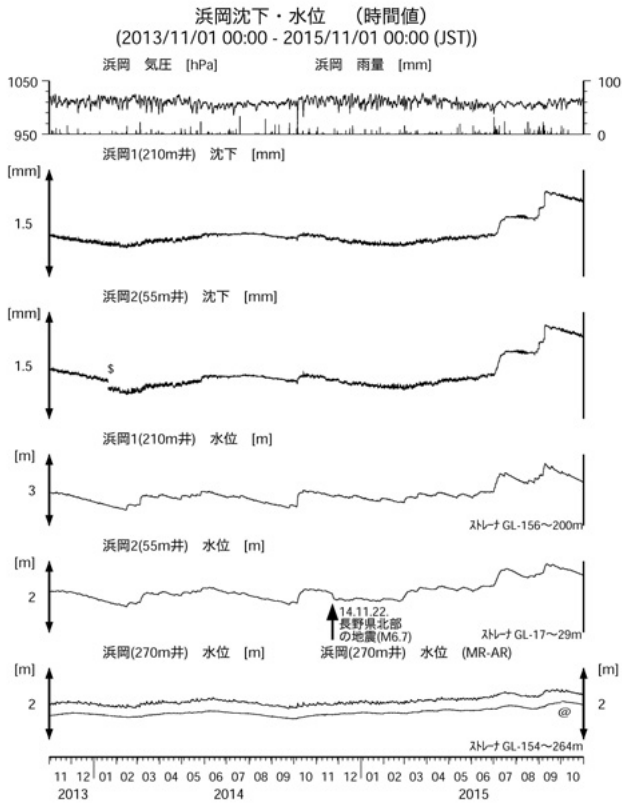
第21図 浜岡における沈下等の観測結果(2013年11月～2015年10月) Fig.21 Observed subsidence data and others at the Hamaoka observation well from Nov. 2013 to Oct. 2015.
