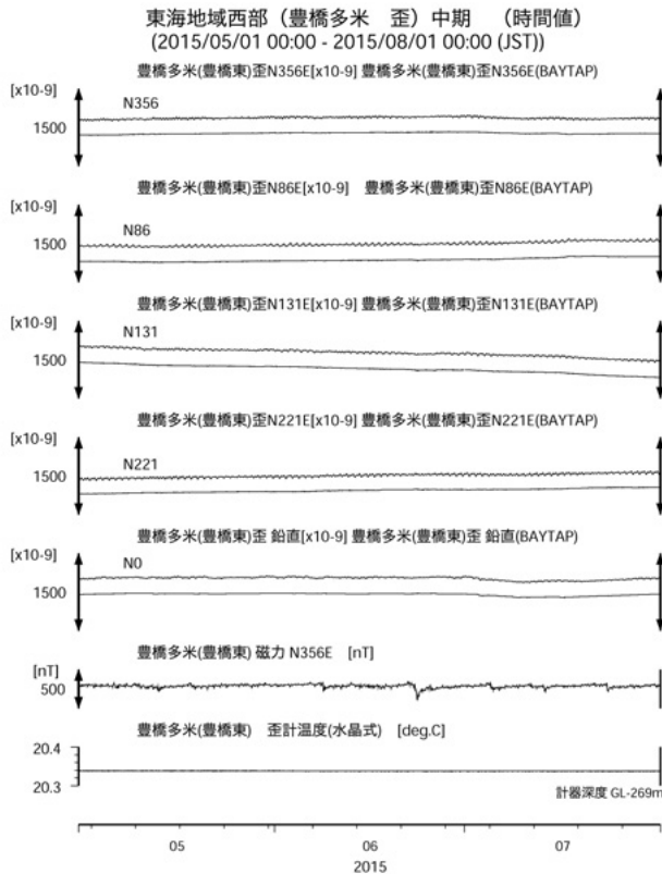
第9図 東海地域西部(豊橋多米)の歪等の観測結果(2015年5月～2015年7月)
