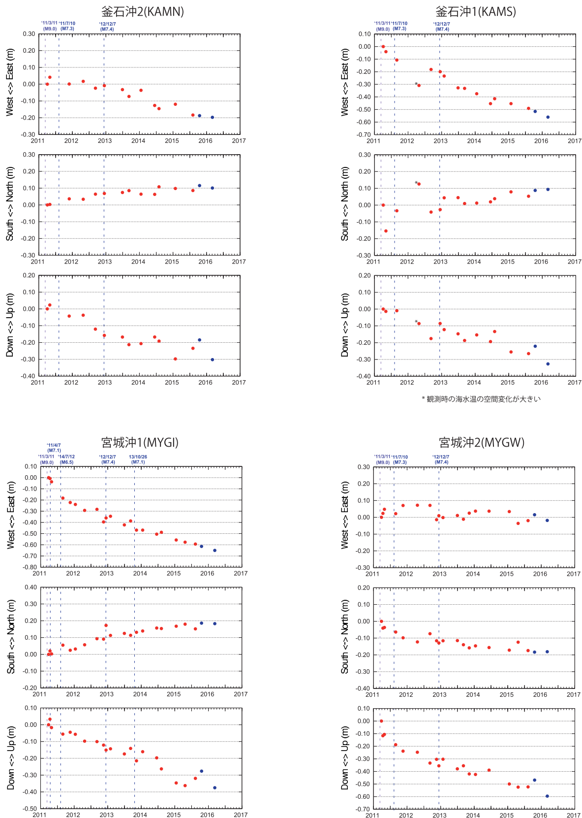
第2図 各海底基準点の局位置解の時系列【電子基準点「福江」固定】
