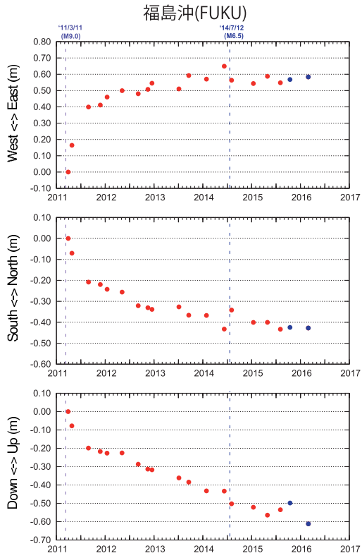
第 2 図 各海底基準点の局位置解の時系列【電子基準点「福江」固定】
