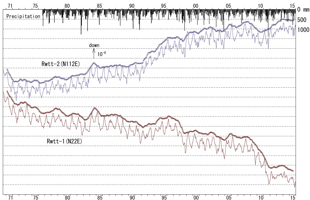
第3図 読取型水管傾斜計による累積傾斜変化 (□=12ヶ月移動平均値・実線=月平均値) および月別雨量 Fig.3 Cumulative tilt change by reading type WTT (□=12month's running mean,solid line=monthly mean)
