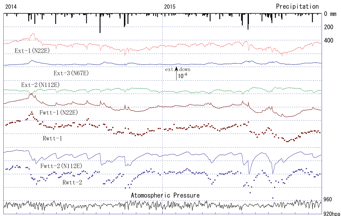
第 1 図 富士川観測所における水晶管伸縮計・水管傾斜計（実線＝フロート型・黒丸＝読取型） 気圧の日平均記録および日降雨量（2014，2015 年）
