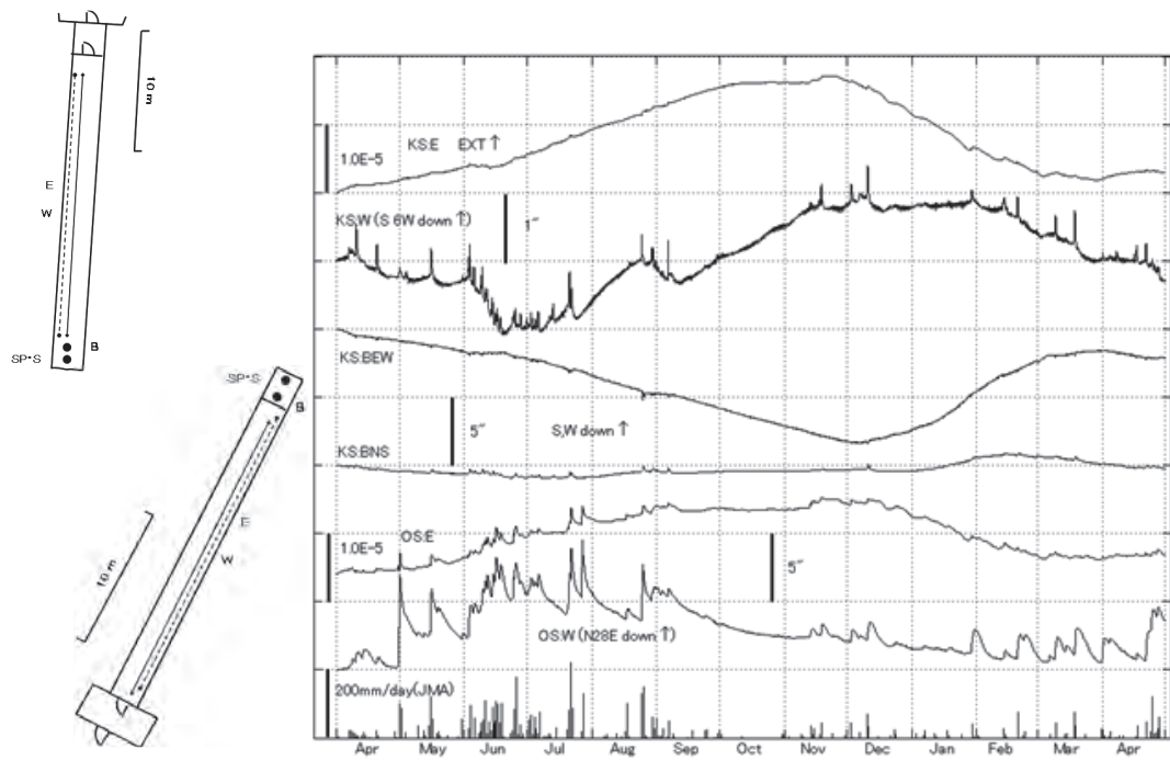
第 10 図 串間・大隈観測所における歪・傾斜変化 (2015 年 4 月～2016 年 4 月)
