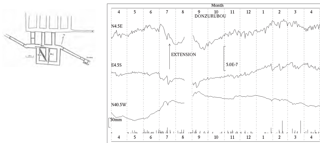
第4図 a 屯鶴峯観測所における歪変化と日雨量（2015年4月～2016年4月） Fig.4a Strain changes and daily precipitation at Donzurubou observatory. (Apr.01,2015 ~ Apr.30,2016).
