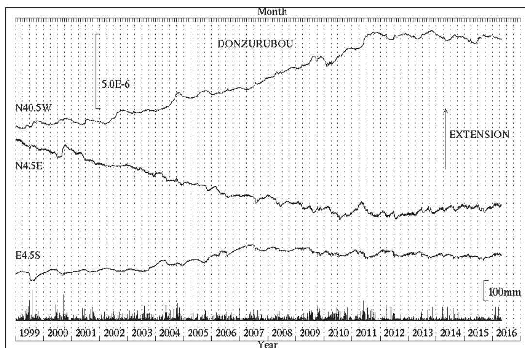
第4図 b 屯鶴峯観測所における歪変化と日雨量（1999年1月～2016年4月） Fig.4b Strain changes and daily precipitation at Donzurubou observatory. (Jan.1,1999 ~ Apr.30,2016).
