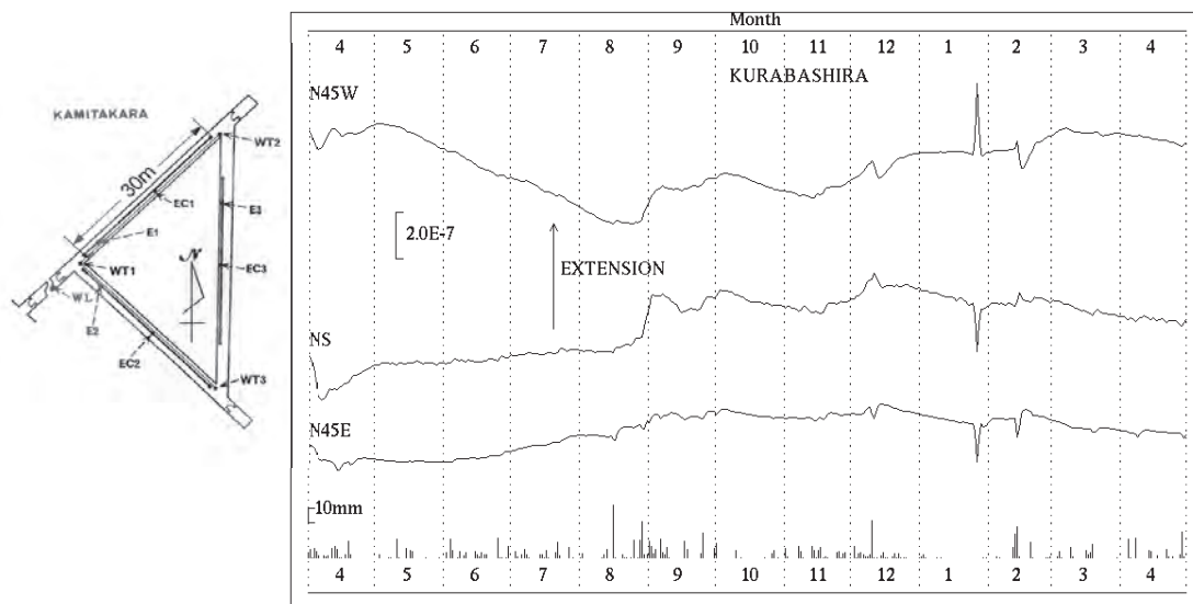
第 2 図 上宝観測所蔵柱観測室における歪変化と日雨量（2015 年 4 月～2016 年 4 月）
