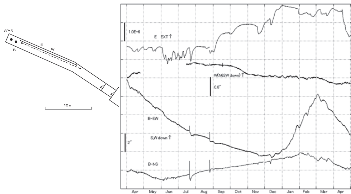
第 9 図 高城観測所における歪変化と傾斜変化（2015 年 4 月～2016 年 4 月）
