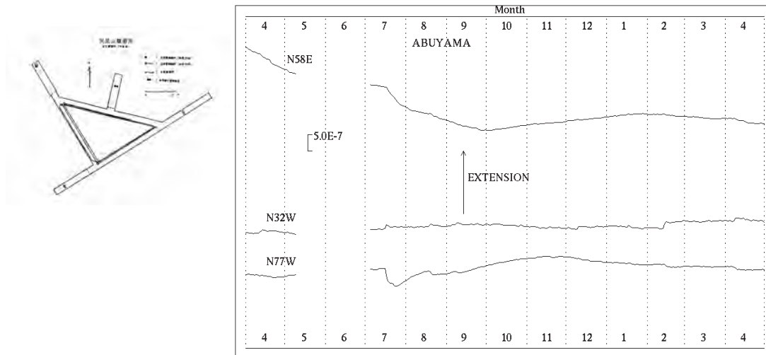
第3図 a 阿武山観測所における歪変化と日雨量（2015年4月～2016年4月）
