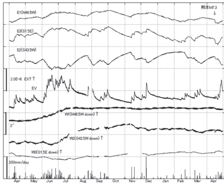
第 6 図 宮崎観測所における歪・傾斜変化と日雨量（2015 年 4 月～2016 年 4 月）
