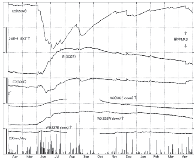
第 7 図 伊佐観測所における歪・傾斜変化と日雨量（2015 年 4 月～2016 年 4 月）
