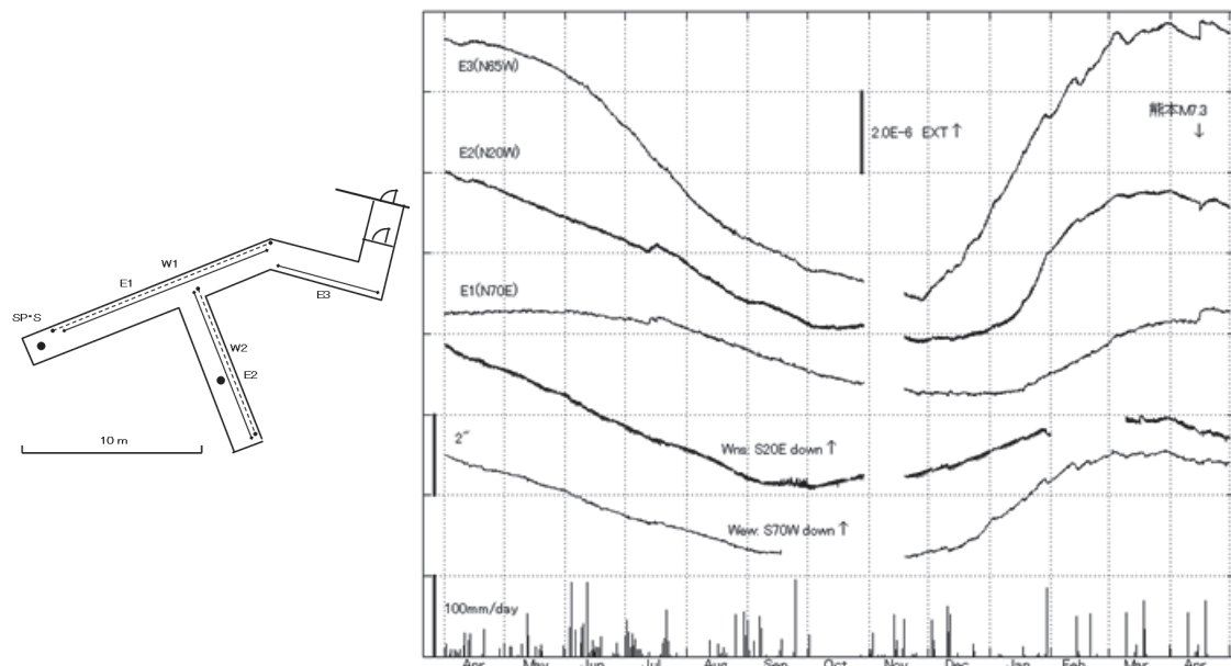
第 8 図 宿毛観測所における歪変化と日雨量（2015 年 4 月～2016 年 4 月）
