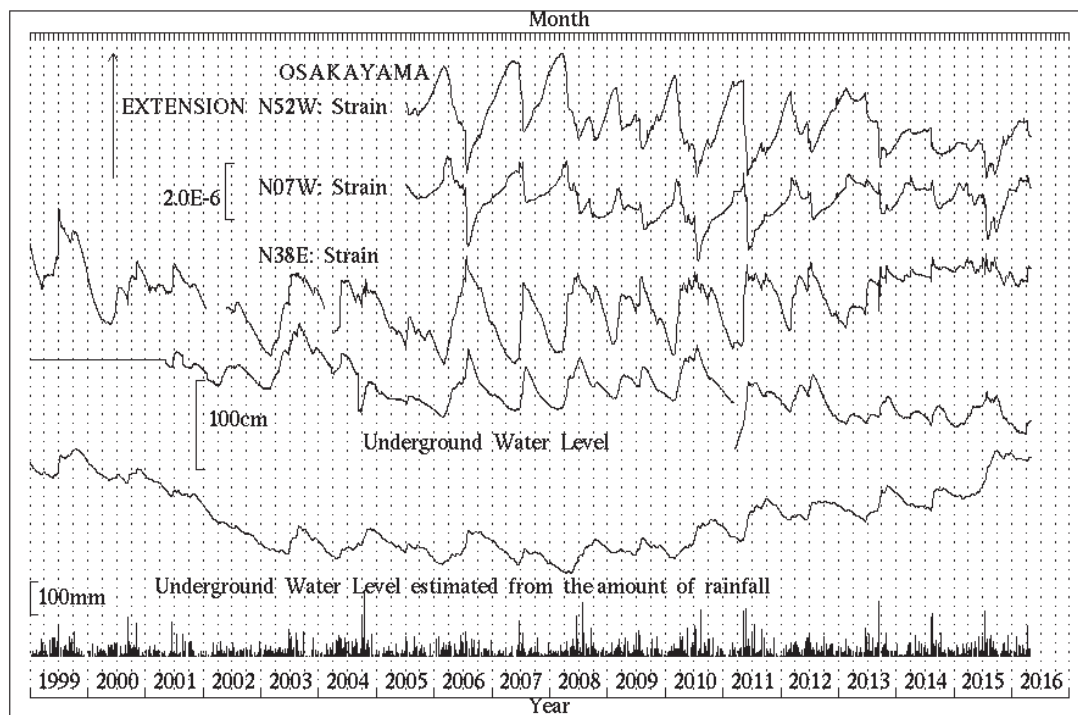
第 5 図 b 逢坂山観測所における歪変化と日雨量（1999 年 1 月～2016 年 4 月）
