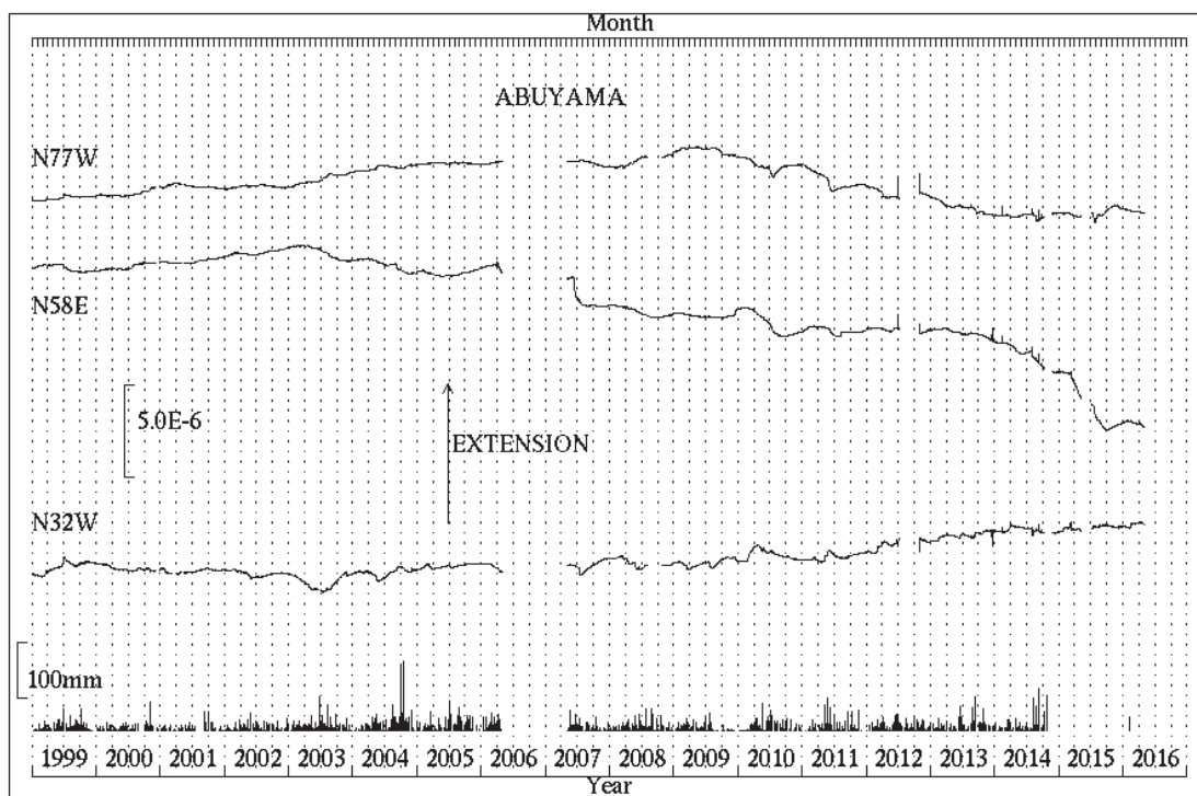
第3図 b 阿武山観測所における歪変化と日雨量（1999年1月～2016年4月）
