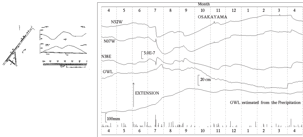
第 5 図 a 逢坂山観測所における歪変化と日雨量（2015 年 4 月～2016 年 4 月）
