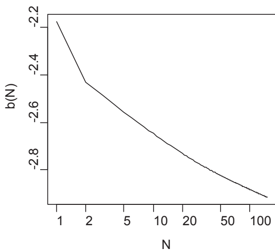
(c) M_{\text{main}} の係数 b(N)
