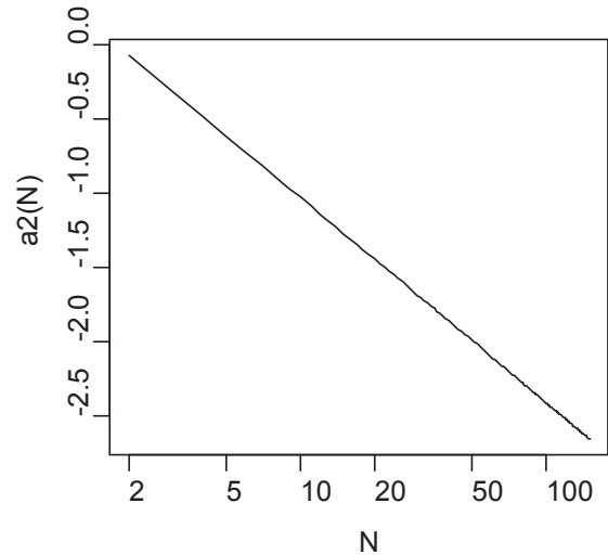
(b) M_1 - M_2 の係数 a_2(N)
