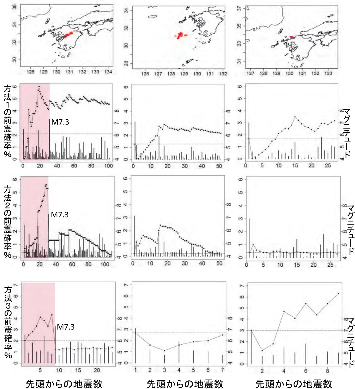
第1図 前震確率の推移（発生地震の順番）。左からパネルの列は順に熊本地震，鹿児島西方沖地震，福岡県西方沖地震。上2列目から順に方法1 2) ，方法2 5) ，方法3 6) による確率予測。
