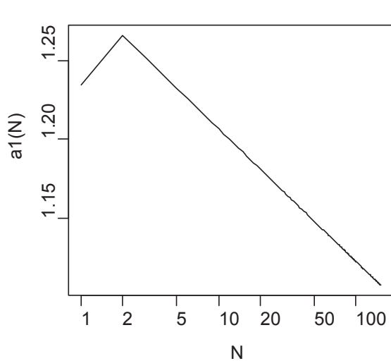
(a) M_1 の係数 a_1(N)
