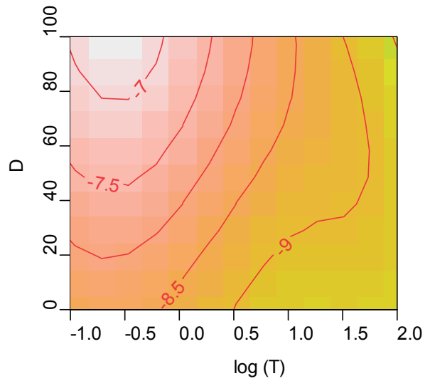
(d) f(N, D, T) ( N=8 のとき )
