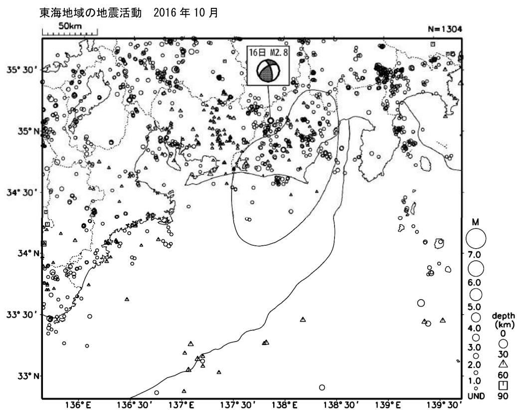
第1図(f) つづき (2016年10月)
