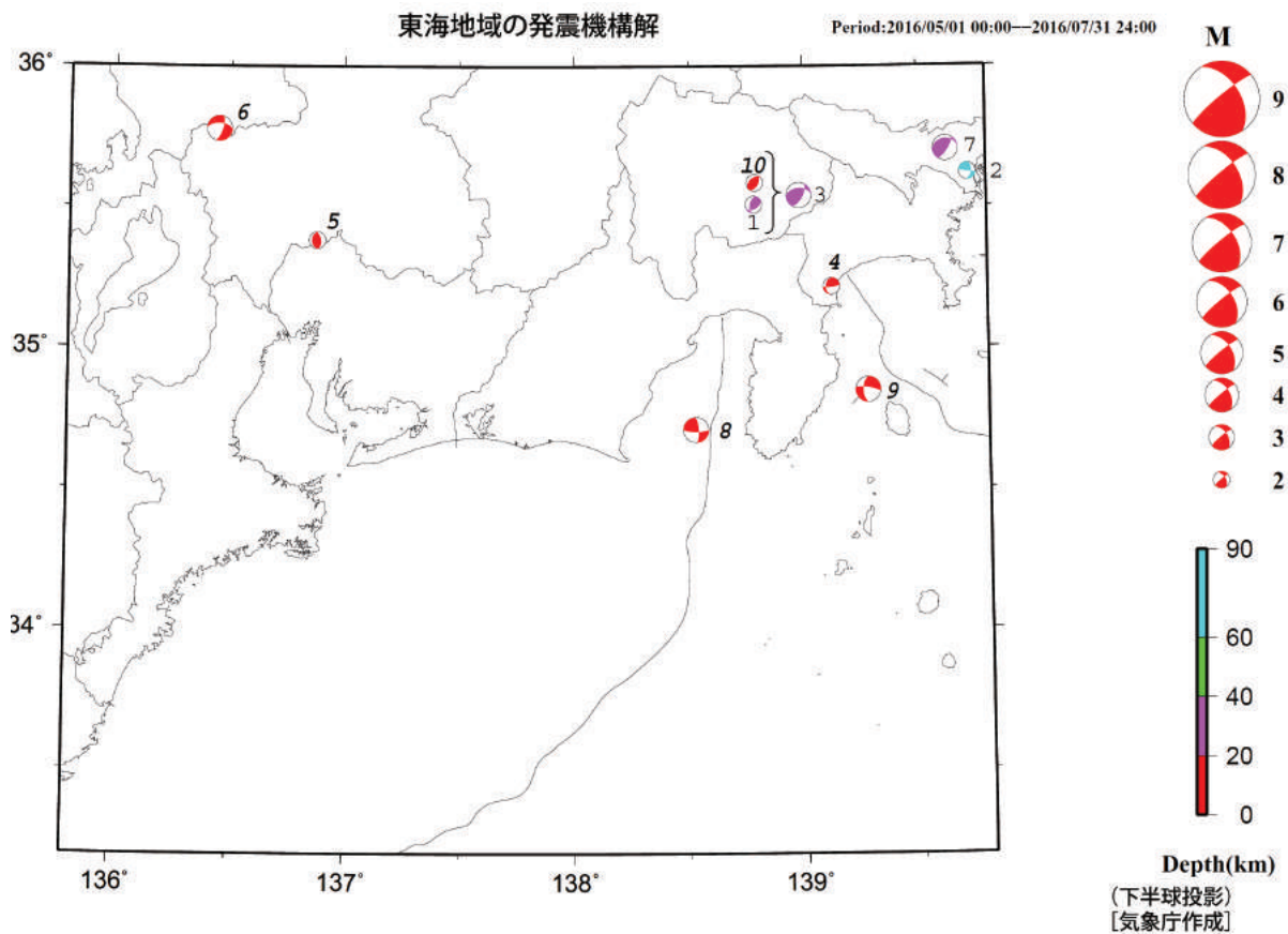
第2図(a) 東海で発生した主な地震の発震機構解 (2016年5月～7月)
