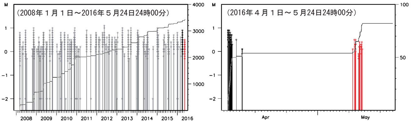
領域a内のM-T図と回数積算図
