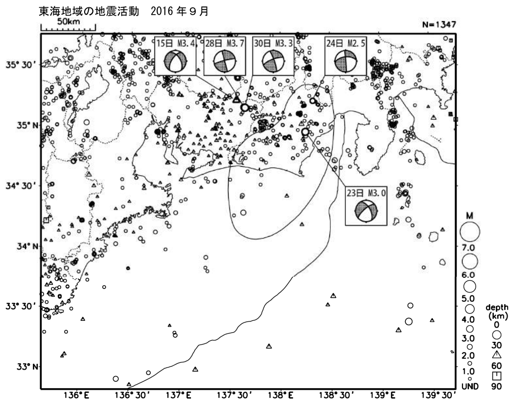
第1図(e) つづき (2016年9月)
