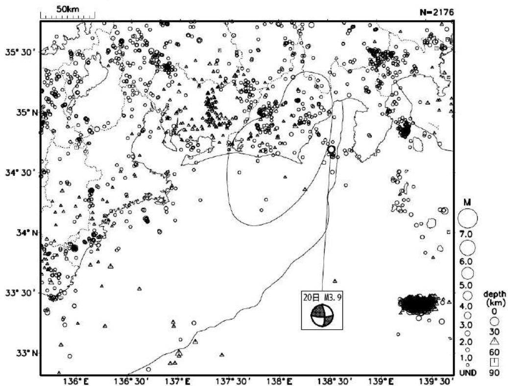
第1図(c) つづき (2016年7月)
