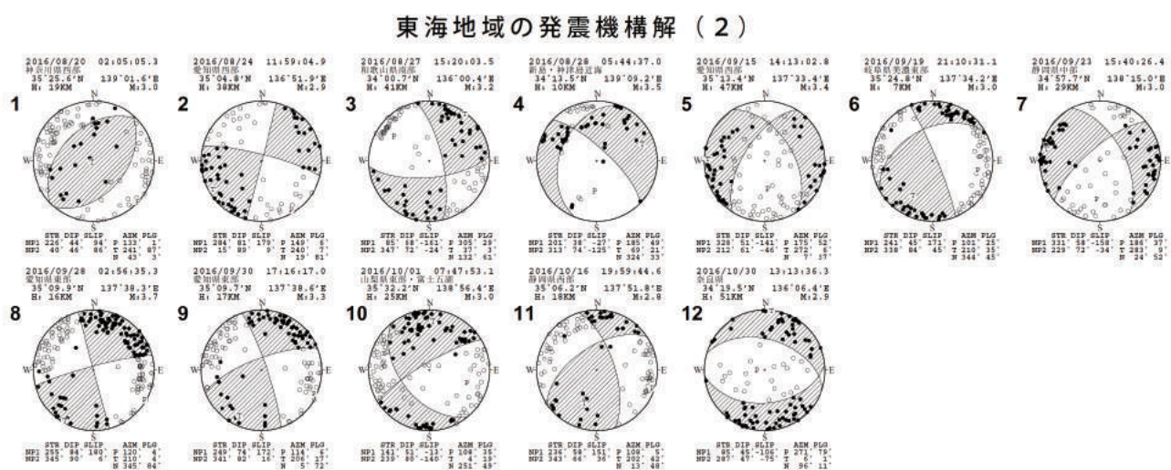
第2図(d) つづき (2016年8月～10月) Fig.2(d) Continued (August – October 2016).
