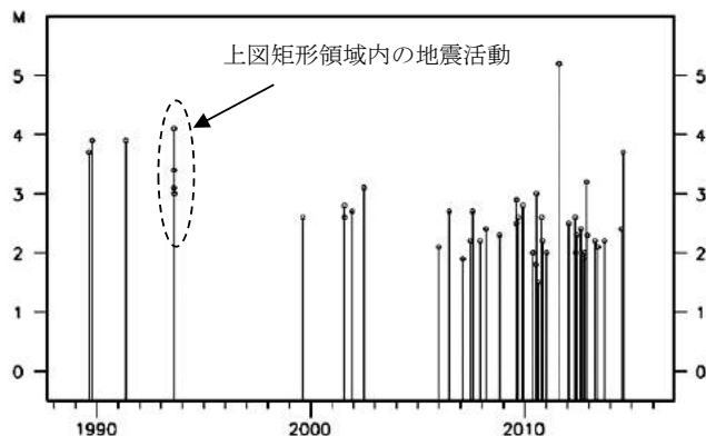
第17図 想定東海地震の発震機構解と類似の型の地震(第366回地震防災対策強化地域判定会気象庁資料 11) より抜粋)
