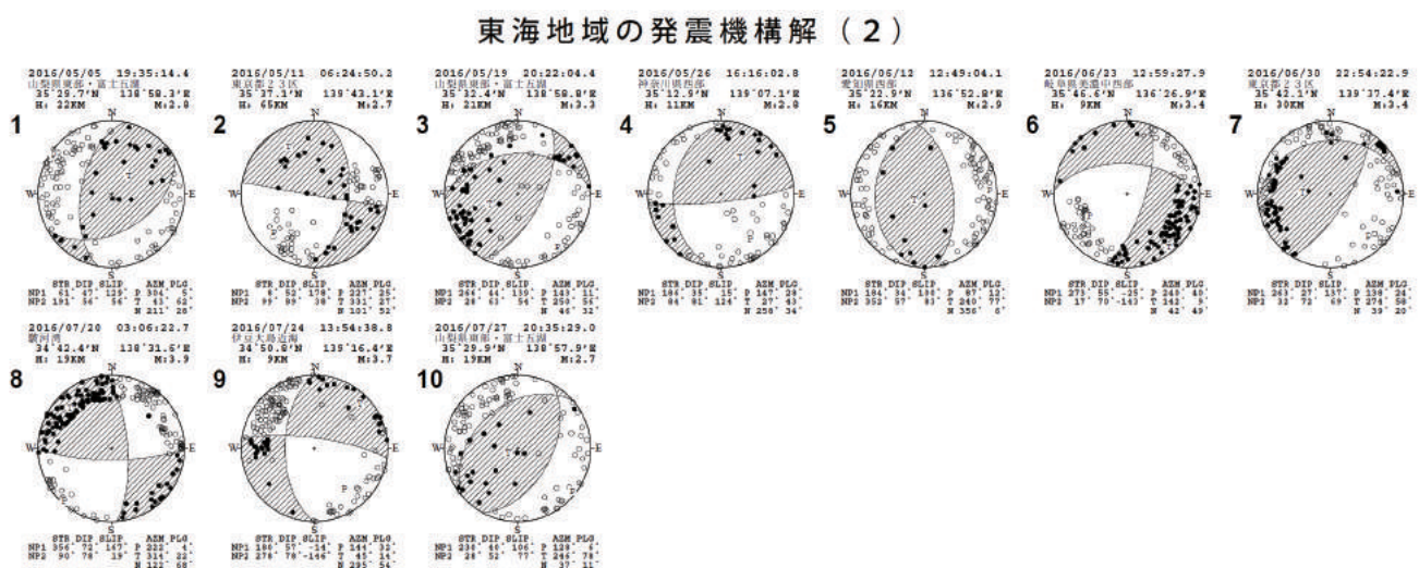
第2図(b) つづき (2016年5月～7月)
