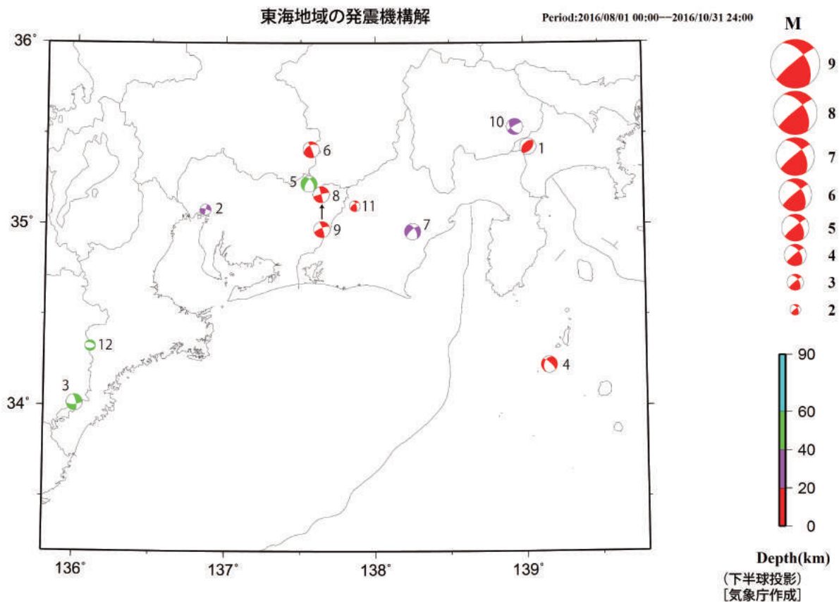
第2図(c) つづき (2016年8月～10月) Fig.2(c) Continued (August – October 2016).
