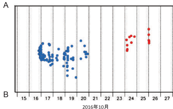
第4図(a) 愛知県の深部低周波地震活動とひずみ変化, 及び推定されるゆっくりすべり領域
