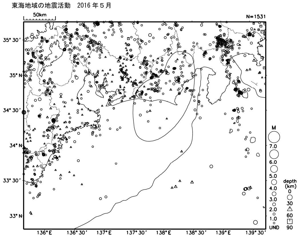
第1図(a) 東海地域で発生した地震の月別震央分布 (2016年5月)
