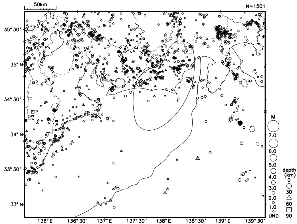
第1図(d) つづき (2016年8月)
