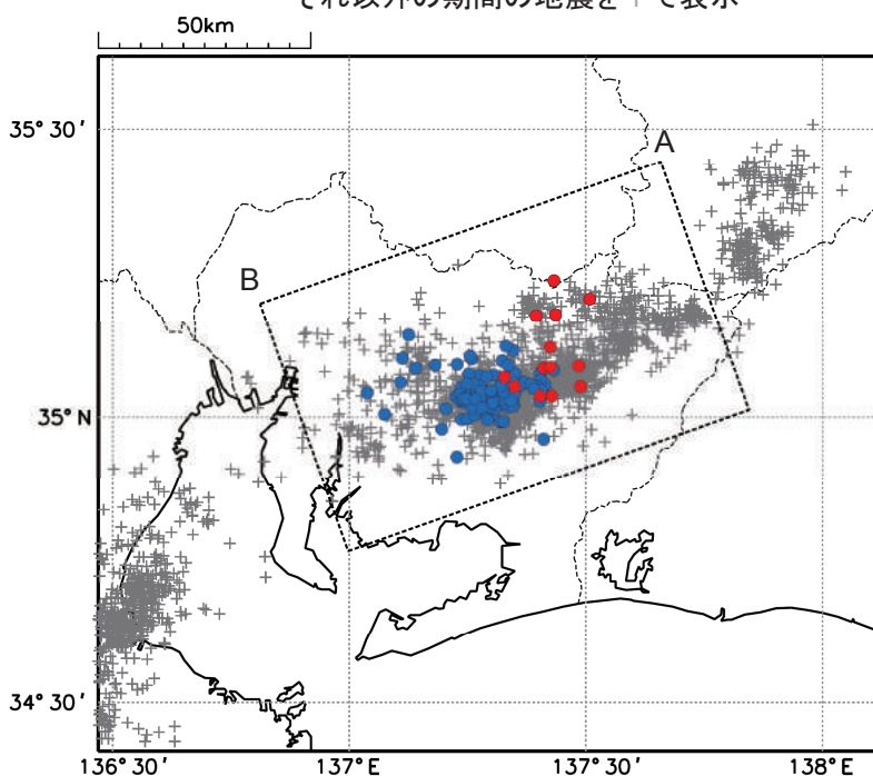
矩形領域内のAB方向の時空間分布図
