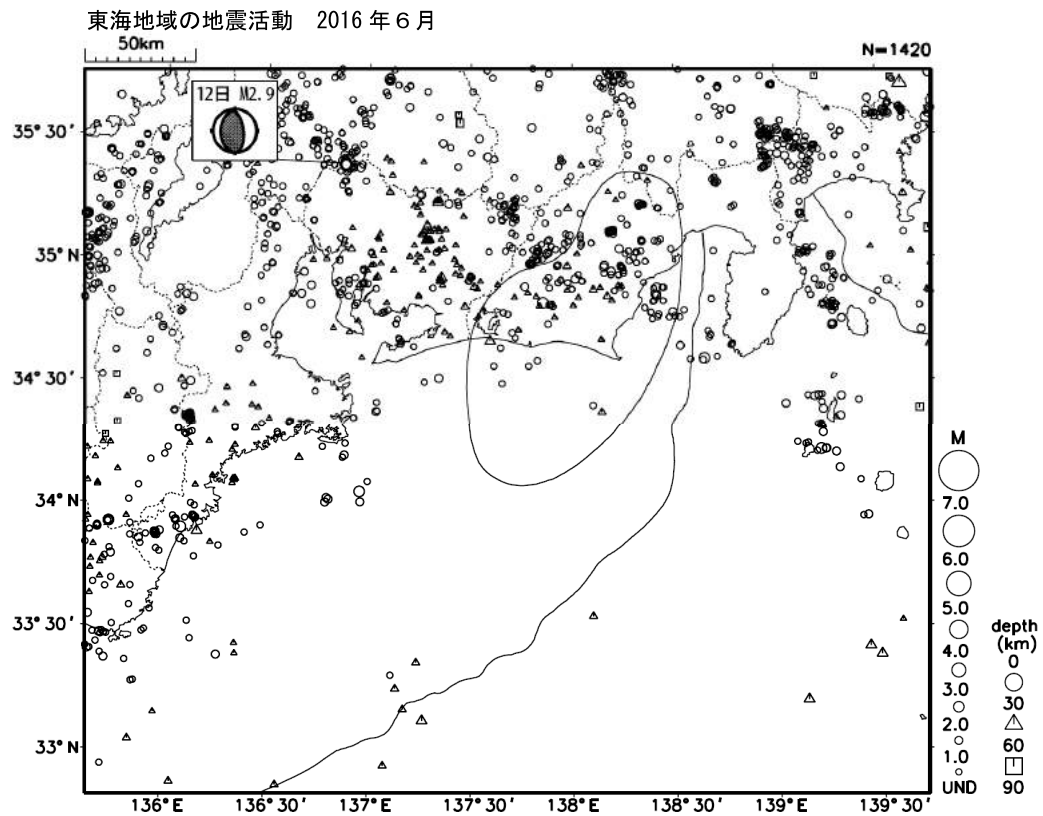
第1図(b) つづき (2016年6月)
