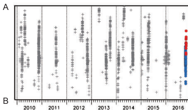
第4図(a) 愛知県の深部低周波地震活動とひずみ変化, 及び推定されるゆっくりすべり領域
