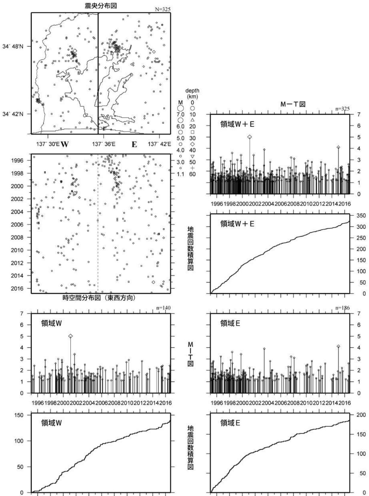
第12図 浜名湖付近のフィリピン海プレート内の地震活動（クラスタを除く、第366回地震防災対策強化地域判定会 気象庁資料 11) より抜粋）
