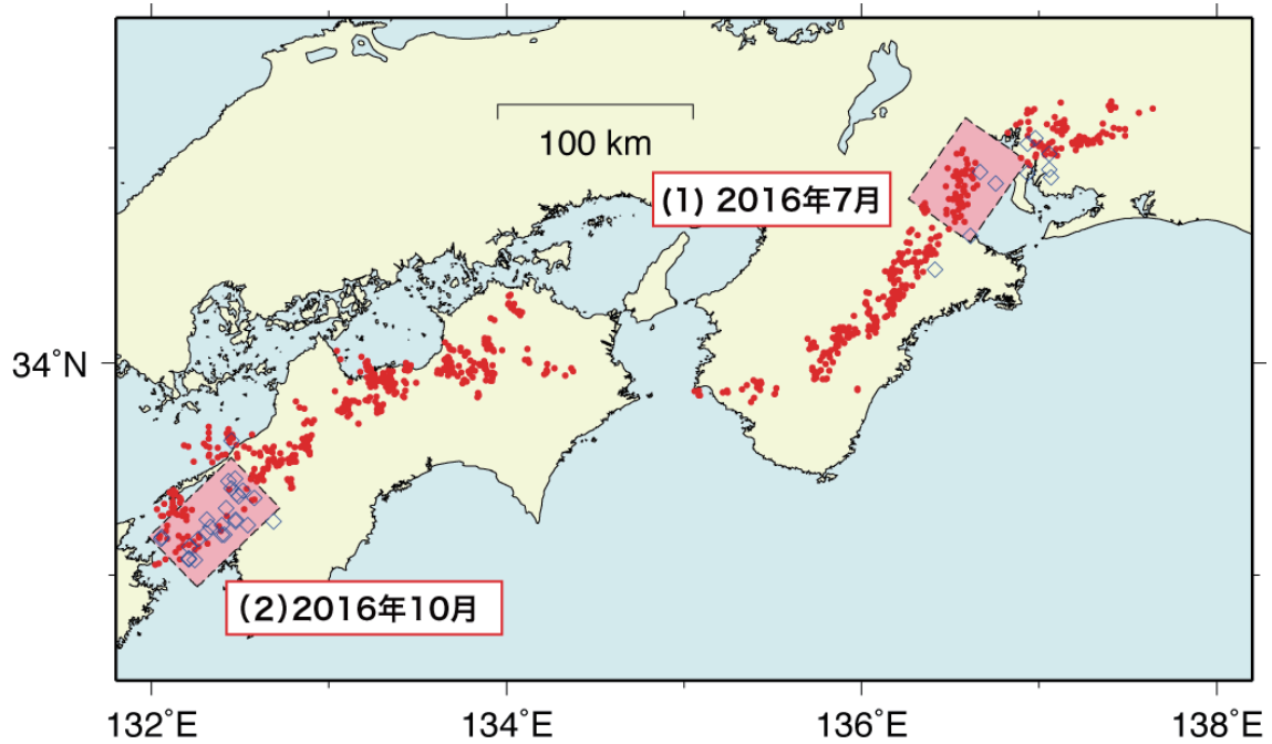
第1図 2016年5月～2016年10月の間に検知された短期的SSE(ピンク矩形). 同期間に発生した深部低周波微動(赤点)及びVLFEの震央(青菱形)を重ねて表示した.
