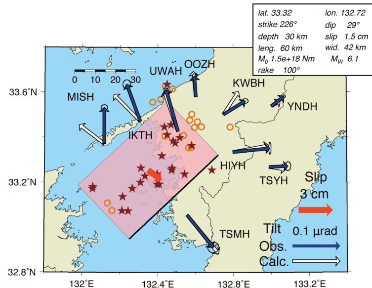
第5図 2016年10月四国西部 SSE の断層モデル。図の見方は第3図と同じ。2016年10月24日から26日の傾斜変化に基づくモデルを示す。 Fig.5 Same as Fig. 3 but for the October 2016 short-term SSE in the western Shikoku.
