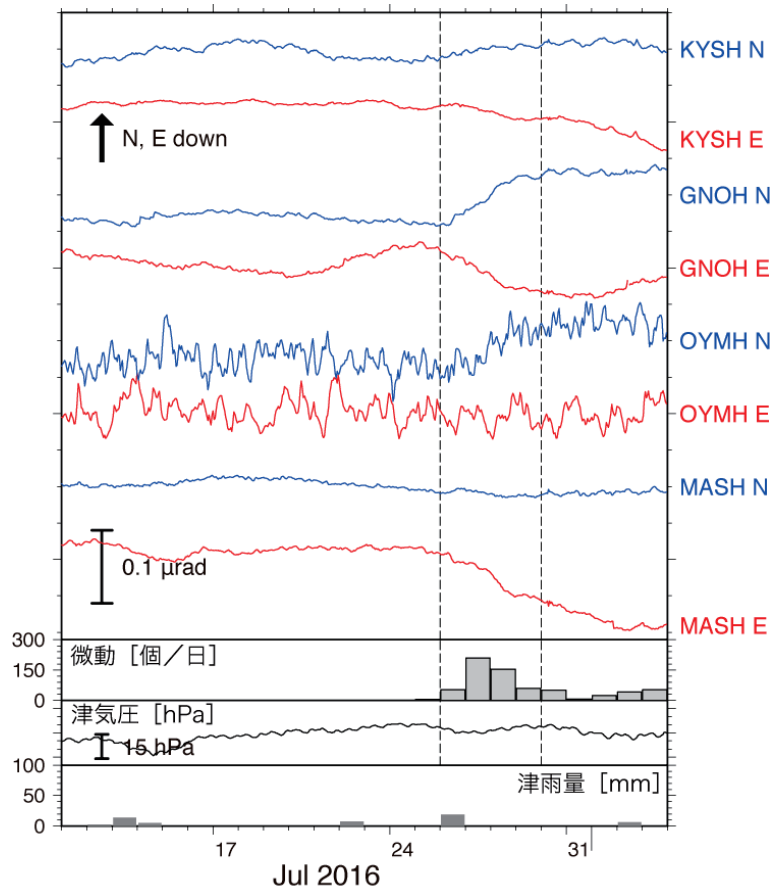
第2図 2016年7月11日から8月3日までの傾斜時系列。観測点位置は第3図に示した。記録は上方方向への変化が北・東下りの傾斜変動を表す。気圧応答・潮汐成分をBAYTAP-G 4) により除去し、直線トレンドを補正した後の記録を示した。7月26日～29日の傾斜変化量をSSEによるものと仮定した。紀伊半島北部での微動活動度・気象庁津観測点での気圧変化および雨量をあわせて表示した。
