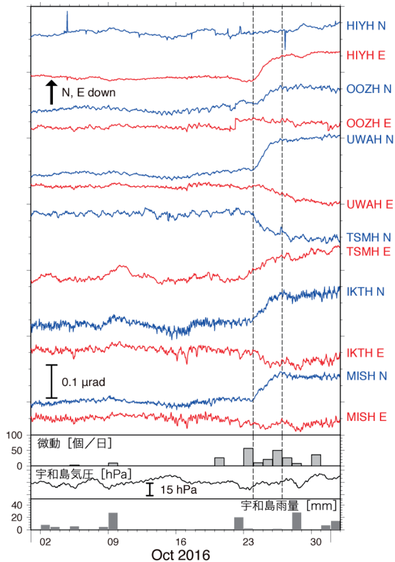
第4図 2016年10月1日から11月1日までの傾斜時系列。図の見方は第2図と同様。観測点位置は第5図に示した。四国西部における微動活動度・気象庁宇和島観測点での気圧変化および雨量をあわせて表示した。 Fig.4 Same as Fig. 2 but for the records observed around the western Shikoku from October 1, 2016 to November 1, 2016. The atmospheric pressure and the precipitation were observed at the JMA Uwajima meteorological observatory. The station locations and the tilt changes during the time window indicated by broken lines are shown in Fig. 5.
