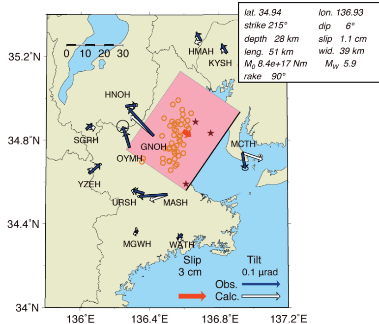
第3図 2016年7月紀伊半島北部短期的SSEの断層モデル。7月26日から29日に観測された傾斜変化ベクトル(青矢印)・このデータから推定されたSSEの断層モデル(赤矩形・矢印)・モデルから計算される傾斜変化ベクトル(白抜き矢印)を示す。同じ期間の微動および超低周波地震の震央を橙円と茶星印で示した。
