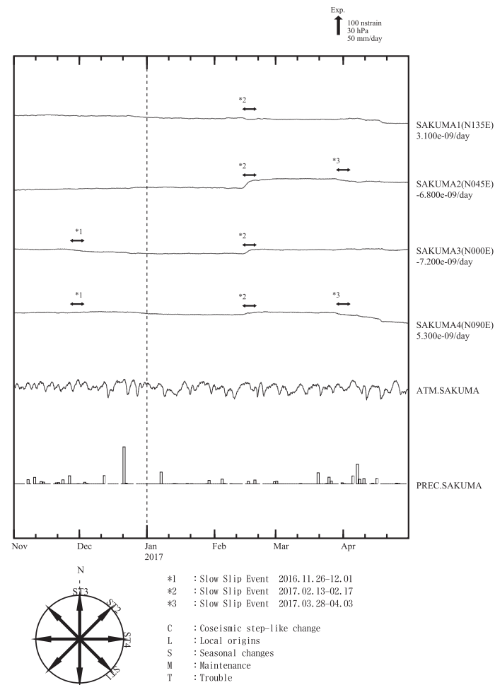
第4図(a)～(e) 左：2010年1月以後の多成分ひずみ計変化（日平均値）。主ひずみ・最大せん断ひずみ・面積ひずみは各方向成分から計算されている。 右：2016年11月～2017年4月の多成分ひずみ計変化（時間値：気圧・潮汐・地磁気・降水補正した値）。各図下部に気圧変化と降水量を示す。 Fig.4(a) – (e) (Left) Strain changes observed by multi-component borehole strainmeters since January 2010 (daily mean values). Principal strain, maximum shear strain and dilatation are calculated with strain values obtained from each component. (Right) Strain changes from November 2016 to April 2017 (hourly values where changes due to barometric pressure, tidal effects, geomagnetic effects and rain effects are corrected) observed by multi-component borehole strainmeters.
