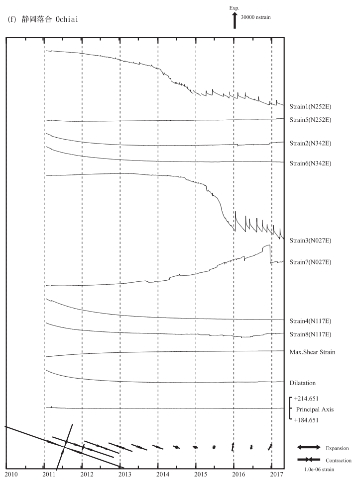
第4図(f)～(k) 左：2010年1月以後の多成分ひずみ計変化（日平均値）。主ひずみ・最大せん断ひずみ・面積ひずみは各方向成分から計算されている。 右：2016年11月～2017年4月の多成分ひずみ計変化（時間値：気圧・潮汐・地磁気補正した値）。各図下部に気圧変化と降水量を示す。
