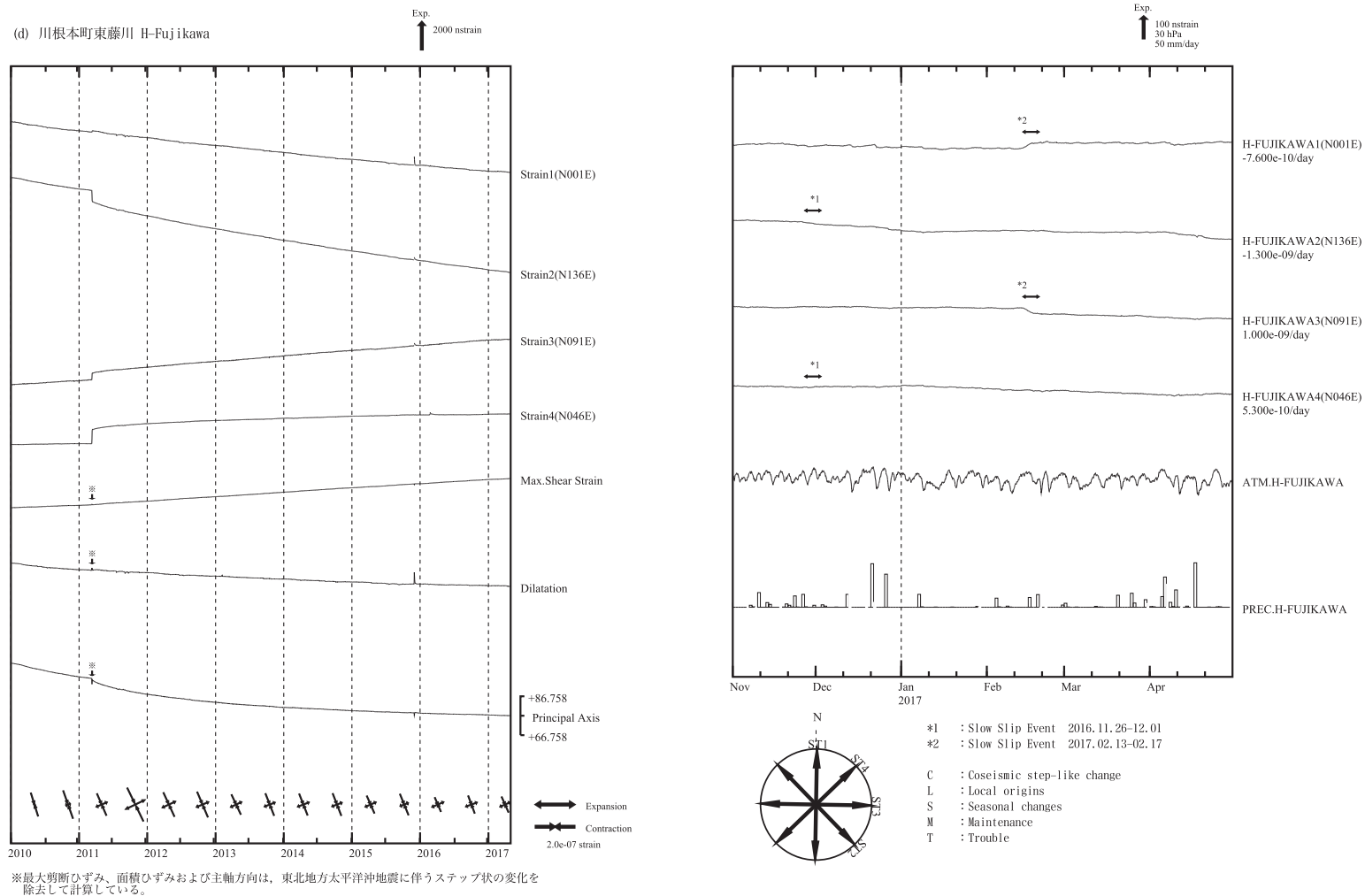
第 4 図 (a) ~ (c) 左：2010 年 1 月以後の多成分ひずみ計変化（日平均値）。主ひずみ・最大せん断ひずみ・面積ひずみは各方向成分から計算されている。 右：2016 年 11 月～2017 年 4 月の多成分ひずみ計変化（時間値：気圧・潮汐・地磁気・降水補正した値）。各図下部に気圧変化と降水量を示す。
