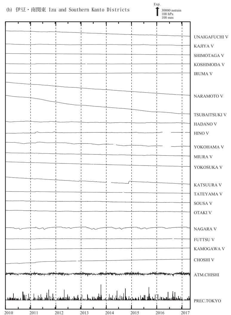
第2図(a), (b) 2010年1月以後の東海・伊豆・南関東地域における区域別体積ひずみ(V)及び面積ひずみ(S)の変化(日平均値). 各図下部に区域を代表する気圧変化と降水量を示す.
