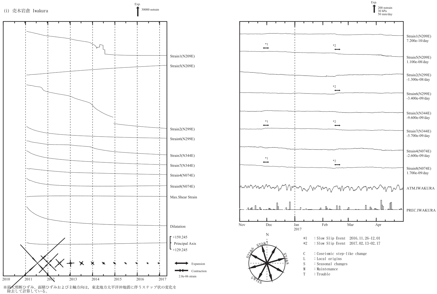
第4図 (f) ~ (k) 左：2010年1月以後の多成分ひずみ計変化（日平均値）。主ひずみ・最大せん断ひずみ・面積ひずみは各方向成分から計算されている。 右：2016年11月～2017年4月の多成分ひずみ計変化（時間値：気圧・潮汐・地磁気補正した値）。各図下部に気圧変化と降水量を示す。
