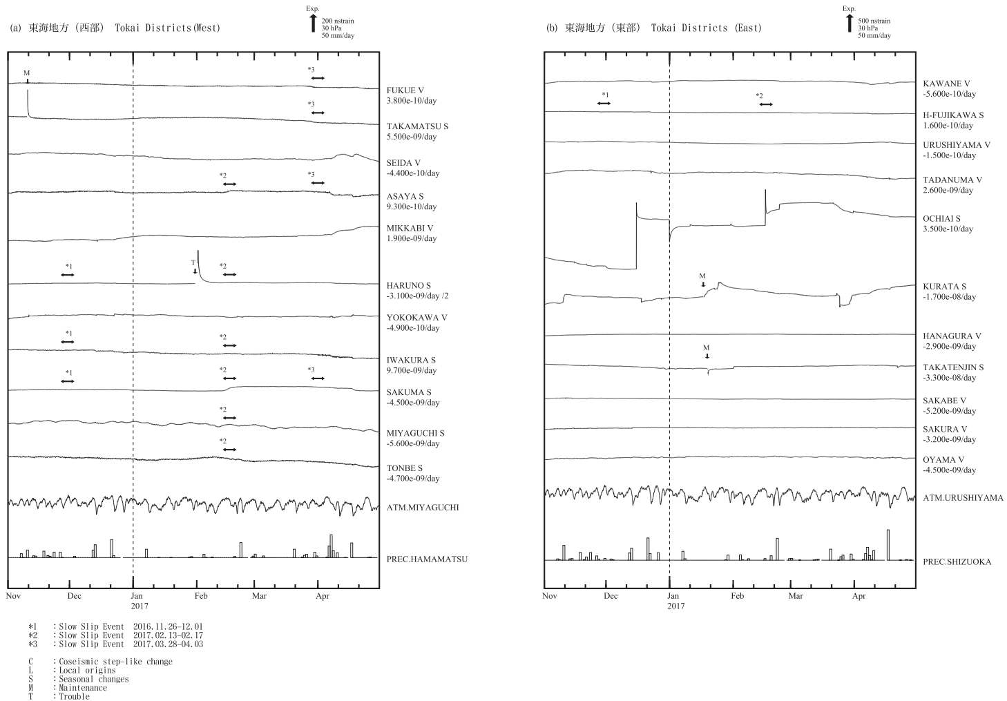
第 3 図 (a) ~ (d) 2016 年 11 月 ~ 2017 年 4 月の東海・伊豆・南関東地域における区域別体積ひずみ (V) 及び面積ひずみ (S) の変化 (時間値: 気圧・潮汐・降水補正した値). 各図下部に区域を代表する気圧変化と降水量を示す. 地点名の下に D strain/day 及び /M はそれぞれ 1 日あたりのトレンド変化量を D として補正していること及び縮尺を 1/M 倍にして表示していることを示している.
