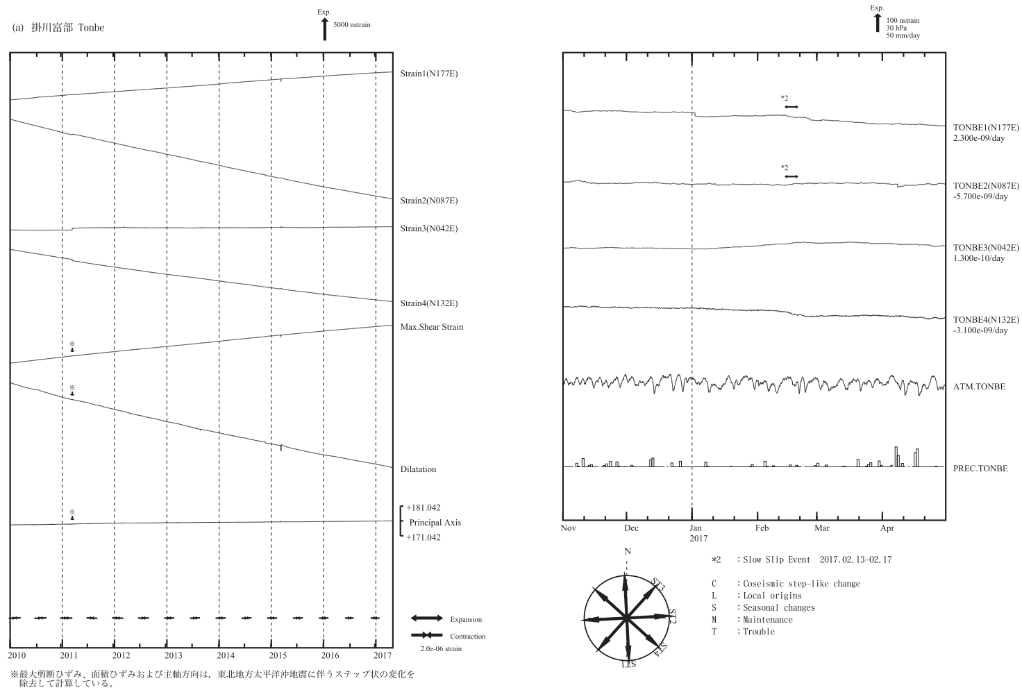
第 4 図 (a) ~ (e) 左：2010 年 1 月以後の多成分ひずみ計変化（日平均値）。主ひずみ・最大せん断ひずみ・面積ひずみは各方向成分から計算されている。 右：2016 年 11 月～2017 年 4 月の多成分ひずみ計変化（時間値：気圧・潮汐・地磁気・降水補正した値）。各図下部に気圧変化と降水量を示す。 Fig.4(a) – (e) (Left) Strain changes observed by multi-component borehole strainmeters since January 2010 (daily mean values). Principal strain, maximum shear strain and dilatation are calculated with strain values obtained from each component. (Right) Strain changes from November 2016 to April 2017 (hourly values where changes due to barometric pressure, tidal effects, geomagnetic effects and rain effects are corrected) observed by multi-component borehole strainmeters.
