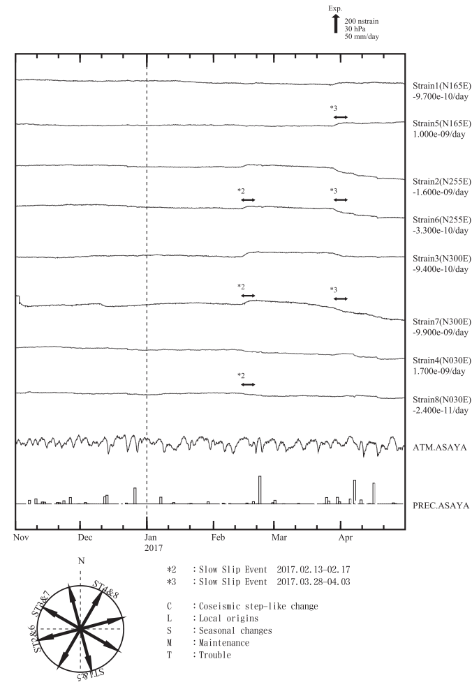
第4図(f)～(k) 左：2010年1月以後の多成分ひずみ計変化（日平均値）。主ひずみ・最大せん断ひずみ・面積ひずみは各方向成分から計算されている。 右：2016年11月～2017年4月の多成分ひずみ計変化（時間値：気圧・潮汐・地磁気補正した値）。各図下部に気圧変化と降水量を示す。
