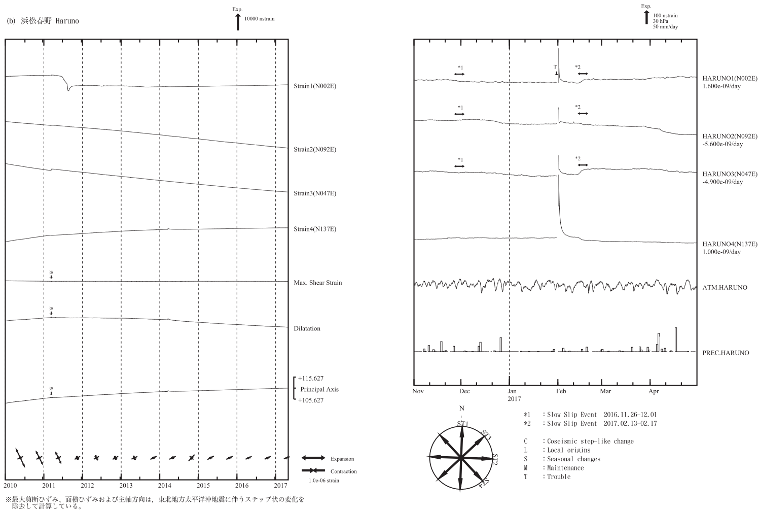
第4図(a)～(e) 左：2010年1月以後の多成分ひずみ計変化（日平均値）。主ひずみ・最大せん断ひずみ・面積ひずみは各方向成分から計算されている。 右：2016年11月～2017年4月の多成分ひずみ計変化（時間値：気圧・潮汐・地磁気・降水補正した値）。各図下部に気圧変化と降水量を示す。 Fig.4(a)–(e) (Left) Strain changes observed by multi-component borehole strainmeters since January 2010 (daily mean values). Principal strain, maximum shear strain and dilatation are calculated with strain values obtained from each component. (Right) Strain changes from November 2016 to April 2017 (hourly values where changes due to barometric pressure, tidal effects, geomagnetic effects and rain effects are corrected) observed by multi-component borehole strainmeters.
