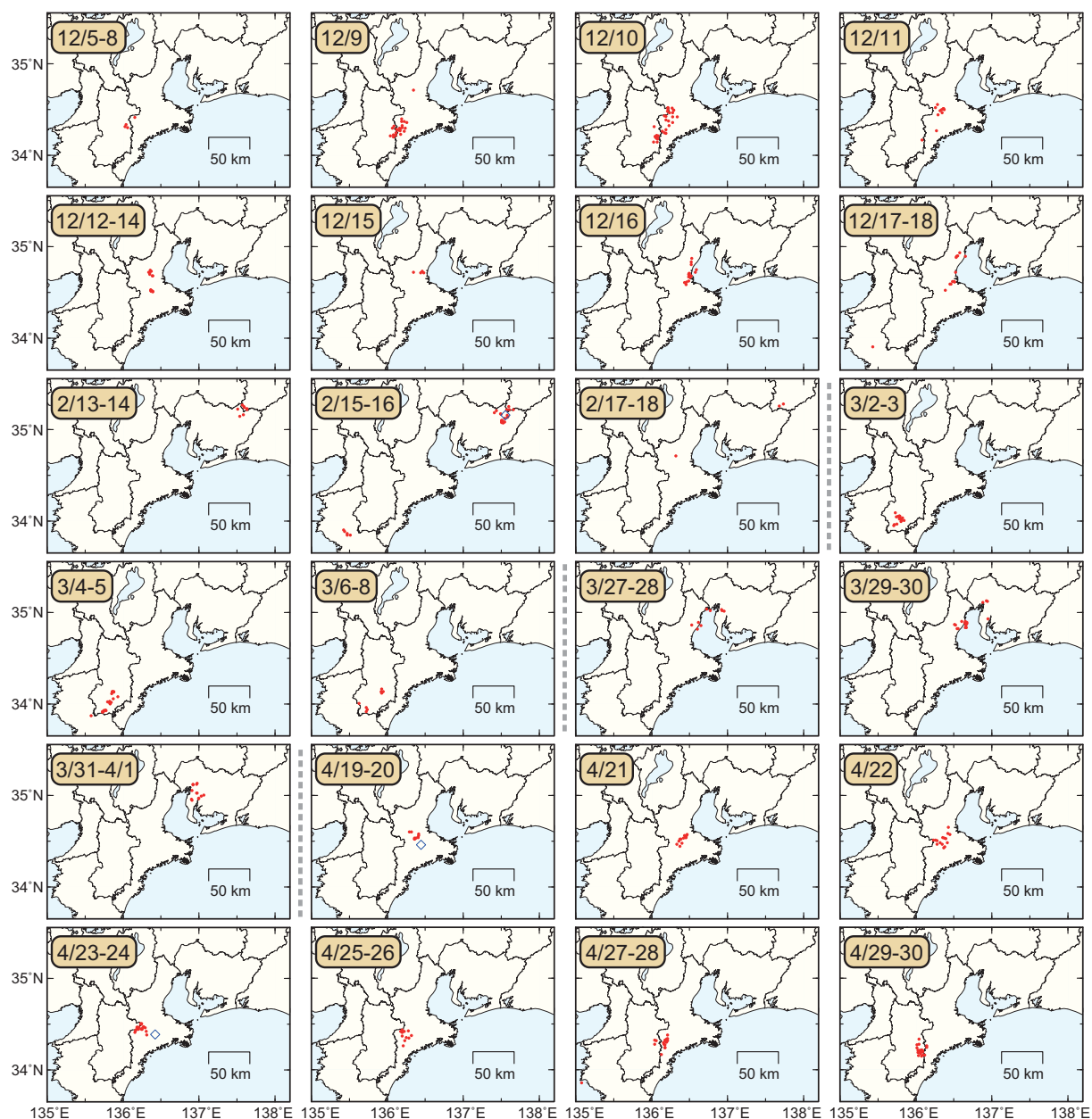
第4図 2016年11月から2017年4月までの期間に東海・紀伊半島地域で発生した、主な深部低周波微動及び深部超低周波地震の活動における震央分布スナップショット。赤丸が当該期間の微動、青菱形が超低周波地震を表す。
