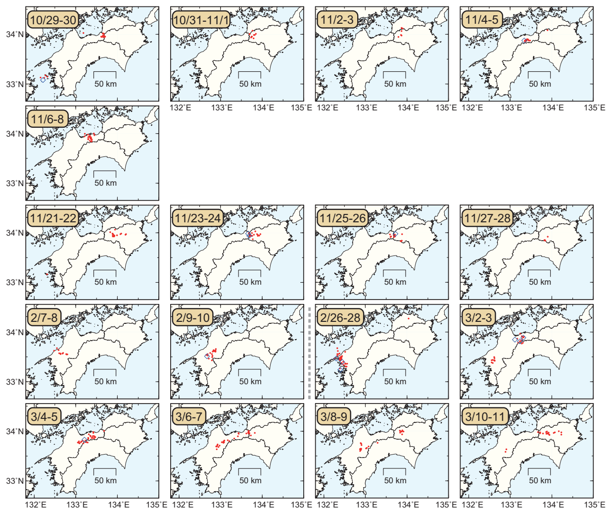
第5図 2016年11月から2017年4月までの期間に四国地域で発生した、主な深部低周波微動及び超低周波地震の活動における震央分布スナップショット。赤丸が当該期間の微動、青菱形が超低周波地震を表す。
