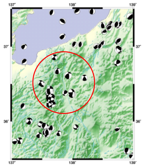
第2図 発震機構解（防災科技研による）
