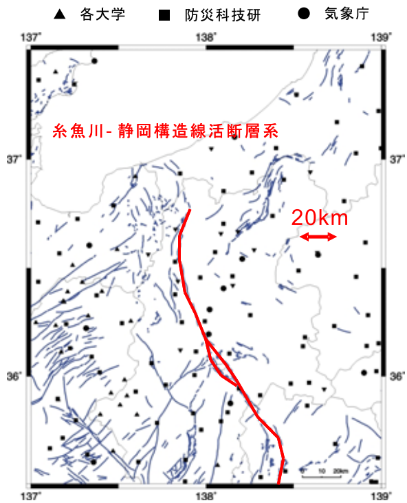
第1図 観測点配置
