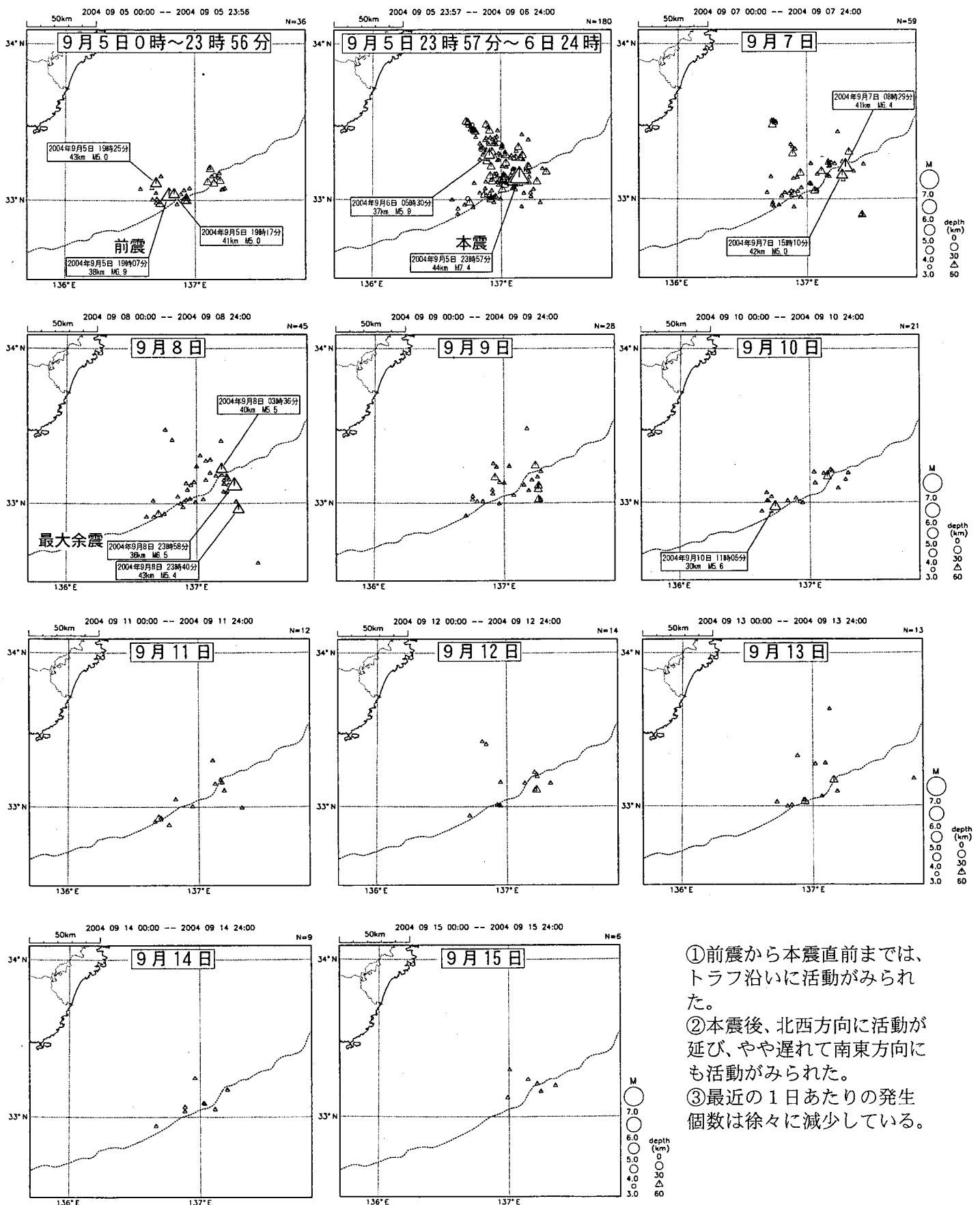
震央分布図 (M \geq 3.0)
