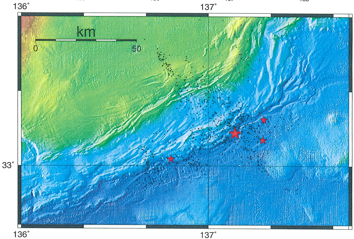
紀伊半島沖の海底地形の陰影図. 黒丸は気象庁一元化震源 (2004年9月5日19時時より7日間) 大きな赤星印は本震, 小さな赤星は M \geq 6.0 以上の震央の位置.
